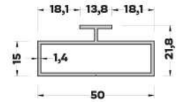
MB-4971 (0,548 kg/mt) ORTA KAYIT PROFİLİ
