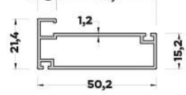
MB-5597 (0,511 kg/mt) ÇERÇEVE KAPAK PROFİLİ
