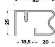
MB-3147 (0,530 kg/mt) BOY KULP PROFİLİ
