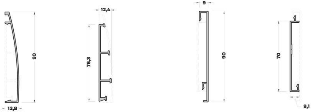
SP-4212 (0,433 kg/mt.) SÜPÜRGELİK PROFİLİ
