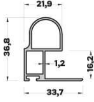
MB-5544 (0,470 kg/mt) BOY KULP PROFİLİ
