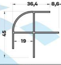
MB-4870 (0,488 kg/mt) BAZA DÖNÜŞ PROFİLİ
