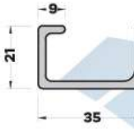
MB-5678 (0,590 kg/mt) KULP PROFİLİ
