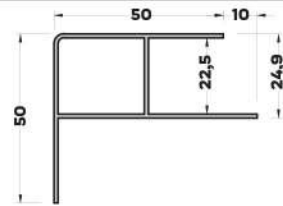
MB-5272 (0,582 kg/mt) BAZA KAPAMA PROFİLİ
