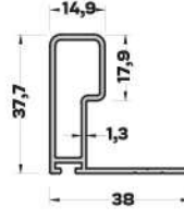
MB-5348 (0,478 kg/mt) BOY KULP PROFİLİ
