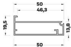
MB-7366 (0,430 kg/mt) ÇERÇEVE KAPAK PROFİLİ
