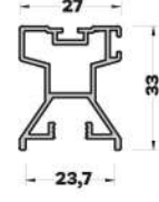
MB-7687 (0,498 kg/mt) YAN KULP PROFİLİ
