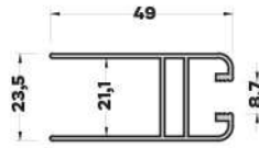
MB-4749 (0,402 kg/mt) ORTA BAĞLANTI PROFİLİ
