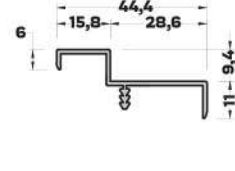
MB-5871 (0,256 kg/mt) ÇITA PROFİLİ
