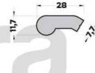
MB-4822 (0,617 kg/mt) KULP PROFİLİ
