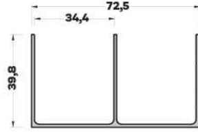
MB-5217 (0,685 kg/mt) ÜST RAY PROFİLİ
