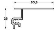
DL-1941 (0,460 kg/mt.) DİLATASYON PROFİLİ
