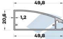
MB-5029 (0,455 kg/mt) ÇERÇEVE KAPAK PROFİLİ
