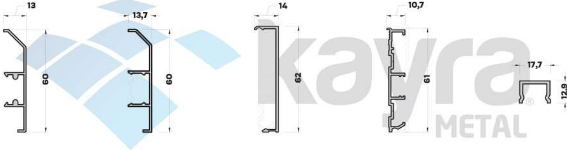
SP-4628 (0,317 kg/mt) SÜPÜRGELİK PROFİLİ
