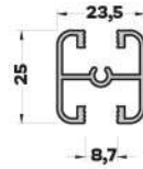
MB-4749 (0,402 kg/mt) ORTA BAĞLANTI PROFİLİ
