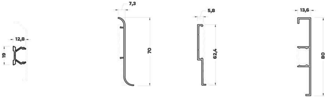
SP-3068 (0,128 kg/mt) SÜPÜRGELİK ALT PROFİLİ
