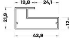
MB-5882 (0,458 kg/mt) ÇERÇEVE KAPAK PROFİLİ
