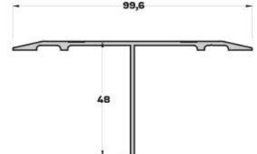
DL-8047 (0,707 kg/mt.) DİLATASYON PROFİLİ
