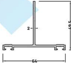
SRMKA-02 ÖZEL SERAMİK FİTİLİ
