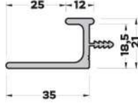
MB-5679 (0,485 kg/mt) KULP PROFİLİ
