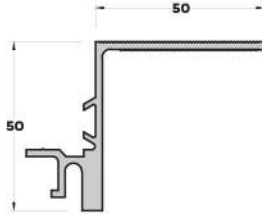
DL-2780 (0,969 kg/mt.) DİLATASYON PROFİLİ
