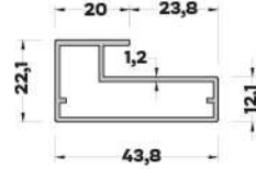
MB-5883 (0,460 kg/mt) ÇERÇEVE KAPAK PROFİLİ
