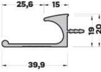
MB-5196 (0,534 kg/mt) KULP PROFİLİ
