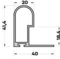
MB-5036 (0,583 kg/mt) BOY KULP PROFİLİ
