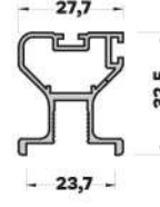
MB-4751 (0,500 kg/mt) YAN KULP PROFİLİ
