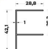
MB-6671 (0,263 kg/mt) BAZA KAPAMA PROFİLİ
