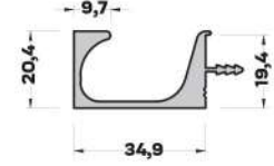
MB-5042 (0,652 kg/mt) KULP PROFİLİ
