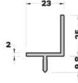
MB-5443 (0,306 kg/mt) ÇITA PROFİLİ
