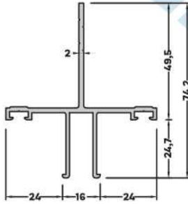
510-1101 (0,866 kg/mt.) COTTA PROFİL CM01
