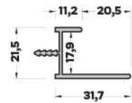
MB-5041 (0,314 kg/mt) KULP PROFİLİ
