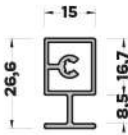
MB-5049 (0,295 kg/mt) ÜST BAĞLANTI PROFİLİ
