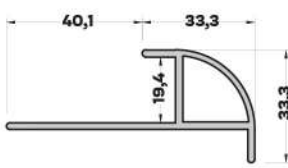
MB-4728 (0,788 kg/mt) BAZA KAPAMA PROFİLİ
