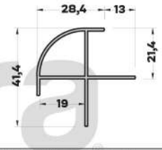
MB-5598 (0,410 kg/mt) BAZA DÖNÜŞ PROFİLİ
