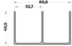
MB-4746 (0,732 kg/mt) ÜST RAY PROFİLİ
