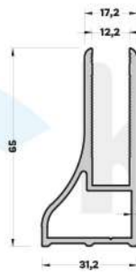
KHR40-1020 (1,063 kg/mt) 65° LİK YARIM CAM KANAL PROFİLİ
