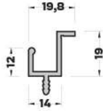
MB-5843 (0,295 kg/mt) ÇITA PROFİLİ
