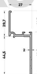
510-1104 (0,545 kg/mt.) COTTA KÖŞE DÖNÜŞ PR. CM04
