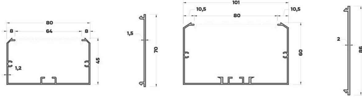
SP-3736 (0,744 kg/mt) KABLO KANALLI SÜPÜRGELİK PR.
