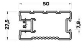
MB-5064 (0,446 kg/mt) ORTA BAĞLANTI PROFİLİ
