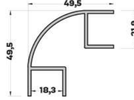
MB-5059 (0,745 kg/mt) BAZA DÖNÜŞ PROFİLİ
