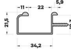
MB-5273 (0,410 kg/mt) KULP PROFİLİ
