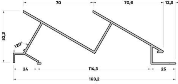
12175 (1,494 kg/mt.) İKİ YAPRAKLI MENFEZ PROFİLİ
