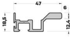
MB-8368 (0,670 kg/mt) YAN KULP PROFİLİ
