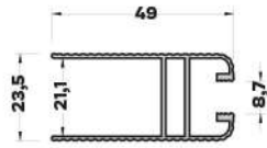
MB-4748 (0,320 kg/mt) ÜST BAĞLANTI PROFİLİ
