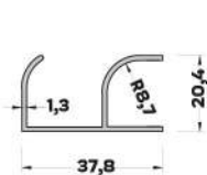
MB-5037 (0,305 kg/mt) BOY KULP PROFİLİ
