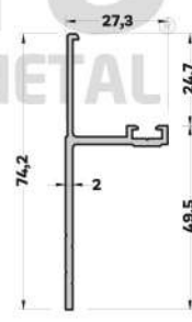
510-1105 (0,539 kg/mt.) COTTA BİTİŞ PROFİLİ CM05
