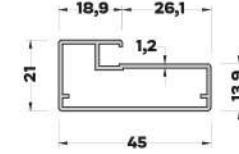
MB-4744 (0,450 kg/mt) ÇERÇEVE KAPAK PROFİLİ
