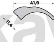
MB-4825 (0,667 kg/mt) KULP PROFİLİ
