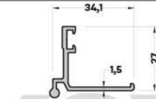
510-1103 (0,352 kg/mt.) COTTA KÖŞE DÖNÜŞ PR. CM03
