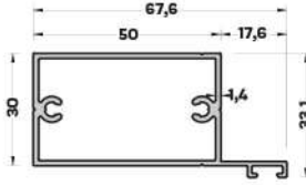
12175 (1,494 kg/mt.) İKİ YAPRAKLI MENFEZ PROFİLİ
