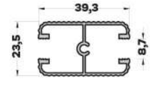
MB-5064 (0,446 kg/mt) ORTA BAĞLANTI PROFİLİ
