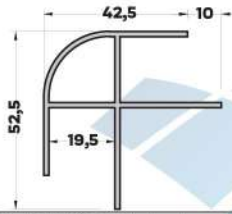
MB-4083 (0,715 kg/mt) BAZA DÖNÜŞ PROFİLİ
