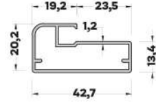
MB-5024 (0,446 kg/mt) ÇERÇEVE KAPAK PROFİLİ
