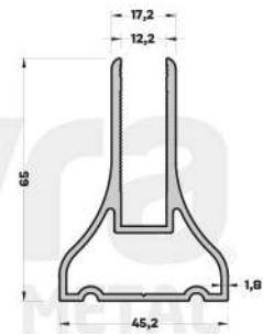
KHR40-1021 (1,212 kg/mt) 65° LİK CAM KANAL PROFİLİ
