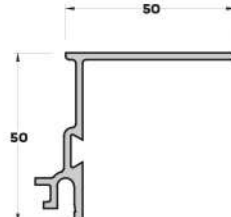
DL-2781 (0,708 kg/mt.) DİLATASYON PROFİLİ
