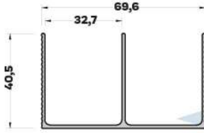
MB-7463 (0,564 kg/mt) ÜST RAY PROFİLİ
