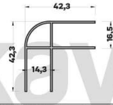
MB-5276 (0,472 kg/mt) BAZA DÖNÜŞ PROFİLİ
