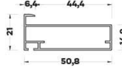
MB-5027 (0,415 kg/mt) ÇERÇEVE KAPAK PROFİLİ
