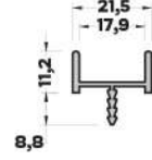
MB-5040 (0,214 kg/mt) KULP PROFİLİ
