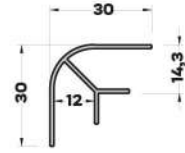
MB-7432 (0,265 kg/mt) BAZA DÖNÜŞ PROFİLİ
