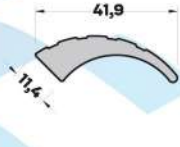
MB-4824 (0,643 kg/mt) KULP PROFİLİ
