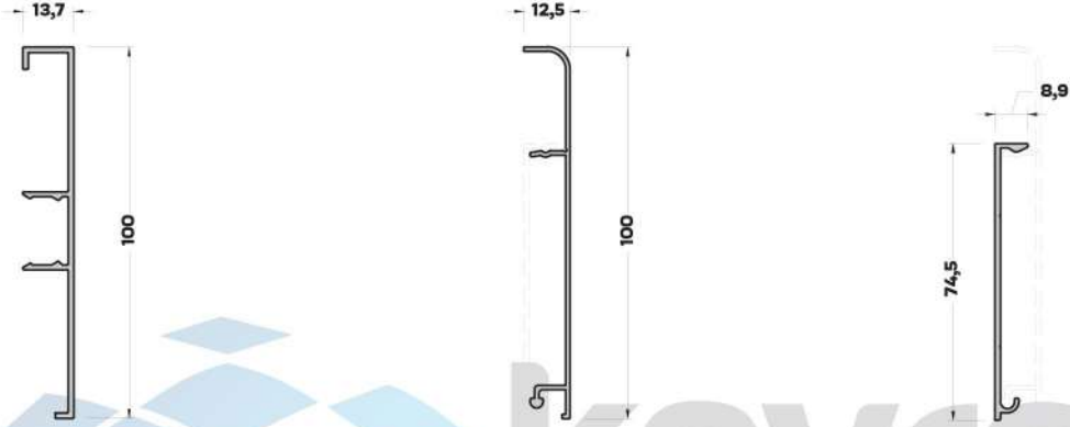
SP-4212 (0,433 kg/mt.) SÜPÜRGELİK PROFİLİ
