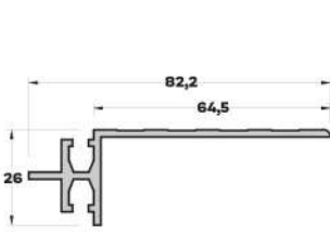
DL-3840 (0,700 kg/mt.) DİLATASYON PROFİLİ
