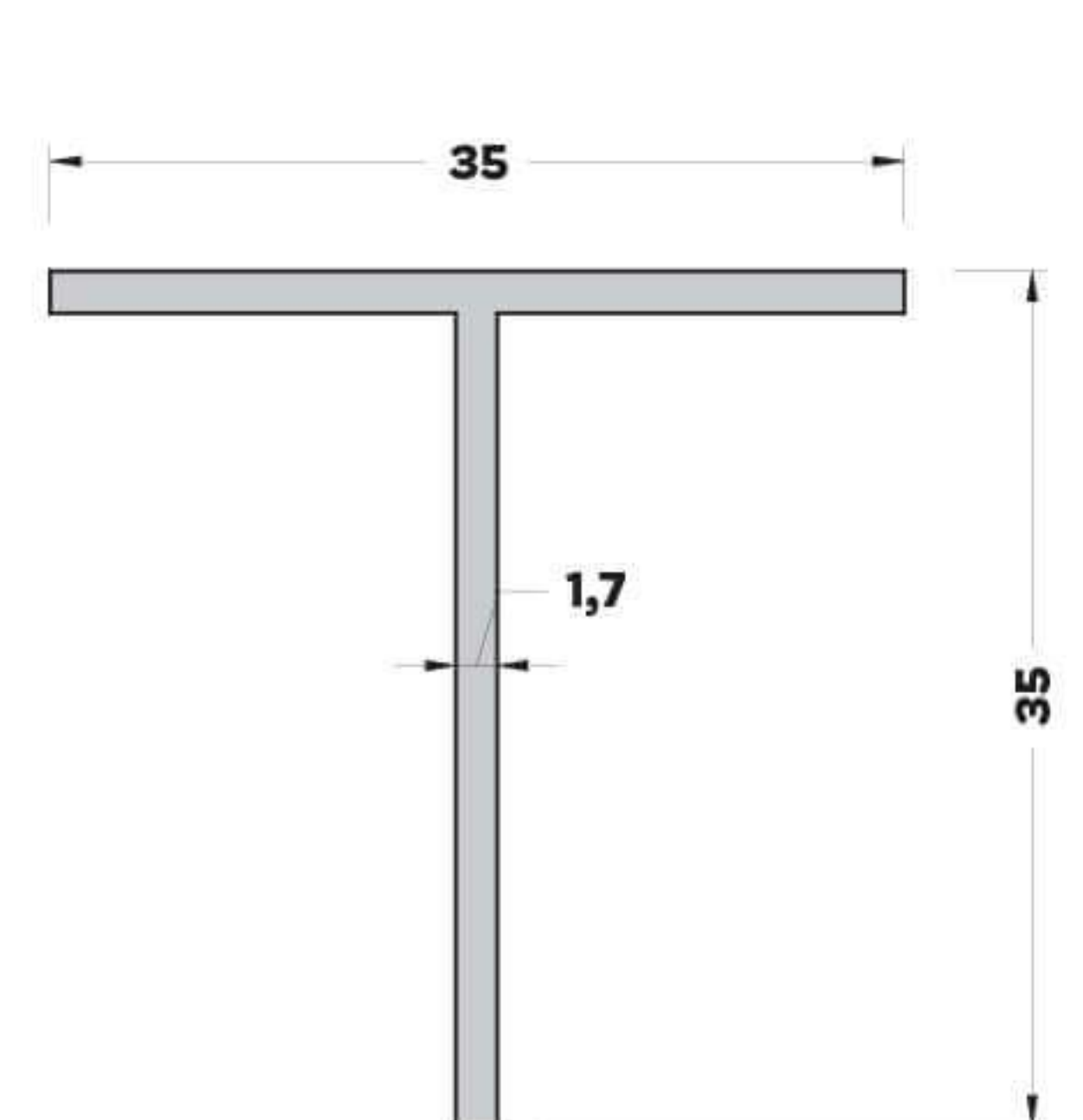
T-1318 (0,176 kg/mt) T BİNİ PROFİLİ
