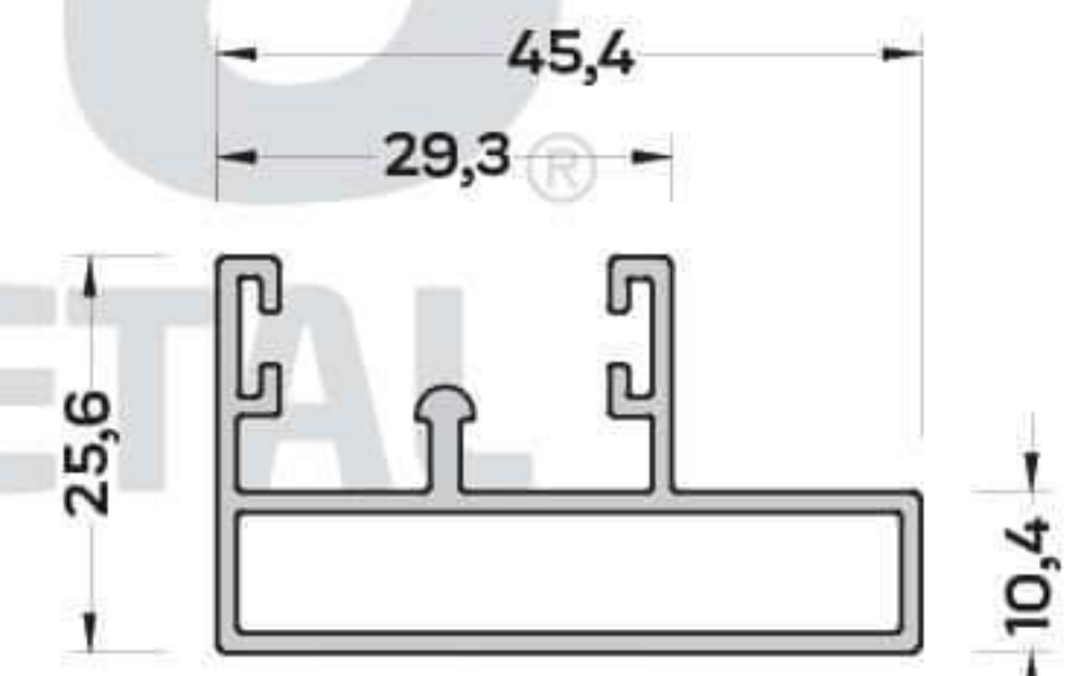
SN-1462 (0,391 kg/mt) SİNEKLİK RAY PROFİLİ
