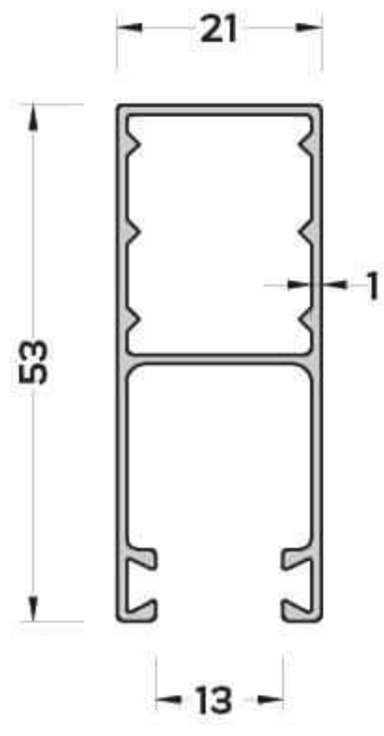
P-3948 (0,475 kg/mt) PANJUR YAN KASA PROFİLİ
