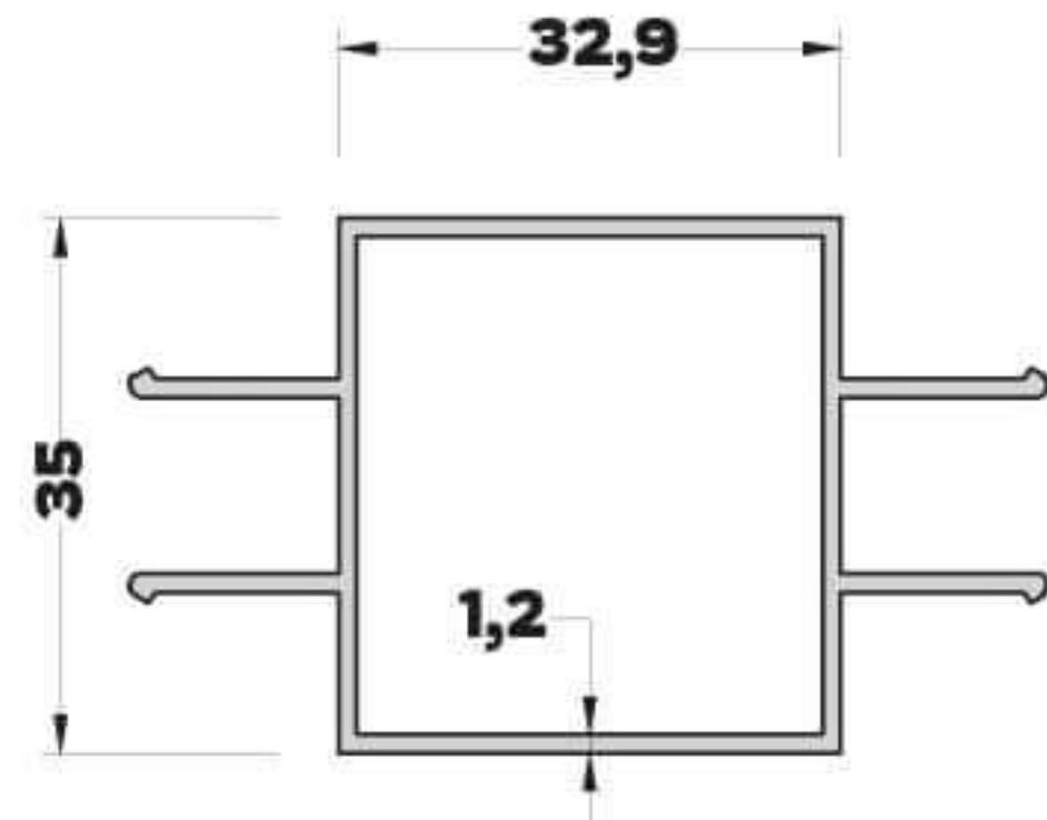
AB-1843 (0,756 kg/mt) TAŞIYICI GÖVDE PROFİLİ
