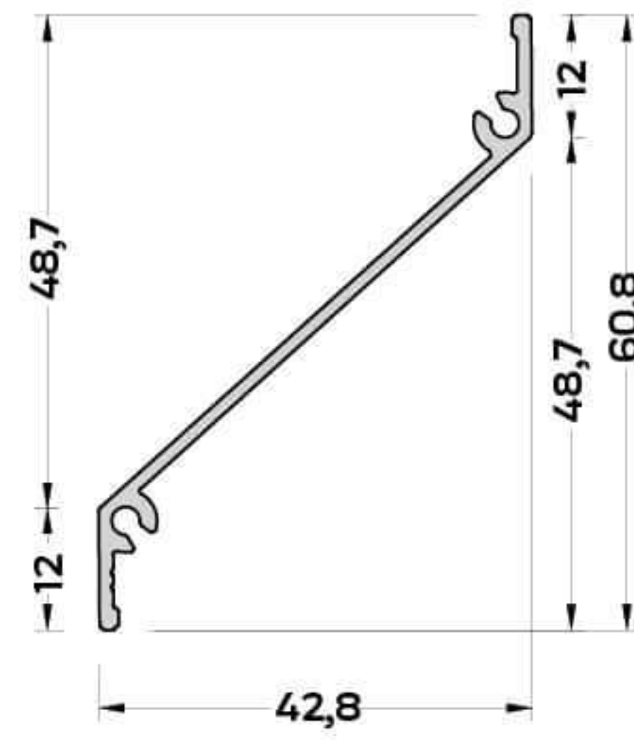
M-3076 (0,343 kg/mt) MENFEZ PROFİLİ
