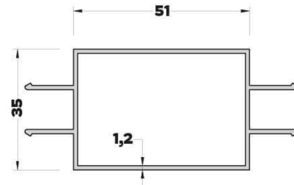
AB-6545 (0,912 kg/mt) KAPI KASA PROFİLİ
