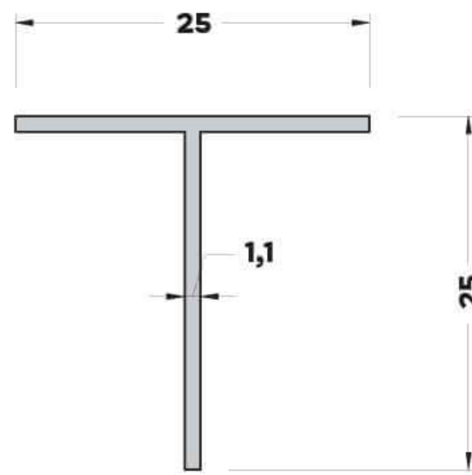
T-156 (0,146 kg/mt) T BİNİ PROFİLİ
