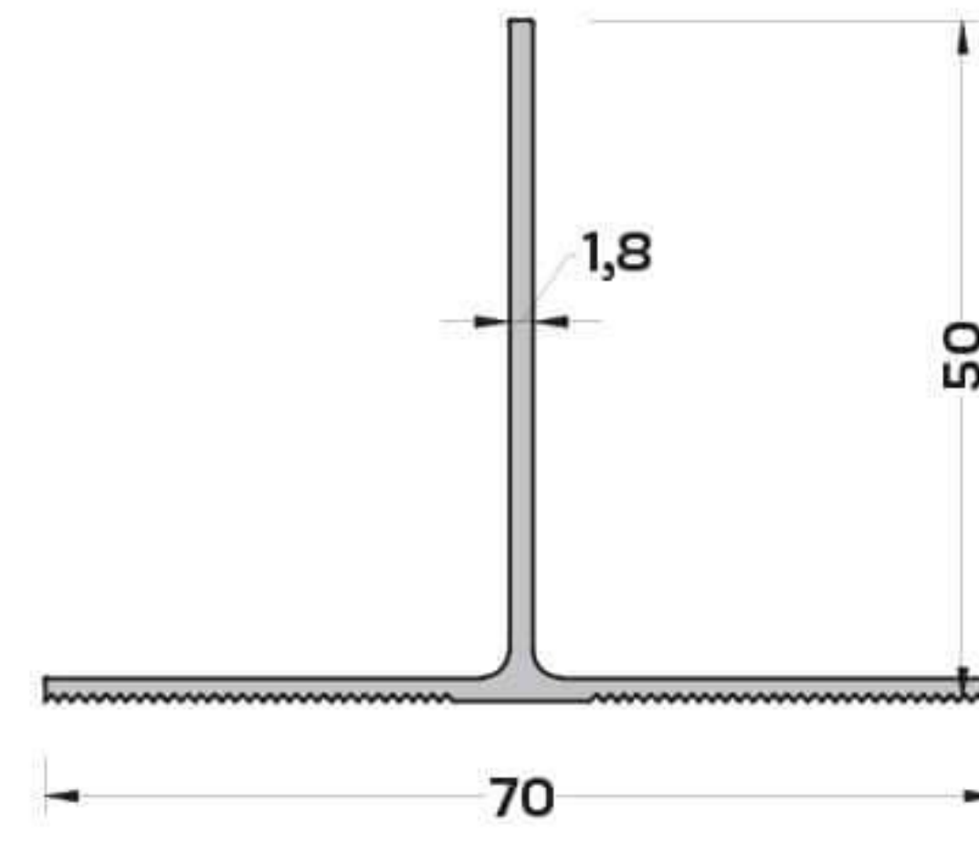
CK-6702 (0,528 kg/mt) T PROFİLİ
