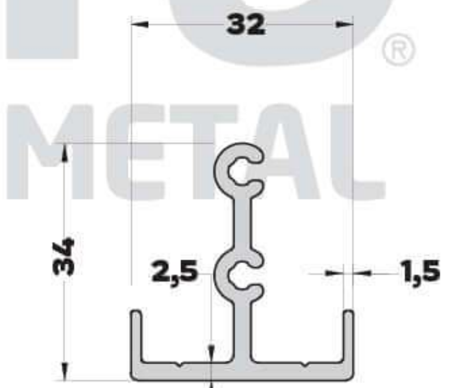
AB-6543 (0,944 kg/mt) PST SİSTEM KASA PROFİLİ
