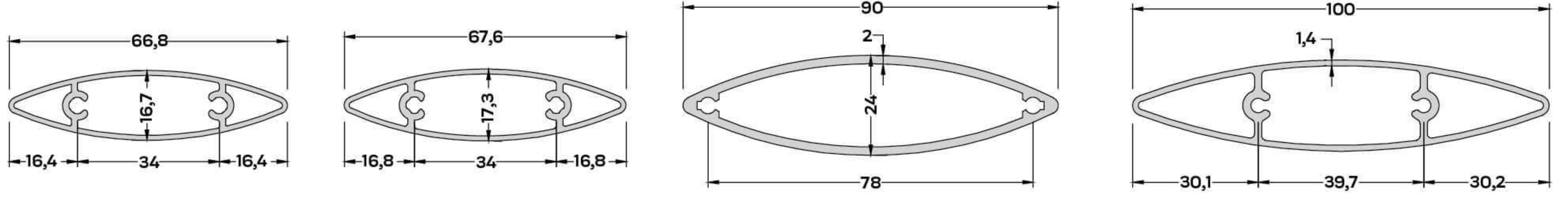
GK-10740 (0,594 kg/mt) GÜNEŞ KIRICI PR. 66,8 mm
