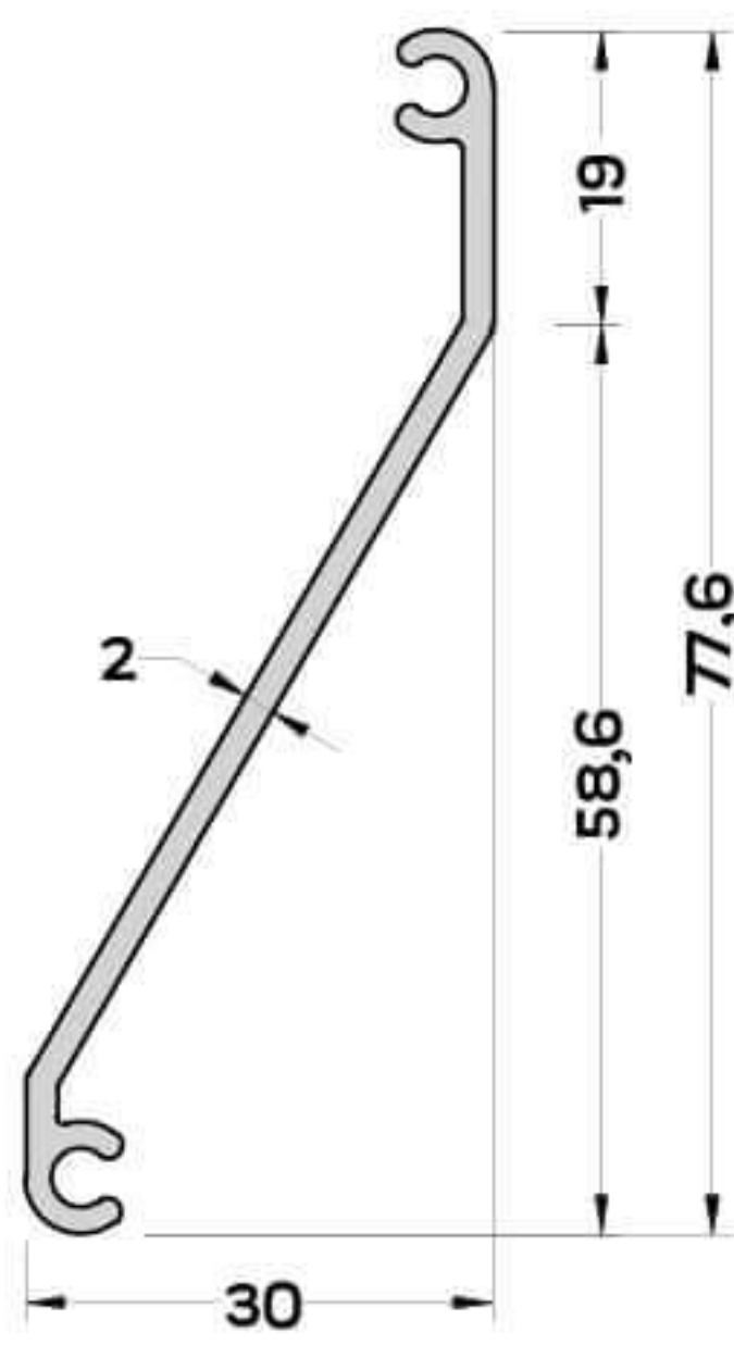
M-2815 (0,521 kg/mt) MENFEZ PROFİLİ
