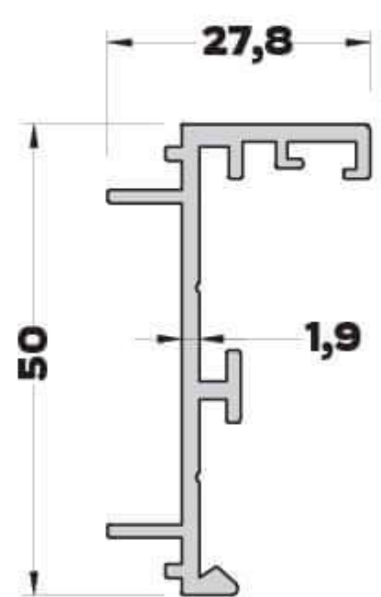
AB-6541 (0,556 kg/mt) ADAPTÖR PROFİLİ
