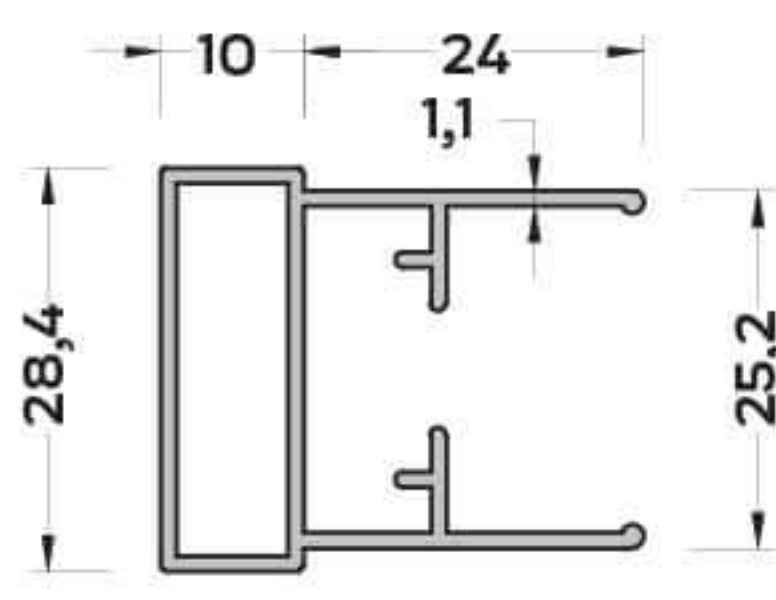
SN-4330 (0,528 kg/mt) SİNEKLİK DİKME PROFİLİ
