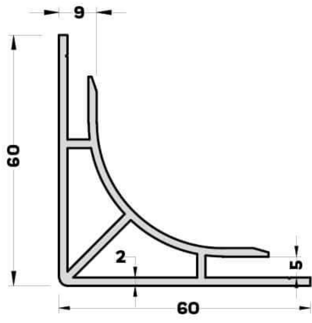
KM-6923 / 1,175 kg/mt KÖŞE DÖNÜŞ PROFİLİ
