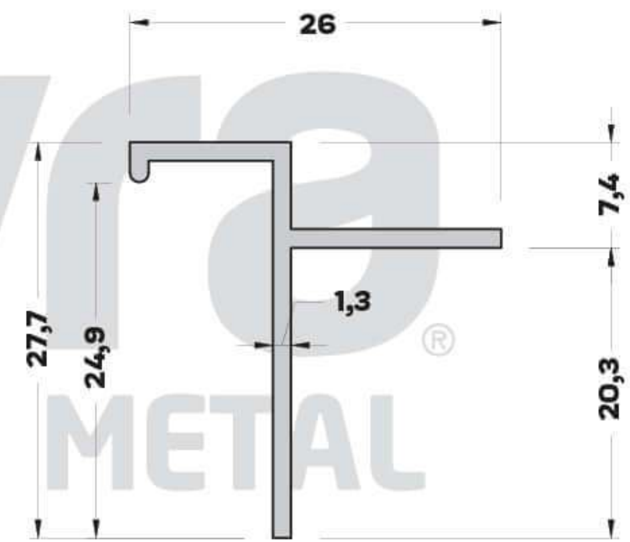
T-1512 (0,180 kg/mt.) ASİMETRİK T BİNİ PROFİLİ
