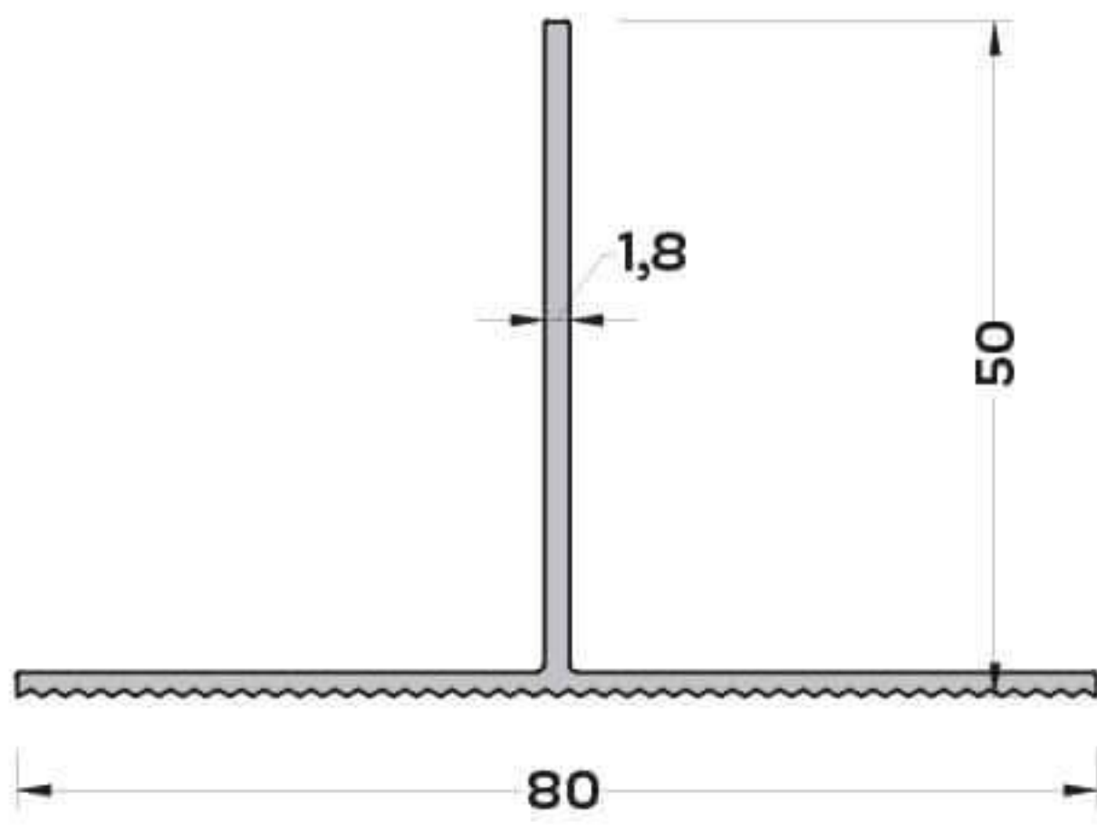
CK-6312 (0,531 kg/mt) T PROFİLİ
