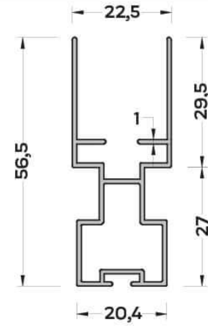
SN-6232 (0,499 kg/mt) SİNEKLİK KANAT PROFİLİ
