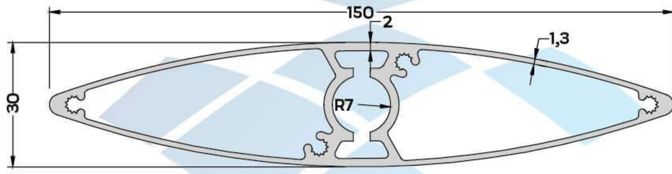
S-8288 (1,486 kg/mt) GÜNEŞ KIRICI PR. 150 mm
