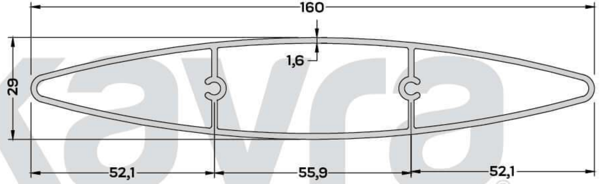
S-6074 (1,675 kg/mt) GÜNEŞ KIRICI PR. 160 mm
