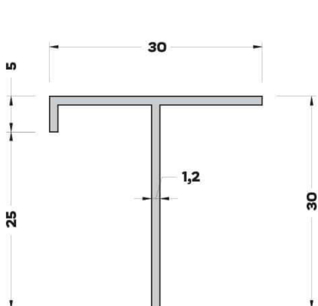
T-6341 (0,176 kg/mt) T BİNİ PROFİLİ
