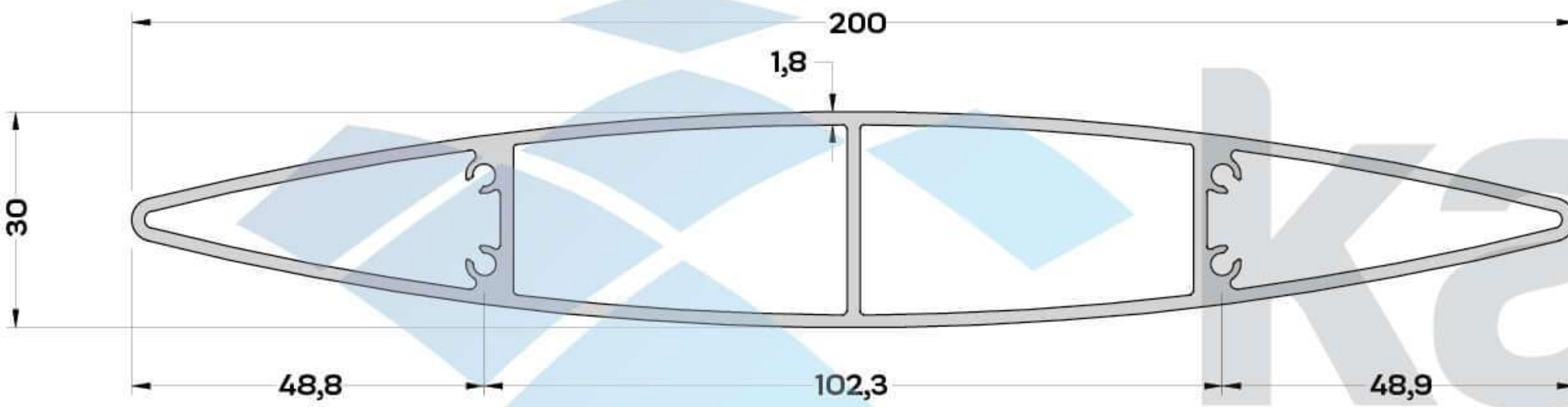
S-1179 (2,208 kg/mt) GÜNEŞ KIRICI PR. 200 mm
