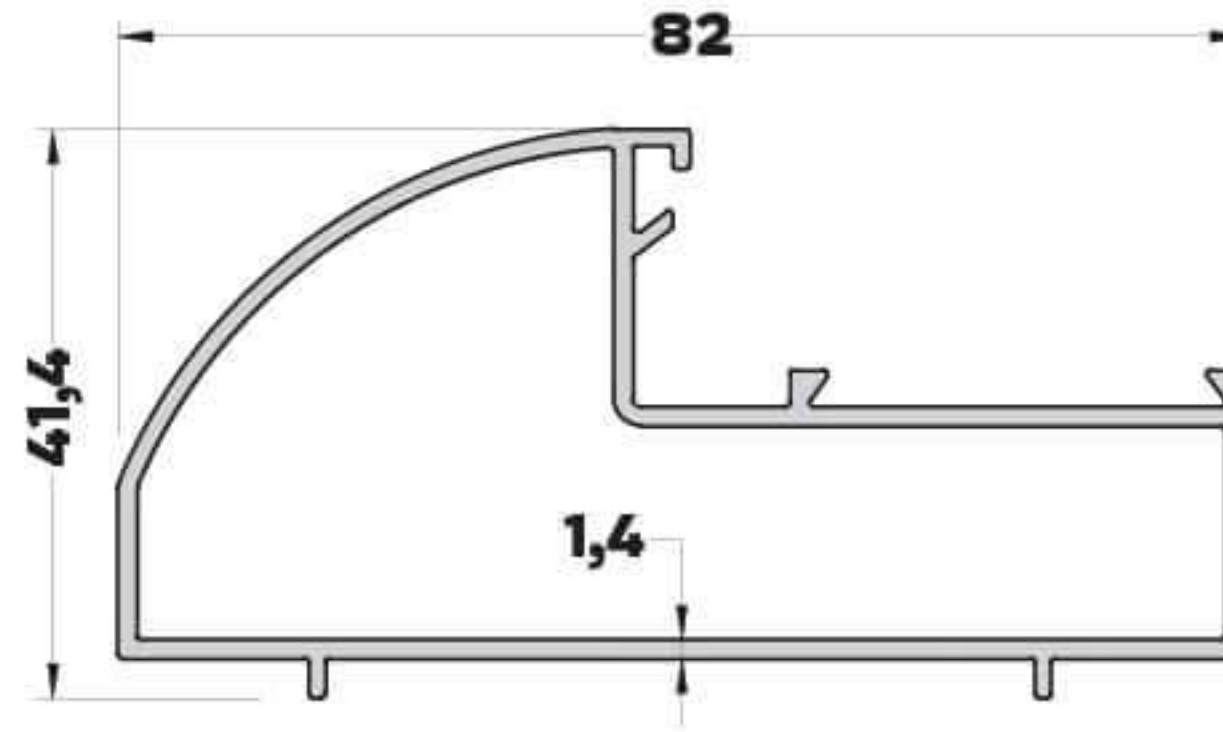
AB-6545 (0,912 kg/mt) KAPI KASA PROFİLİ
