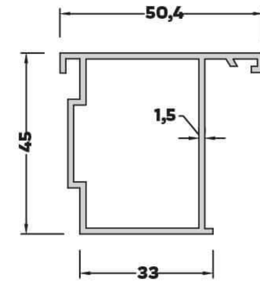
AL-3039 (0,744 kg/mt) PİVOT ADAPTÖR PROFİLİ
