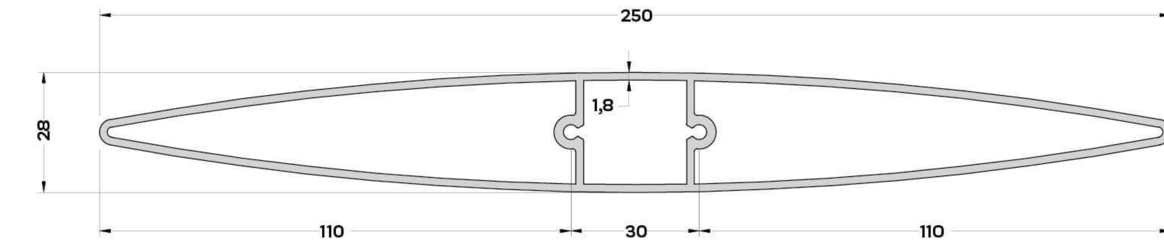
S-4837 (2,570 kg/mt) GÜNEŞ KIRICI PR. 200 mm
