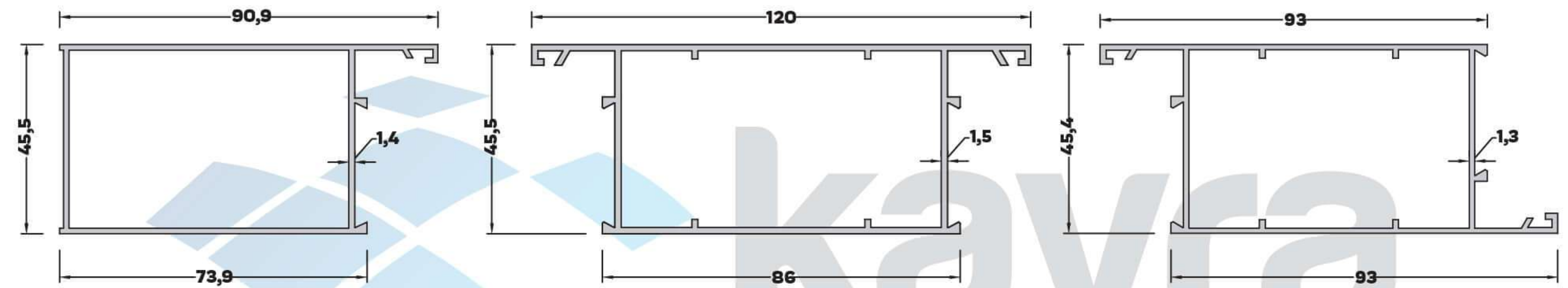
AL-2083 (0,986 kg/mt) BAZA KASA PROFİLİ AL-3038 (1,336 kg/mt) BAZA ORTA KAYIT PROFİLİ AL-3045 (1,088 kg/mt) KAPI KANAT PROFİLİ
