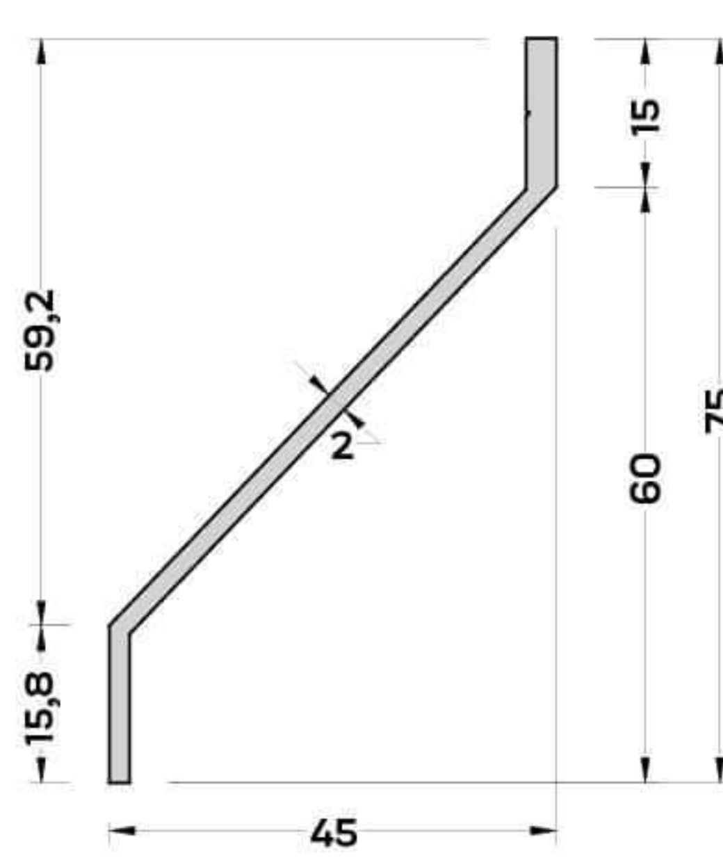
M-5297 (0,538 kg/mt) MENFEZ PROFİLİ
