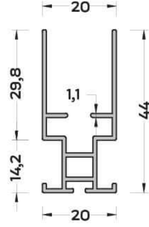
SN-4822 (0,421 kg/mt) SİNEKLİK KANAT PROFİLİ
