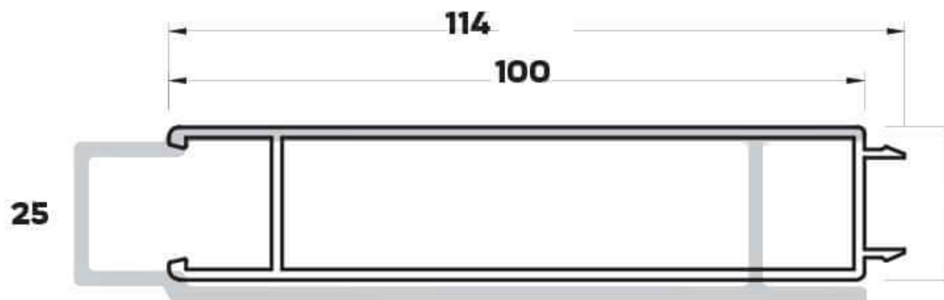
L-4442 (0,886 kg/mt) LAMBRI PROFİLİ
