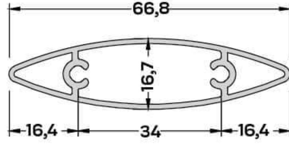
GK-10740 (0,594 kg/mt) GÜNEŞ KIRICI PR. 66,8 mm
