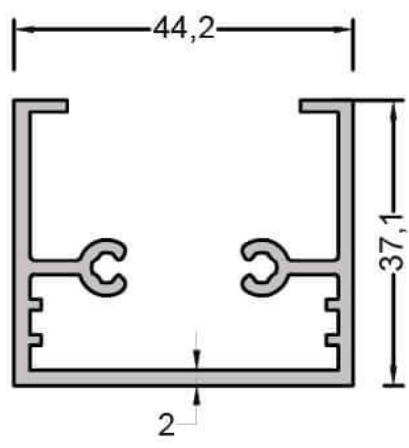
M-8905 ( 2,150 kg/mt ) ÜST RAY PROFİLİ
