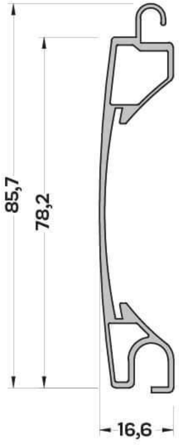
P-7056 (0,315 kg/mt) PANJUR LAMEL PROFİLİ
