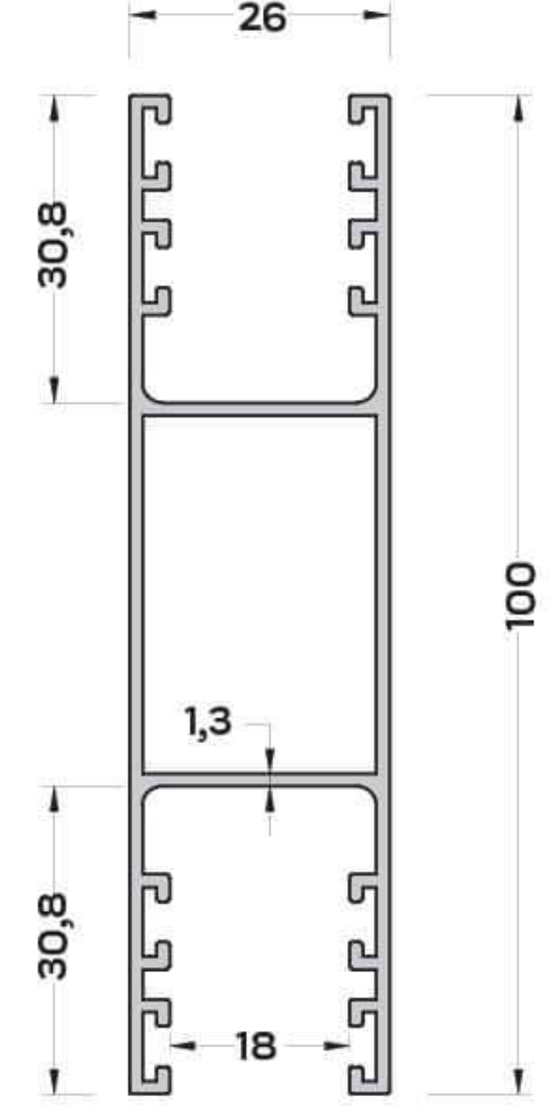
P-3453 (1,111 kg/mt) PANJUR ORTA KASA PROFİLİ
