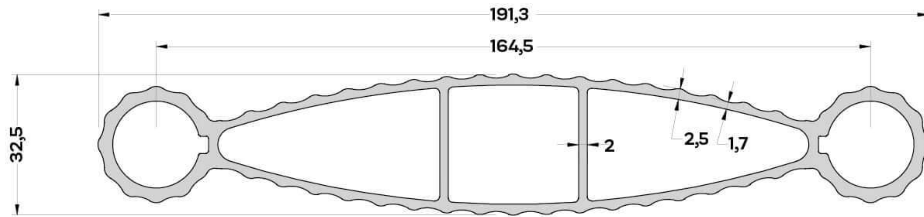
S-5355 (3,069 kg/mt) GÜNEŞ KIRICI PR. 191,3 mm
