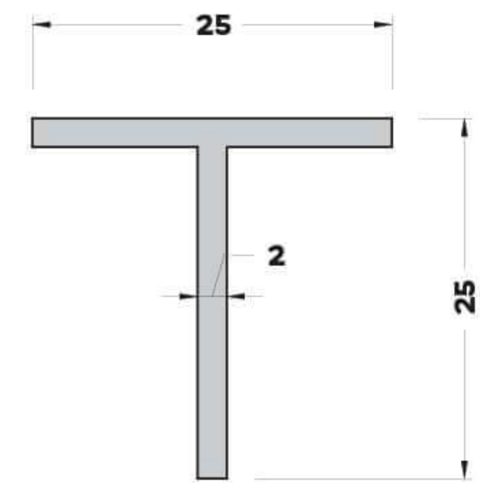
T-1183 (0,273 kg/mt) T BİNİ PROFİLİ
