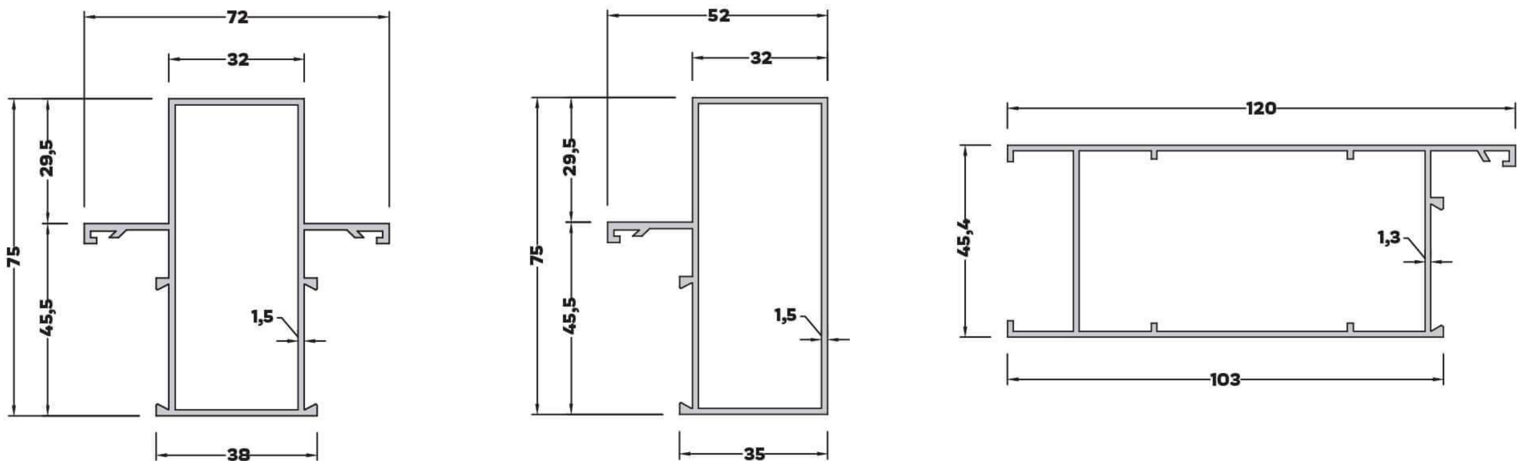
AL-3087 (1,144 kg/mt) TEKVİYELİ ORTA KAYIT PR. AL-3086 (0,996 kg/mt) TEKVİYELİ ORTA KAYIT PR. AL-3069 (1,220 kg/mt) ETEK PROFİLİ
