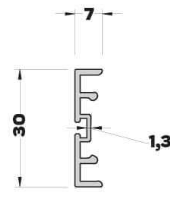
AB-6635 (0,203 kg/mt) KAPAK PROFİLİ
