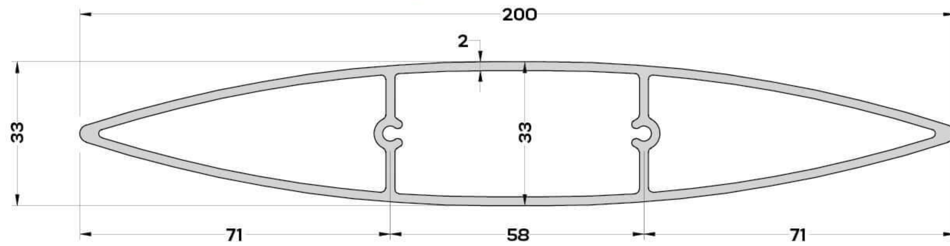
S-4472 (2,464 kg/mt) GÜNEŞ KIRICI PR. 200 mm
