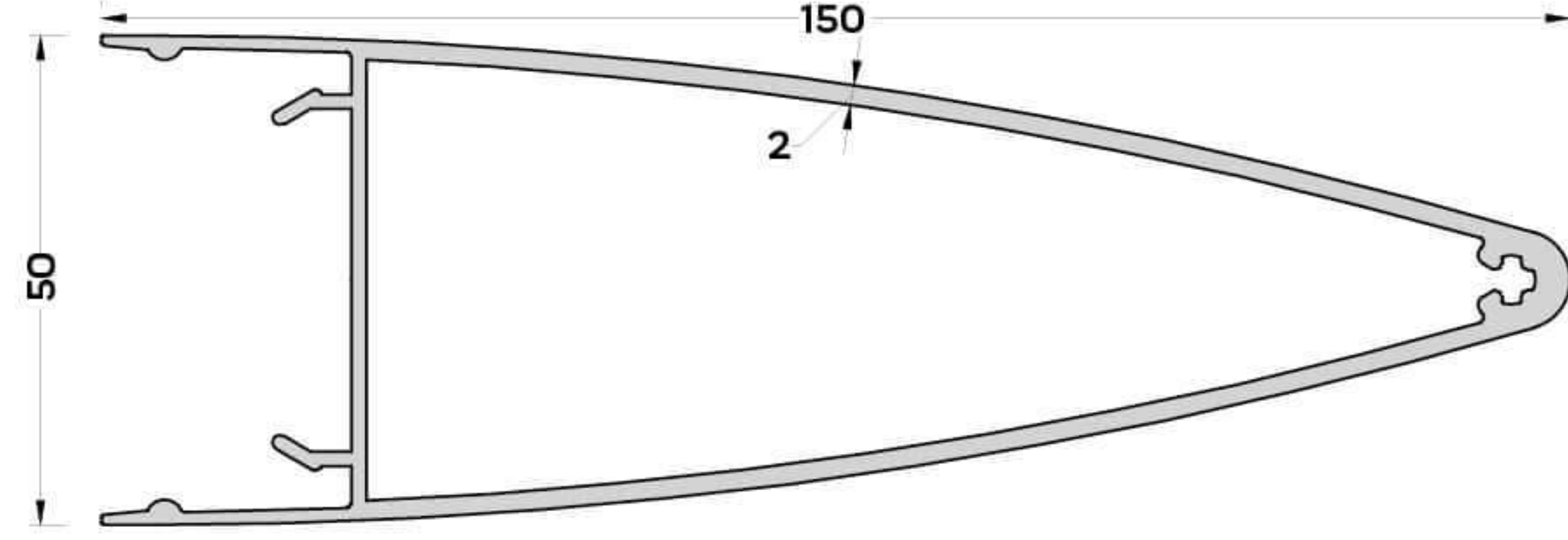
S-4000 (1,905 kg/mt) GÜNEŞ KIRICI PR.
