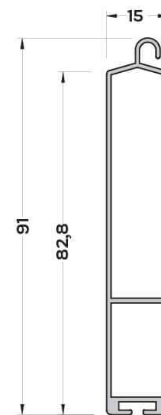
P-3046 (0,340 kg/mt) PANJUR ETEK PROFİLİ
