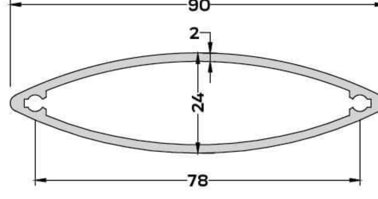
S-5447 (1,022 kg/mt) GÜNEŞ KIRICI PR. 90 mm
