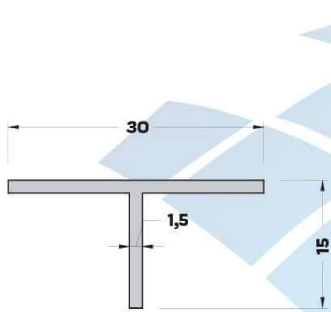
T-704 (0,160 kg/mt) T BİNİ PROFİLİ
