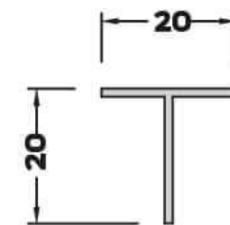
T-4680 (0,126 kg/mt) T BİNİ PROFİLİ
