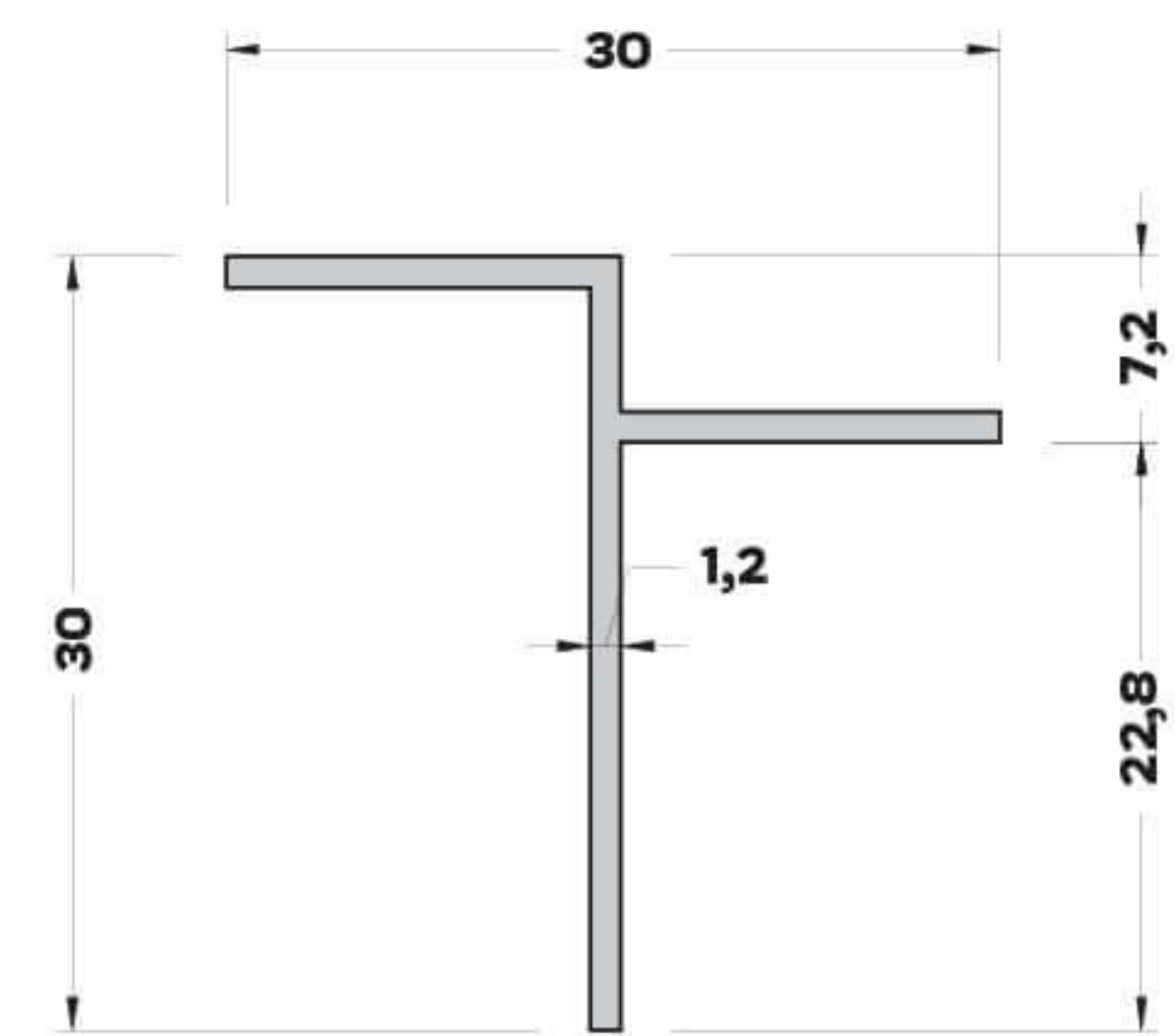
T-5527 (0,200 kg/mt.) ASİMETRİK T BİNİ PROFİLİ
