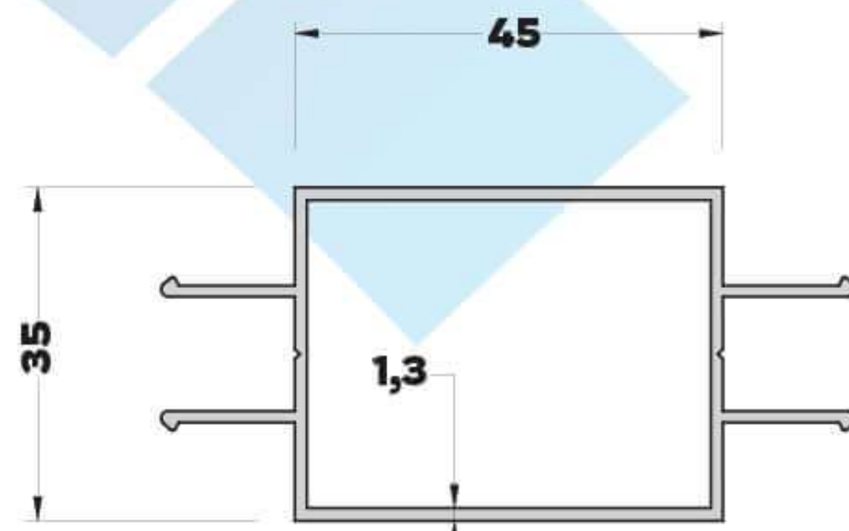
AB-6637 (0,692 kg/mt) TAŞIYICI GÖVDE PROFİLİ
