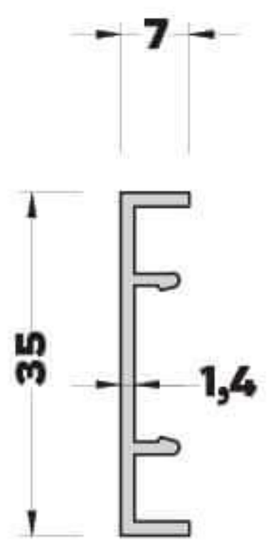
AB-6638 (0,203 kg/mt) KAPAK PROFİLİ
