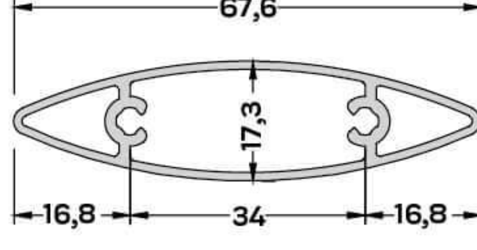
S-8960 (0,620 kg/mt) GÜNEŞ KIRICI PR. 67,6 mm
