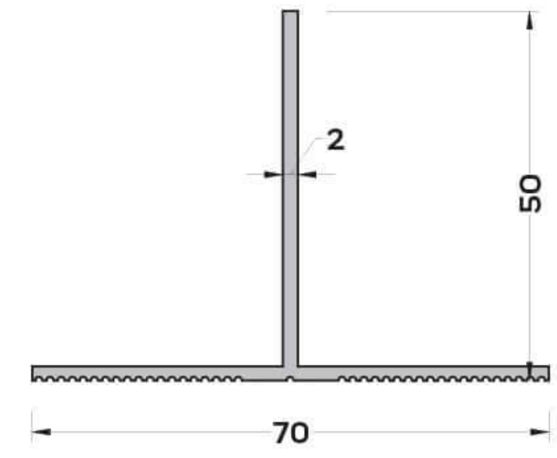
CK-6754 (0,601 kg/mt) T PROFİLİ
