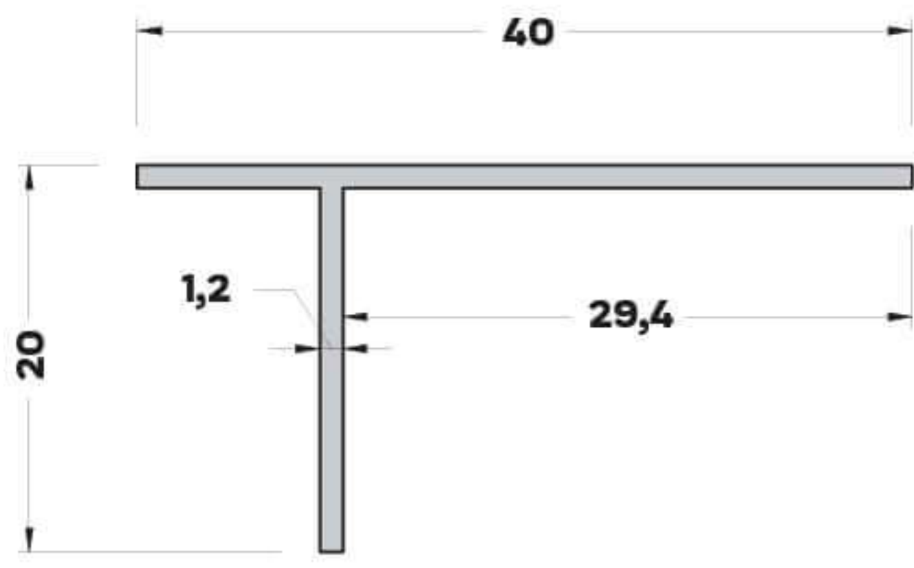
T-2969 (0,324 kg/mt.) T BİNİ PROFİLİ
