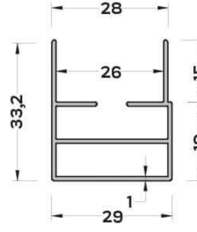
SN-6231 (0,383 kg/mt) SİNEKLİK RAY PROFİLİ
