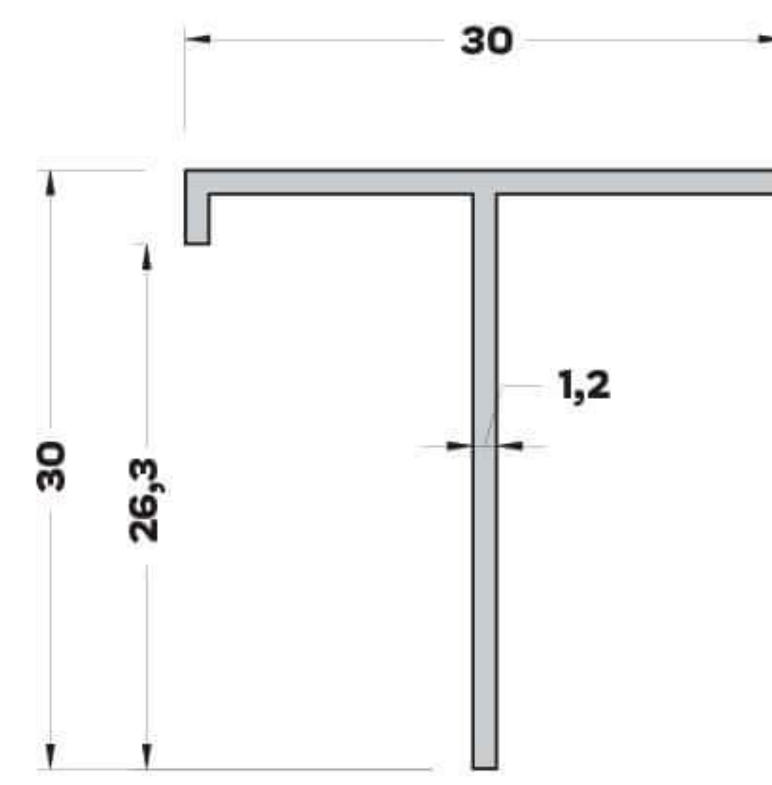
T-5575 (0,205 kg/mt.) T BİNİ PROFİLİ
