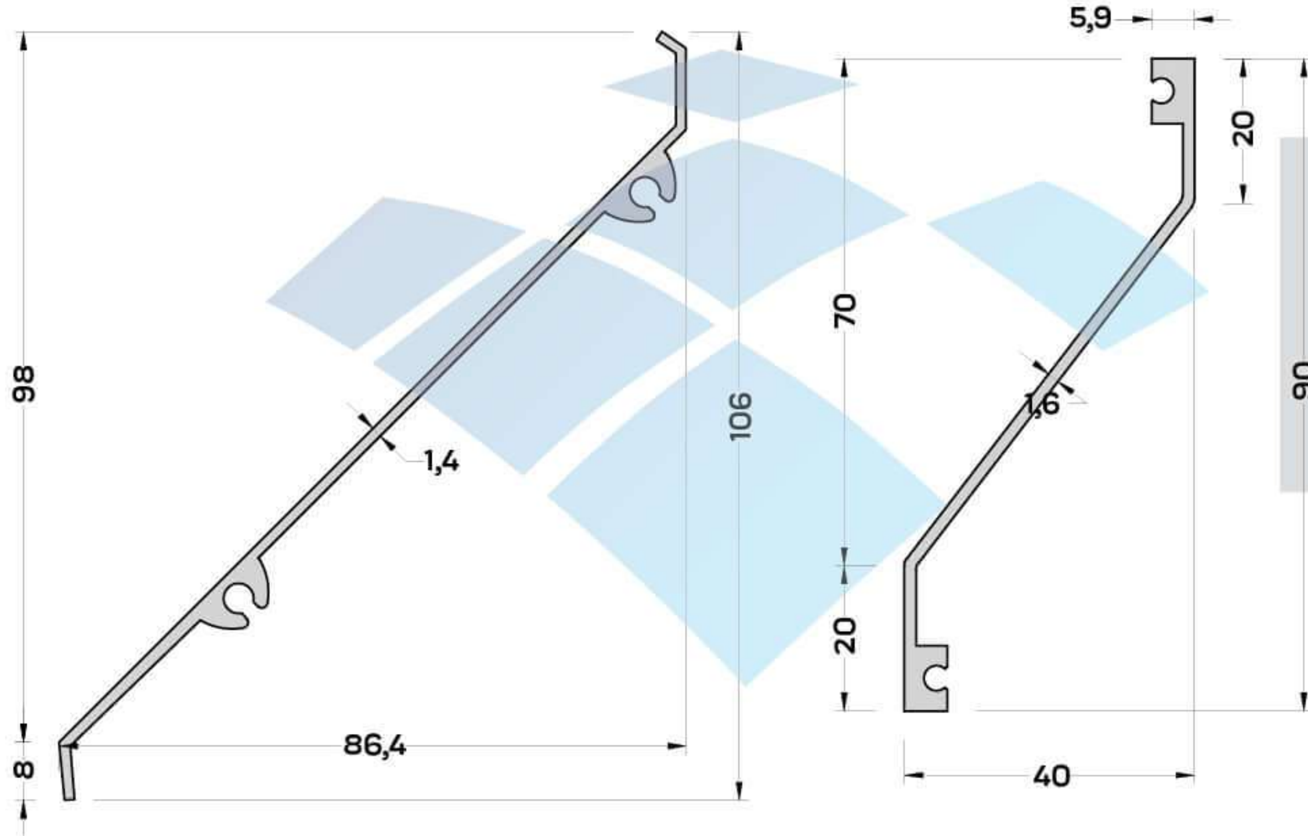
M-3757 (0,720 kg/mt) MENFEZ PROFİLİ
