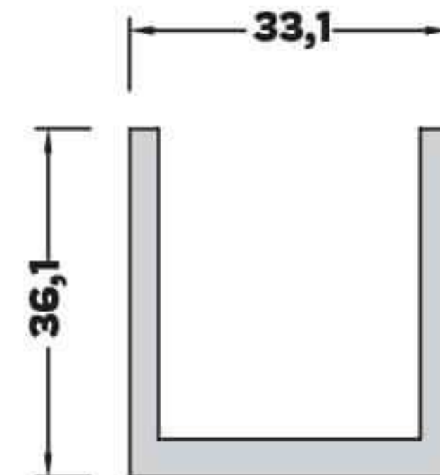
AL-1216 (0,878 kg/mt) GENİŞ U BAĞLANTI PROFİLİ
