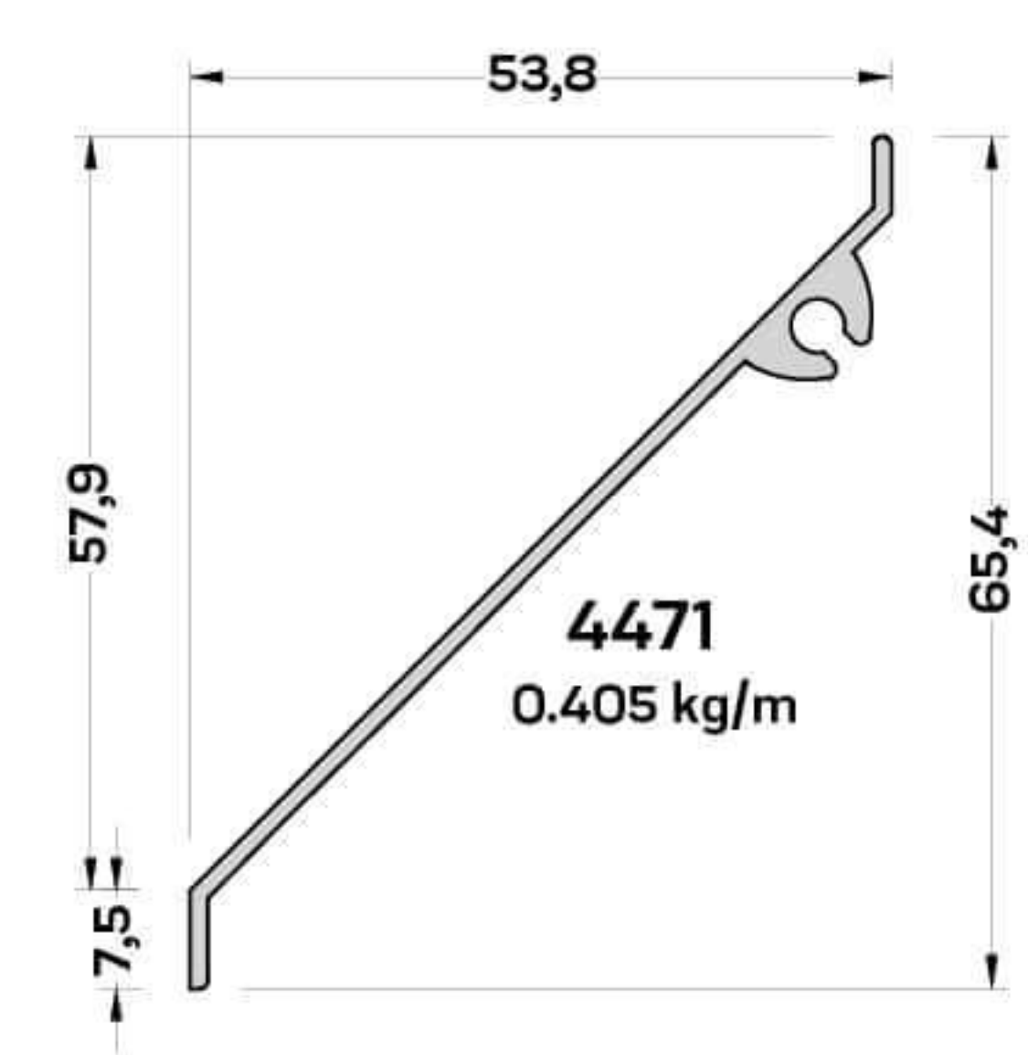
M-4471 (0,405 kg/mt) MENFEZ PROFİLİ
