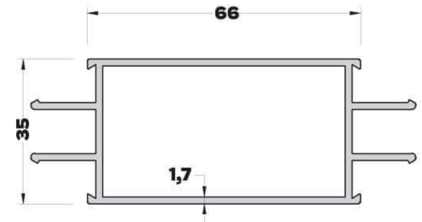
AB-4476 (0,965 kg/mt) KAPI KASA PROFİLİ
