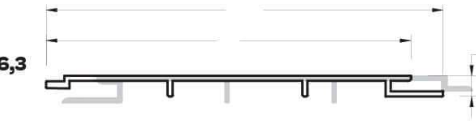
L-124 (0,237 kg/mt) LAMBRI PROFİLİ
