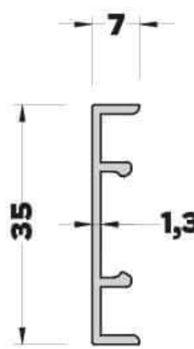
AB-6638 (0,203 kg/mt) KAPAK PROFİLİ
