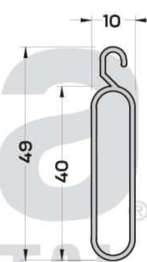
P-3453 (1,111 kg/mt) PANJUR ORTA KASA PROFİLİ
