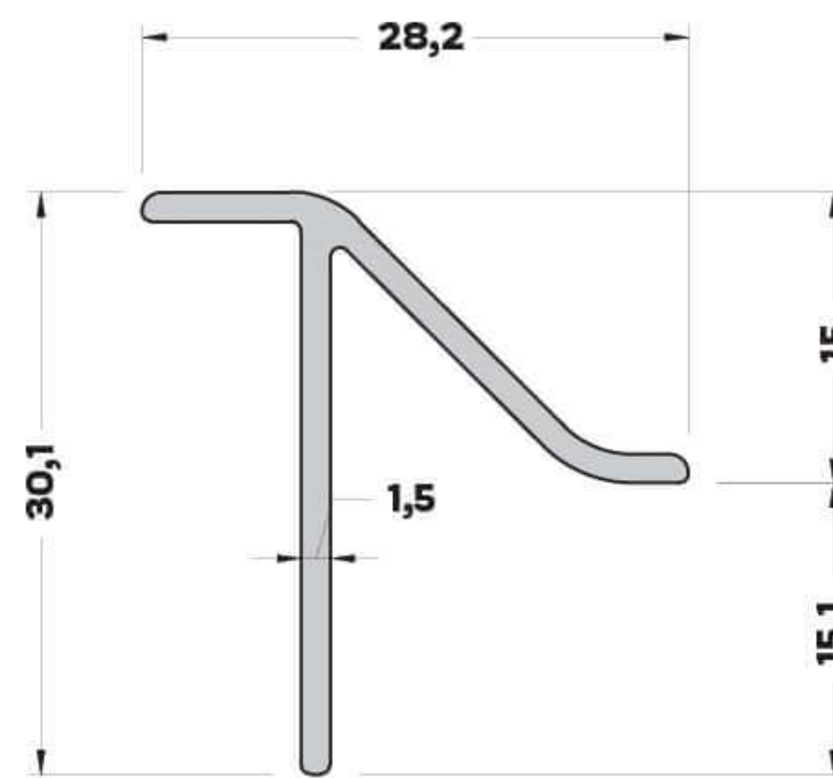
T-266 (0,250 kg/mt.) ASİMETRİK T BİNİ PROFİLİ
