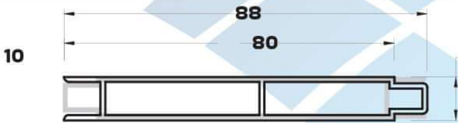
L-1640 (0,998 kg/mt) LAMBRI PROFİLİ
