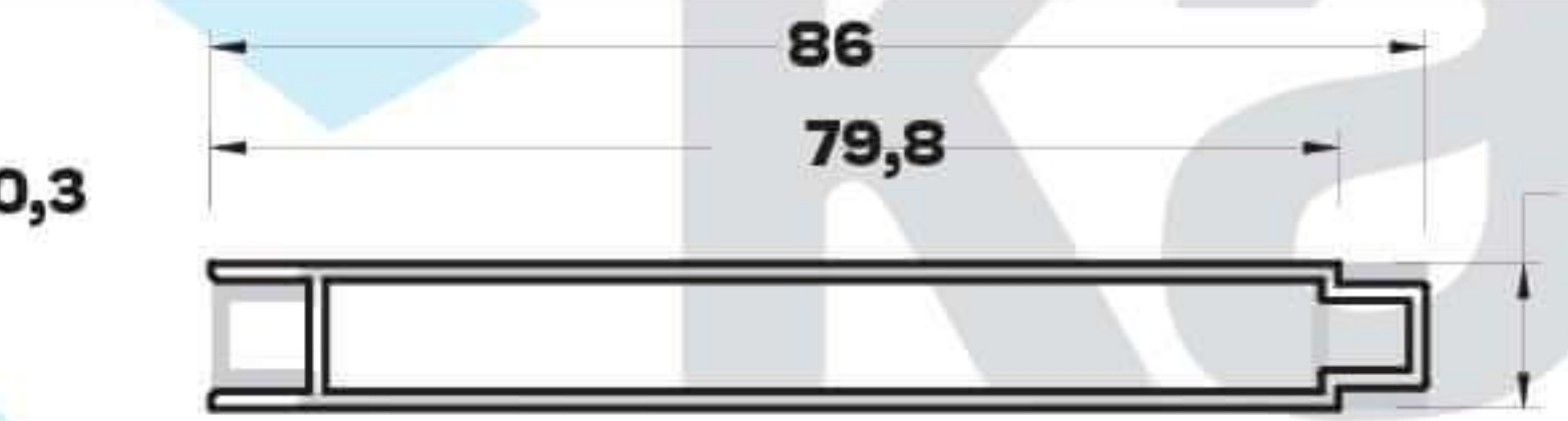
L-4426 (0,925 kg/mt) LAMBRI PROFİLİ
