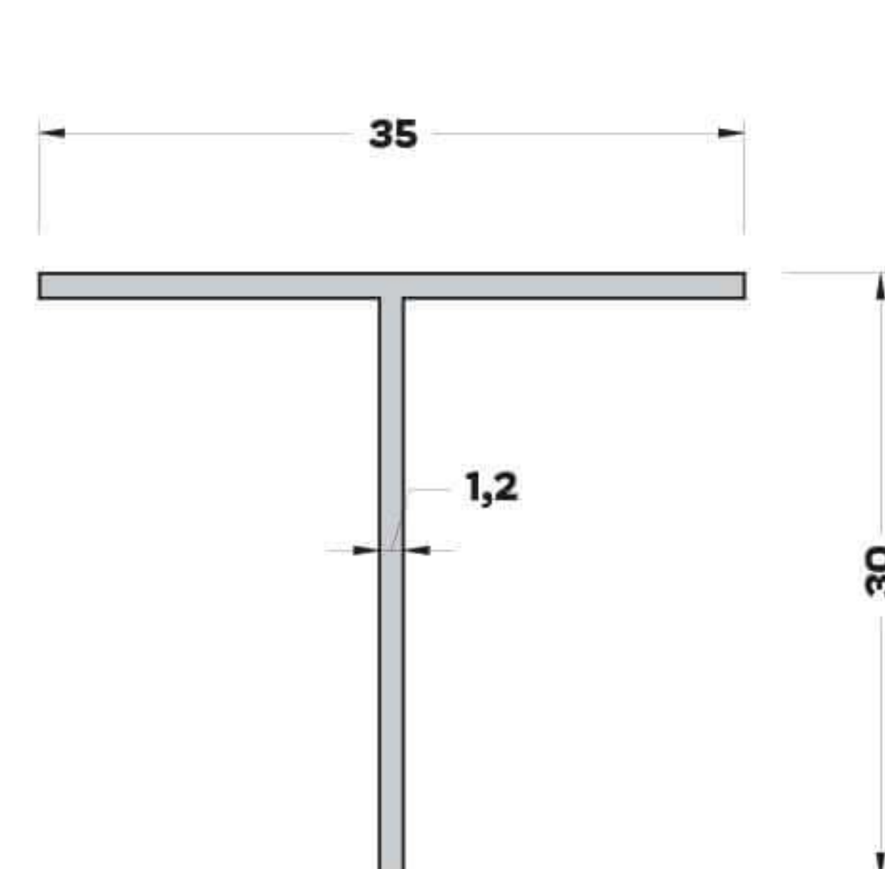
T-3063(0,176 kg/mt) T BİNİ PROFİLİ
