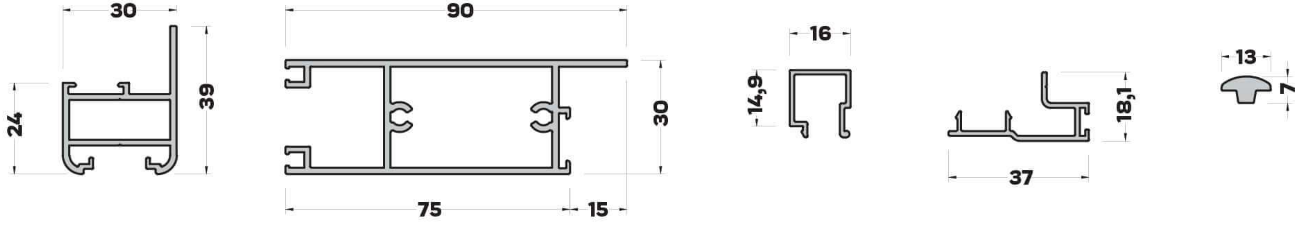
FS-11043 (0,469 kg/mt) FOTOSEL KANAT DIKME PROFİLİ
