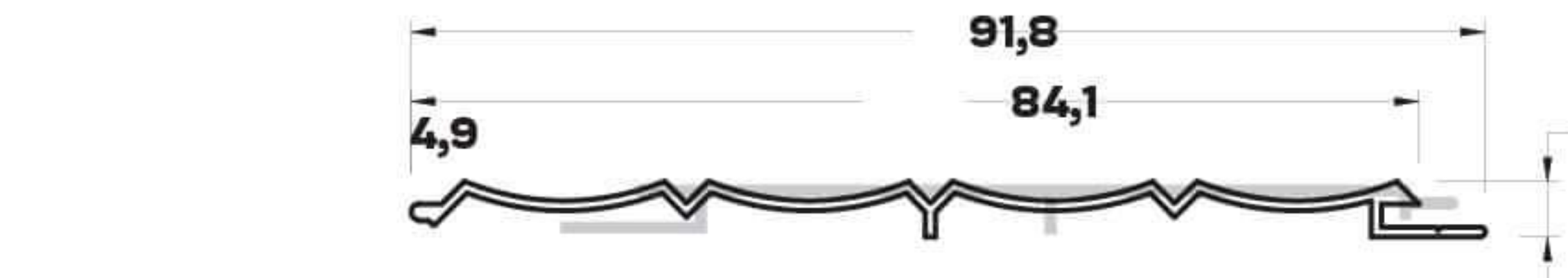
L-2000/12 (0,395 kg/mt) LAMBRI PROFİLİ
