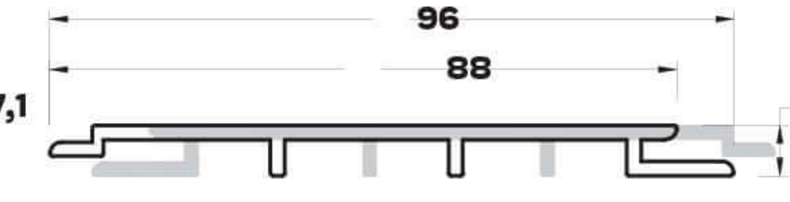
L-114 (0,336 kg/mt) LAMBRI PROFİLİ
