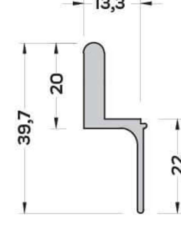
SN-4108 (0,442 kg/mt) SİNEKLİK PROFİLİ
