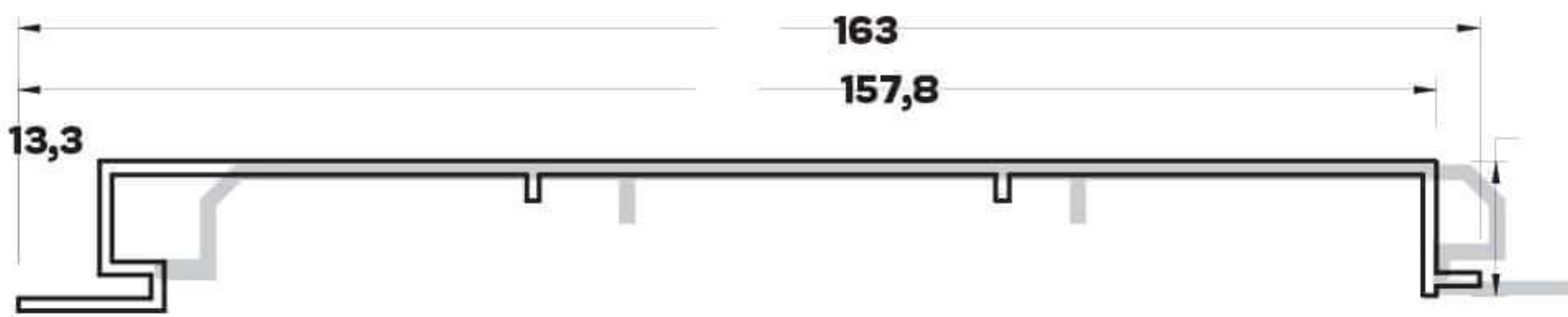
L-3012 (0,329 kg/mt) LAMBRI PROFİLİ
