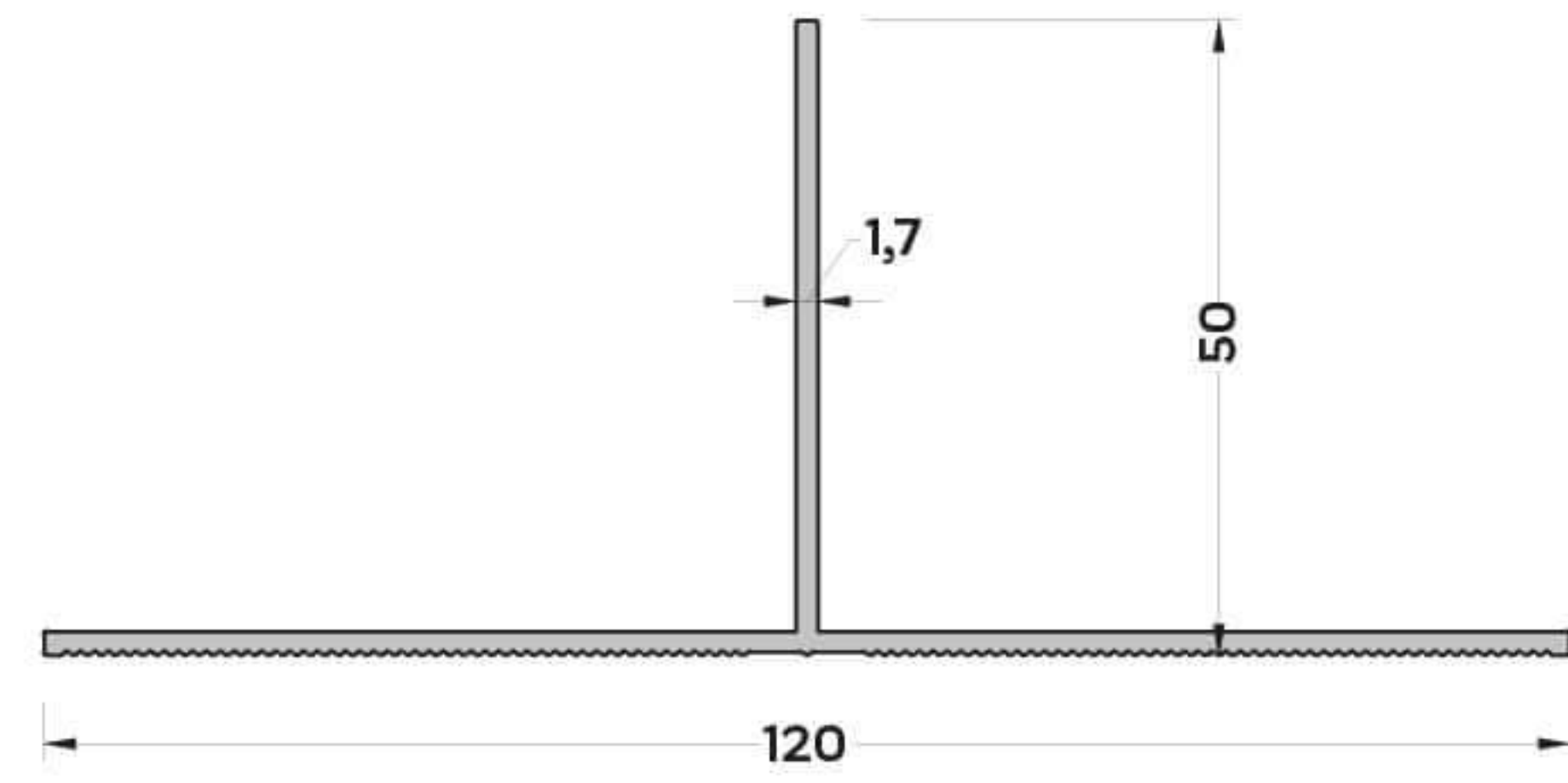
CK-6754 (0,601 kg/mt) T PROFİLİ
