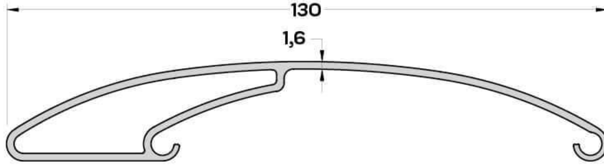
S-4000 (1,905 kg/mt) GÜNEŞ KIRICI PR.
