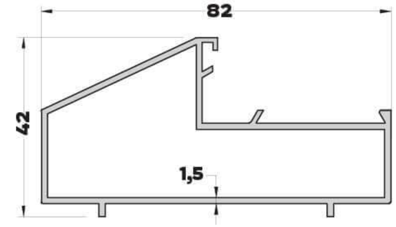
AB-4476 (0,965 kg/mt) KAPI KASA PROFİLİ
