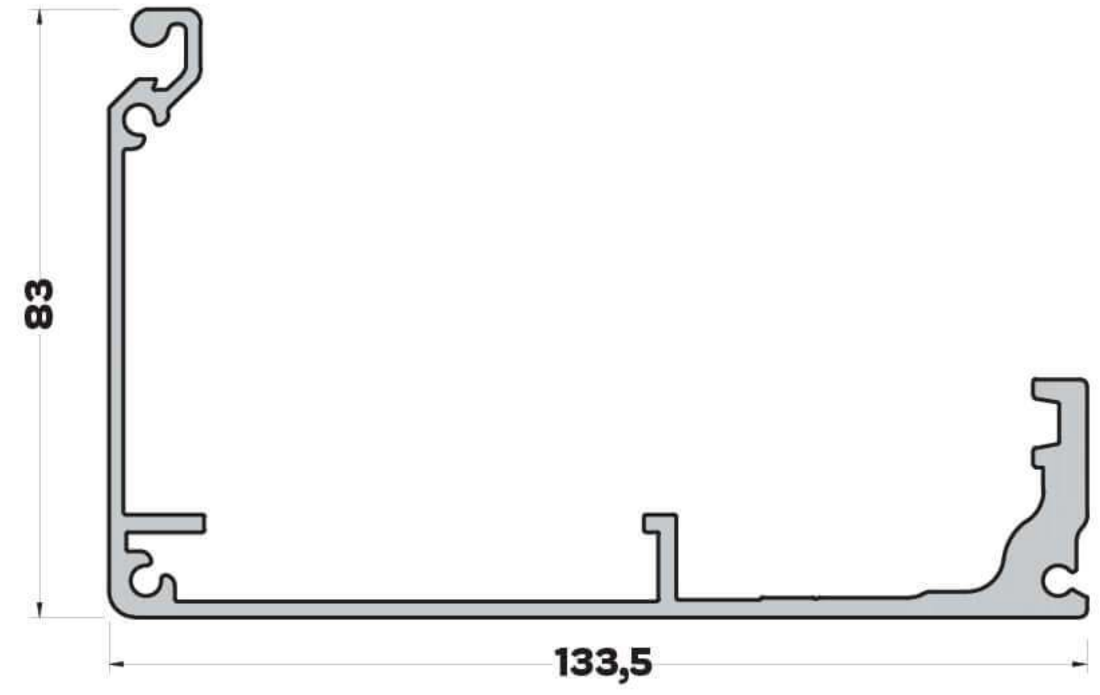
FS-7577 (2,250 kg/mt) FOTOSEL ŞASE PROFİLİ
