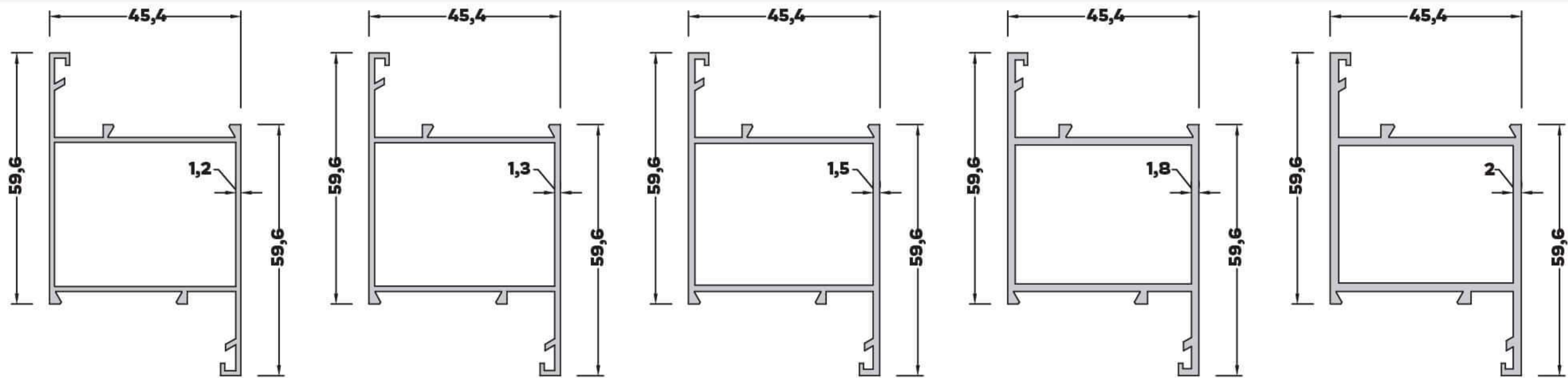
AL-3075 (0,767 kg/mt) GENİŞ KANAT PROFİLİ AL-219 (0,820 kg/mt) GENİŞ KANAT PROFİLİ AL-243 (0,926 kg/mt) GENİŞ KANAT PROFİLİ AL-279 (1,090 kg/mt) GENİŞ KANAT PROFİLİ AL-207 (1,192 kg/mt) GENİŞ KANAT PROFİLİ
