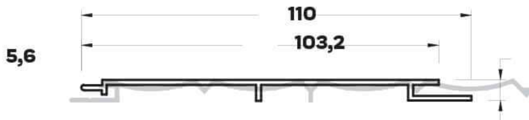
L-1317 (0,635 kg/mt) LAMBRI PROFİLİ
