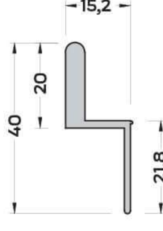
SN-5967 (0,222 kg/mt) SİNEKLİK PROFİLİ
