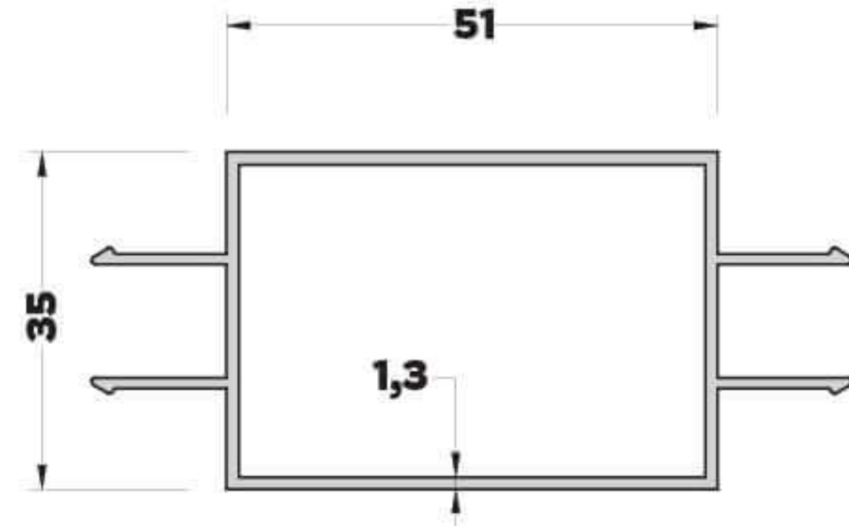
AB-1843 (0,756 kg/mt) TAŞIYICI GÖVDE PROFİLİ
