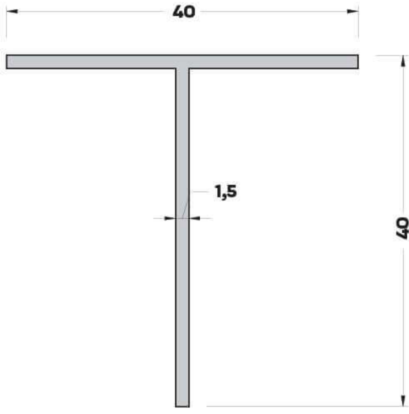
T-2969 (0,324 kg/mt.) T BİNİ PROFİLİ
