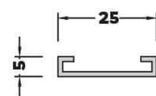
AL-3009 (0,218 kg/mt) TEK CAM ÇITA PROFİLİ
