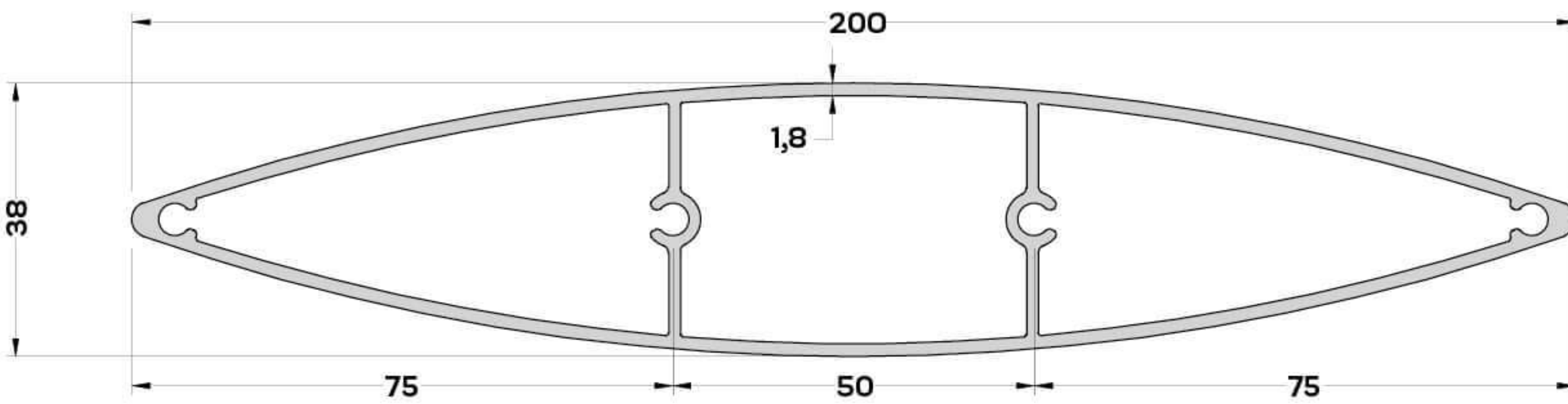
S-5355 (3,069 kg/mt) GÜNEŞ KIRICI PR. 191,3 mm
