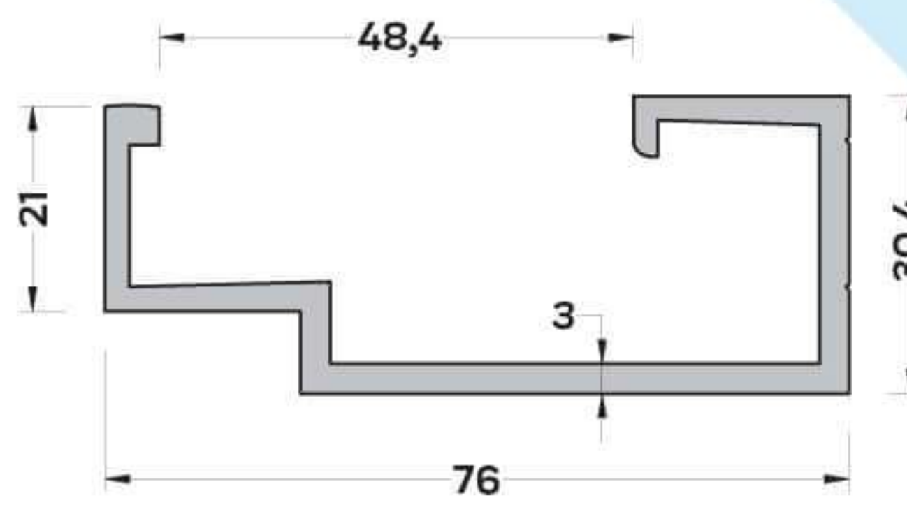
CK-6998 (1,208 kg/mt) KOMPAKT PROFİLİ
