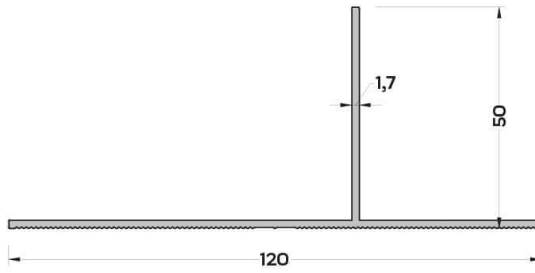
CK-6755 (0,507 kg/mt) T PROFİLİ
