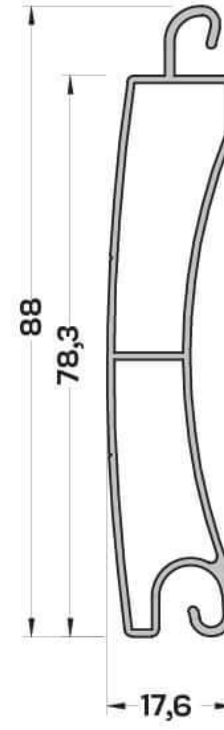
P-7625 (0,645 kg/mt) PANJUR LAMEL PROFİLİ
