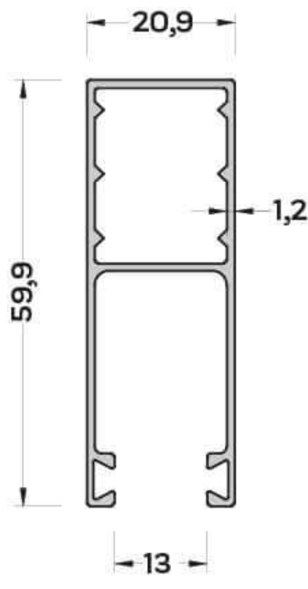
P-3872 (0,470 kg/mt) PANJUR YAN KASA PROFİLİ
