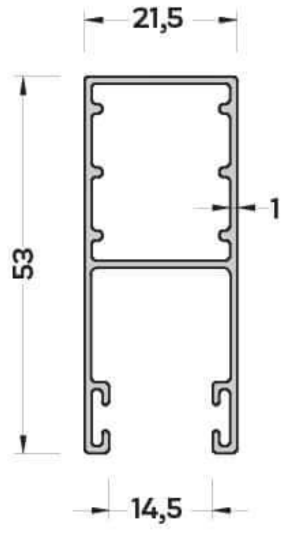
P-3872 (0,470 kg/mt) PANJUR YAN KASA PROFİLİ
