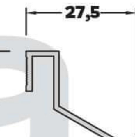
AL-3047 (0,246 kg/mt) DAMLALIK PROFİLİ
