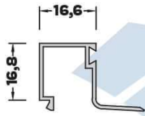
AL-1365 (0,818 kg/mt) 90° KÖŞE DÖNÜŞ PROFİLİ
