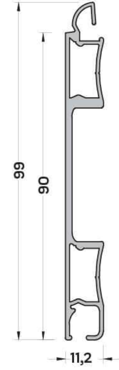
P-7196 (0,790 kg/mt) PANJUR LAMEL PROFİLİ
