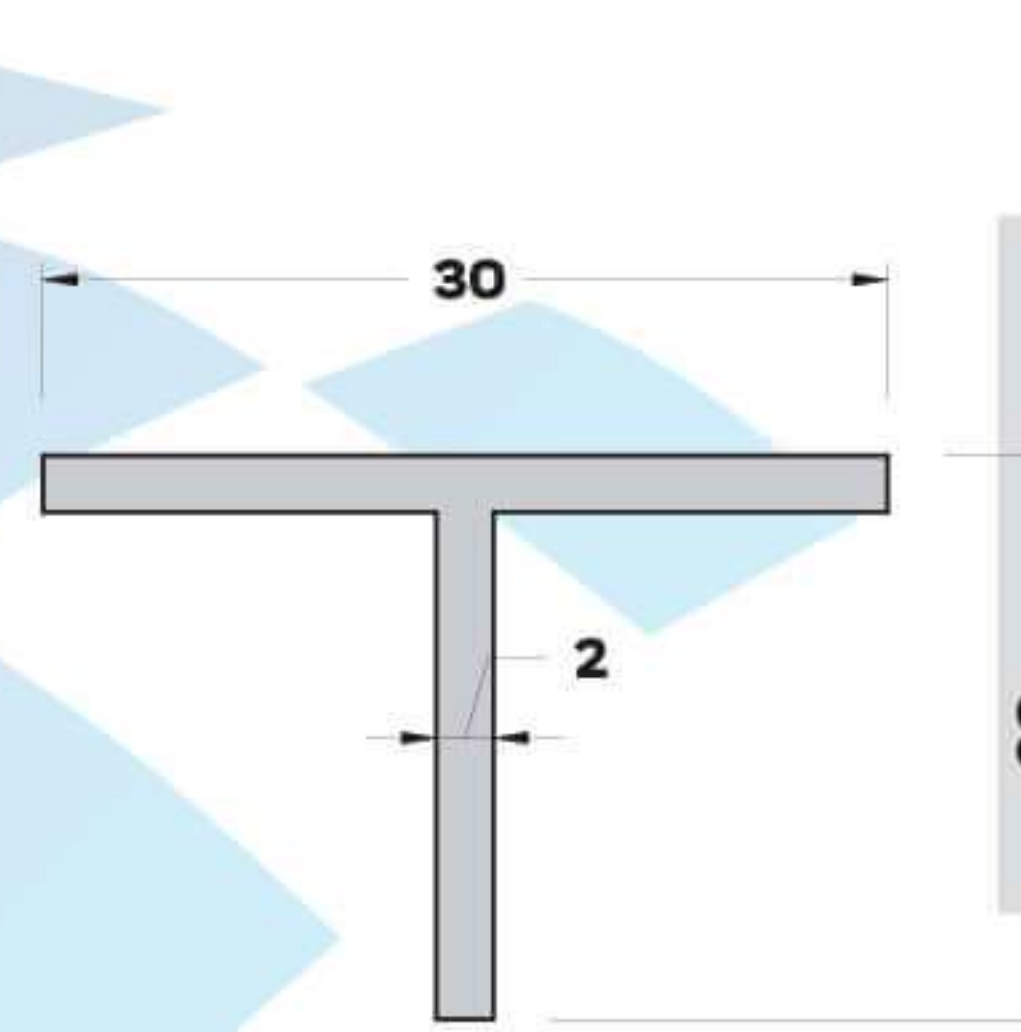
T-156 (0,146 kg/mt) T BİNİ PROFİLİ
