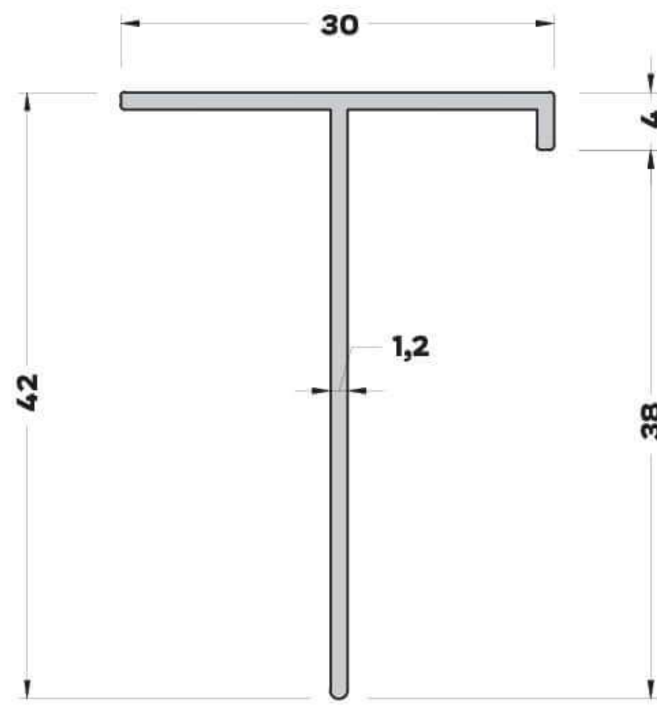
T-1035 (0,239 kg/mt) T BİNİ PROFİLİ
