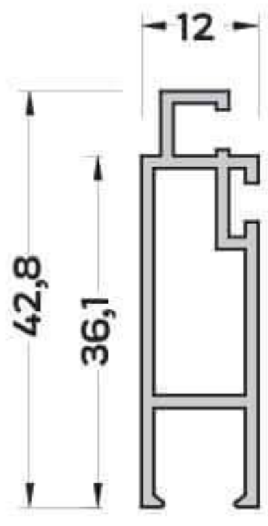
SN-1444 (0,261 kg/mt) SİNEKLİK PROFİLİ
