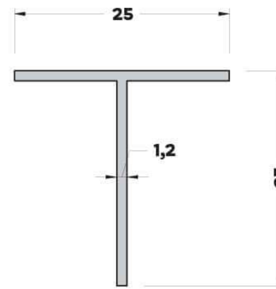
T-3062(0,158 kg/mt) T BİNİ PROFİLİ
