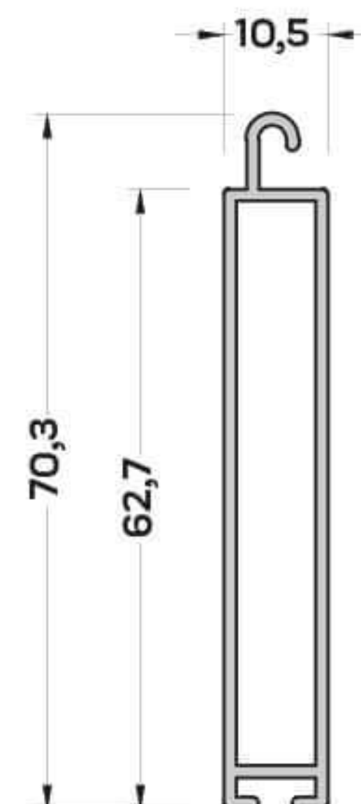
P-1901 (0,295 kg/mt) PANJUR ETEK PROFİLİ
