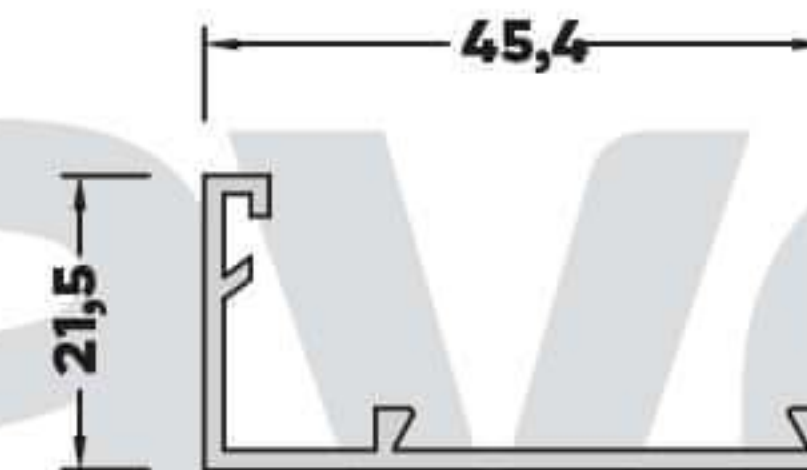
AL-3039 (0,744 kg/mt) PİVOT ADAPTÖR PROFİLİ
