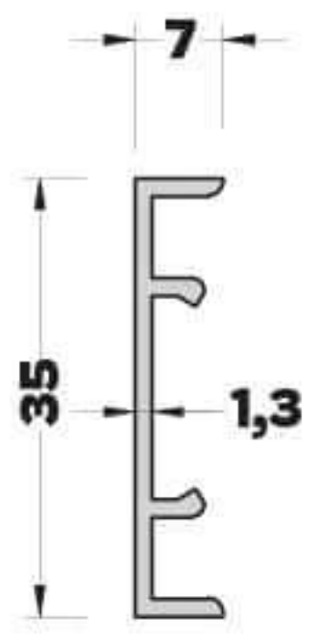
AB-1844 (0,197 kg/mt) KAPAK PROFİLİ
