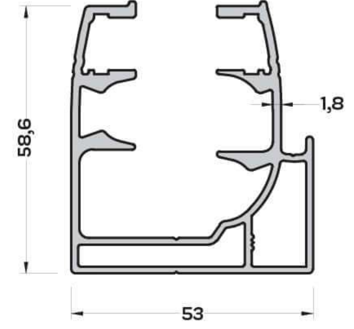
900-1102 (1,548 kg/mt) FIRTINA KASA PROFİLİ
