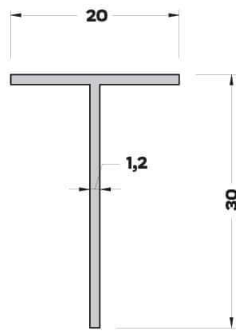
T-4681 (0,093 kg/mt) T BİNİ PROFİLİ
