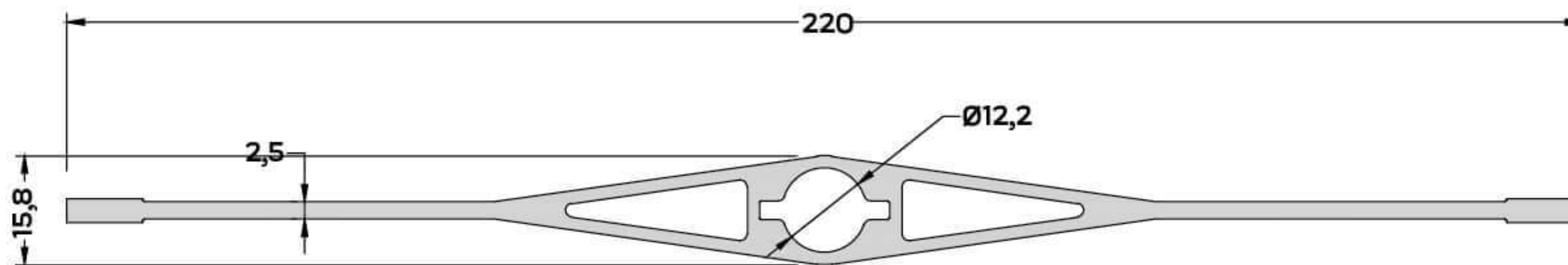
S-7348 (2,515 kg/mt) GÜNEŞ KIRICI PR. 200 mm
