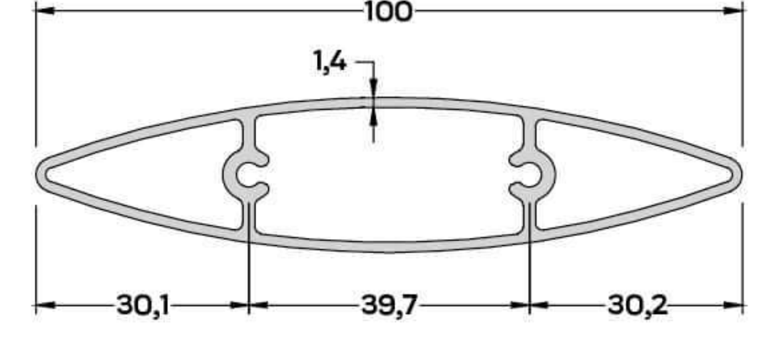
S-4834 (1,016 kg/mt) GÜNEŞ KIRICI PR. 100 mm
