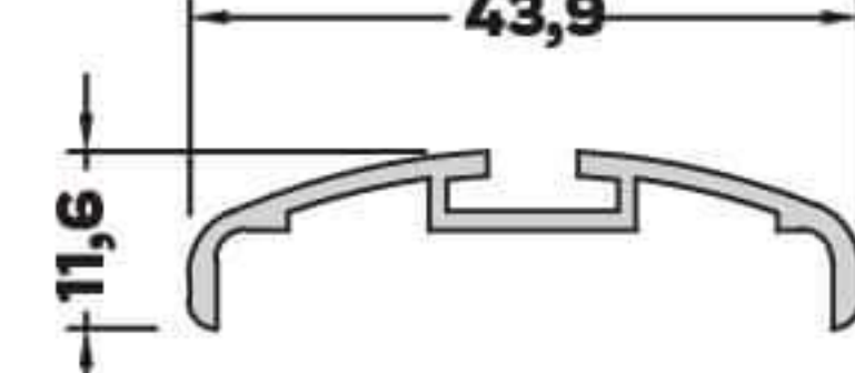
AL-3628 (0,231 kg/mt) EĞİMLİ TEK CAM ÇITA PR.
