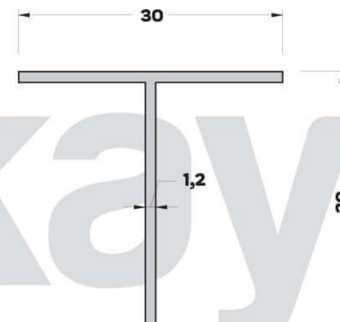
T-3062(0,158 kg/mt) T BİNİ PROFİLİ
