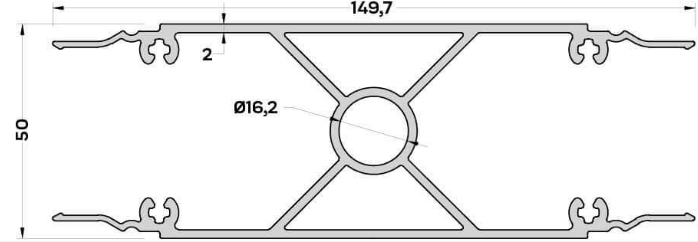
S-4004 (2,666 kg/mt) GÜNEŞ KIRICI PR.
