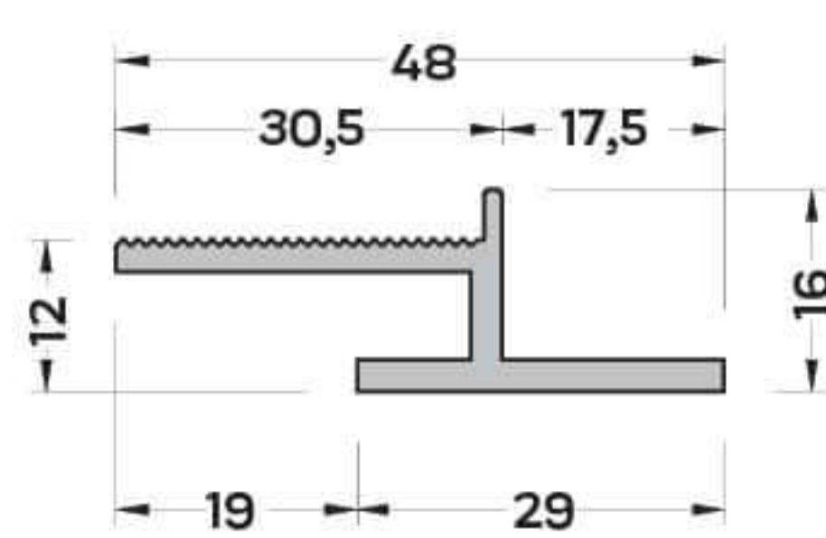
CK-6751 (0,446 kg/mt) ÜST ASKI PROFİLİ
