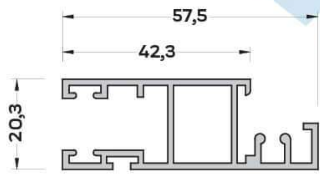
SN-2780 (0,400 kg/mt) SİNEKLİK PROFİLİ
