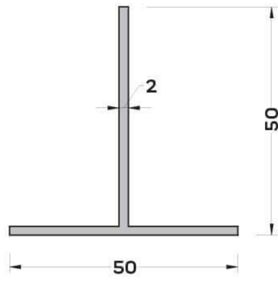
CK-6312 (0,531 kg/mt) T PROFİLİ
