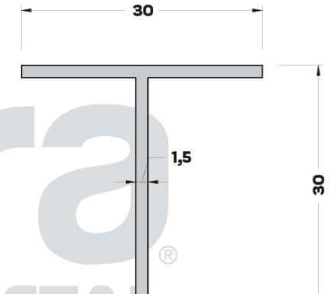
T-1183 (0,273 kg/mt) T BİNİ PROFİLİ
