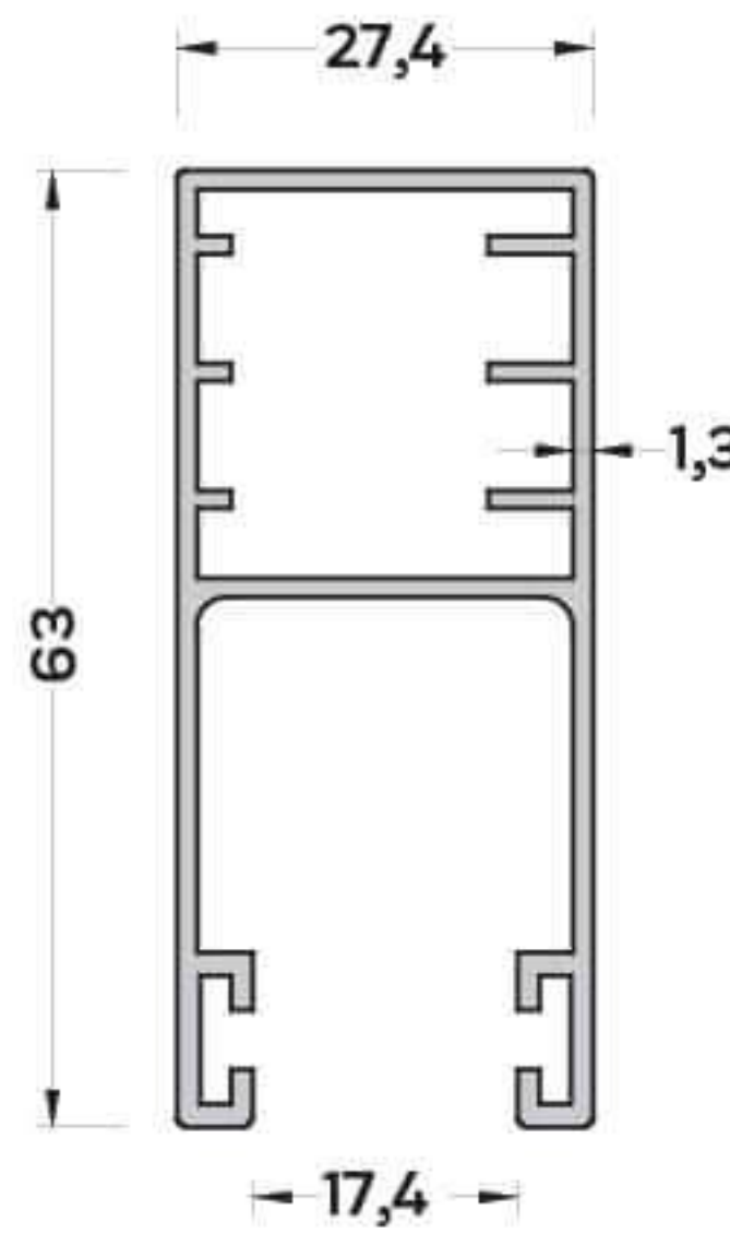
P-5042 (0,614 kg/mt) PANJUR YAN KASA PROFİLİ
