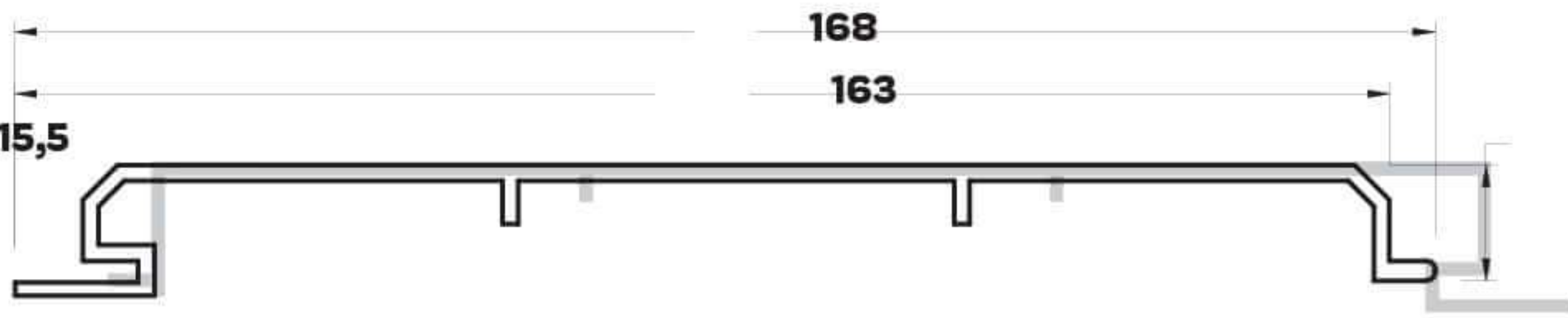
L-1853 (0,360 kg/mt) LAMBRI PROFİLİ
