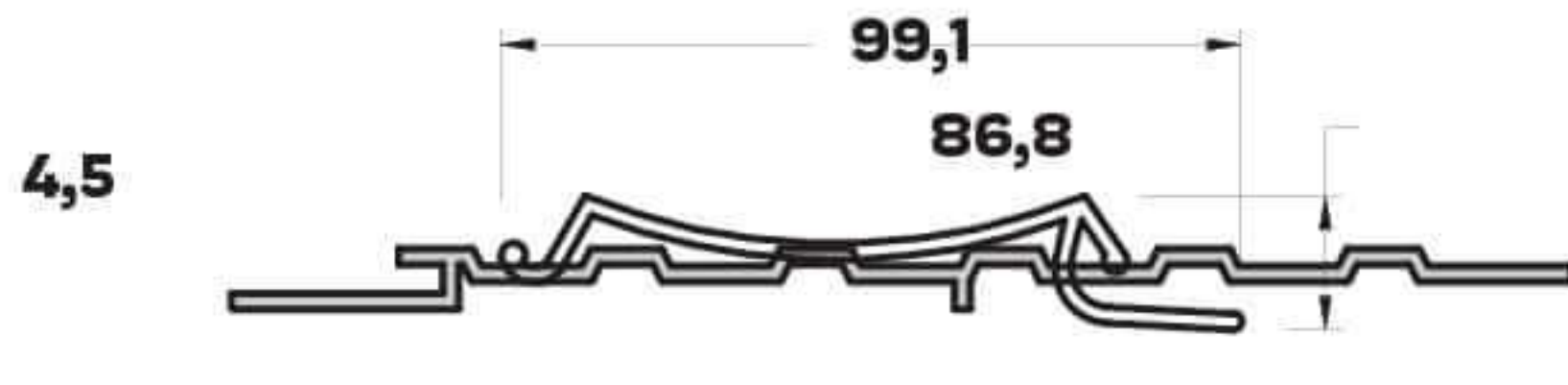
L-222 (0,378kg/mt) LAMBRI PROFİLİ
