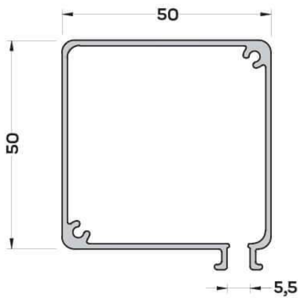
SN-3926 (0,804 kg/mt) SİNEKLİK PROFİLİ
