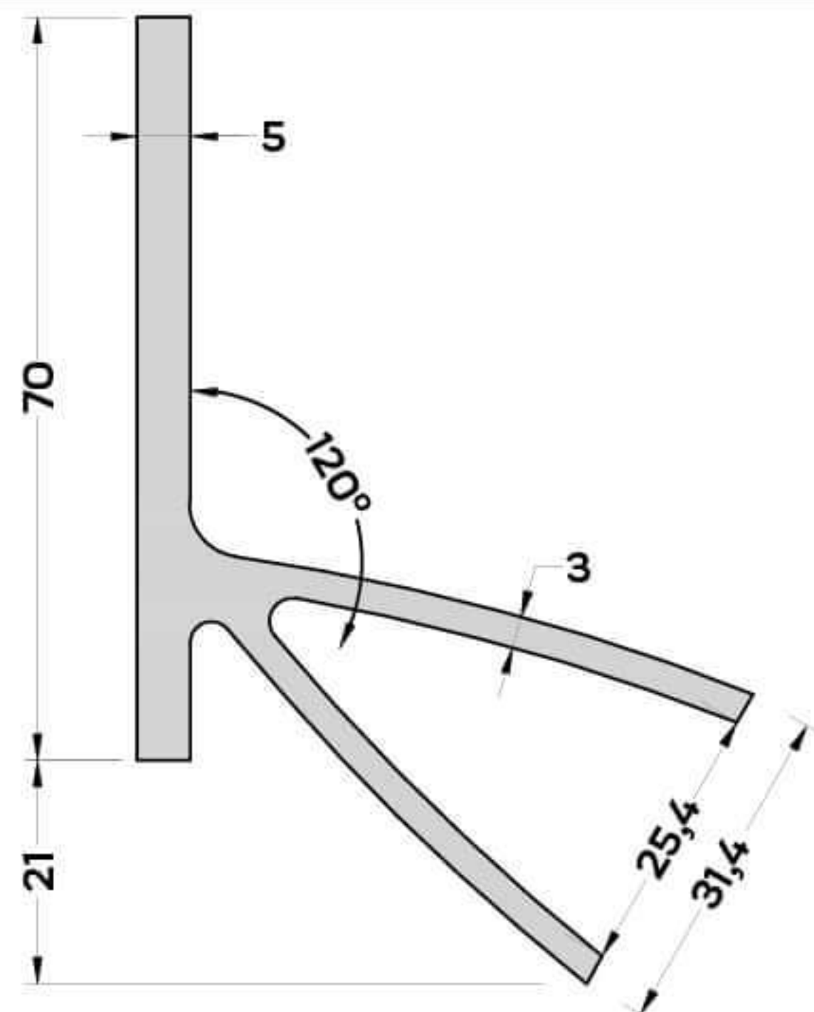
S-10069 (1,539 kg/mt) GÜNEŞ KIRICI AYAK PR.
