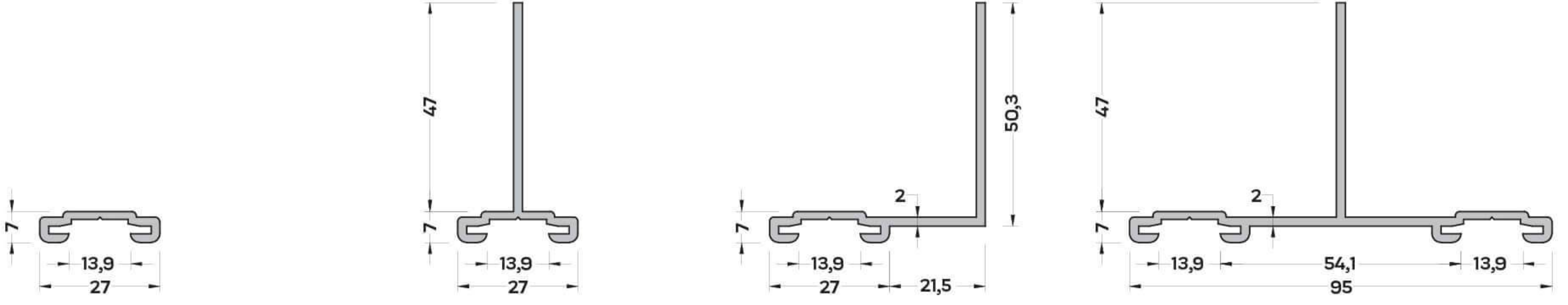
CK-4289 (0,226 kg/mt) SERAMİK CEPHE PR. 4289
