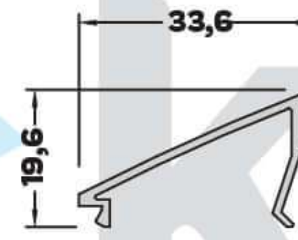
AL-5995 (0,787 kg/mt) 90° KÖŞE DÖNÜŞ PROFİLİ
