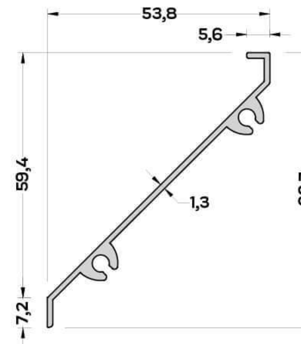
M-3164 (0,477 kg/mt) MENFEZ PROFİLİ
