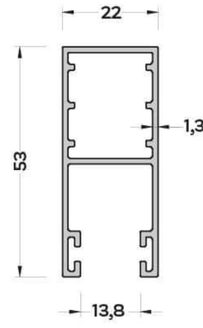
P-5042 (0,614 kg/mt) PANJUR YAN KASA PROFİLİ
