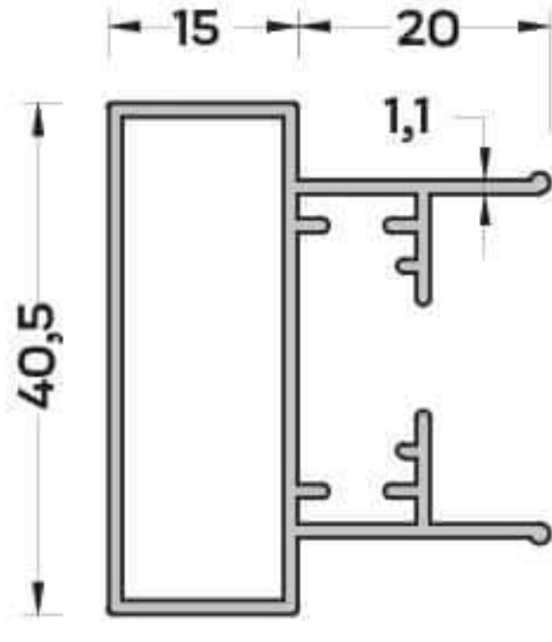
SN-4330 (0,528 kg/mt) SİNEKLİK DİKME PROFİLİ
