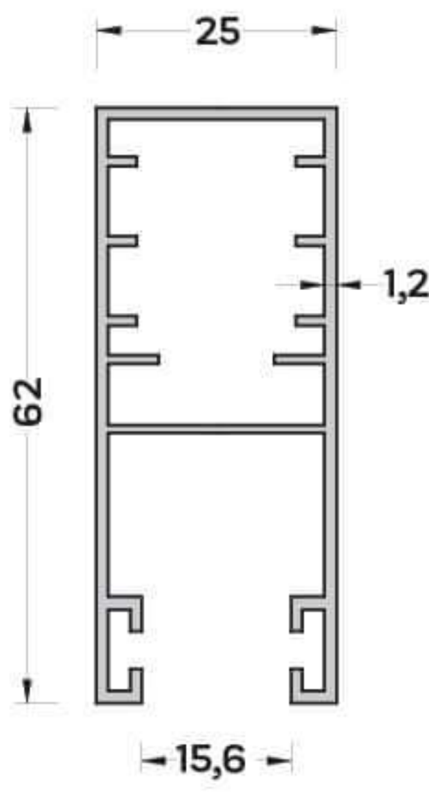
P-3948 (0,475 kg/mt) PANJUR YAN KASA PROFİLİ
