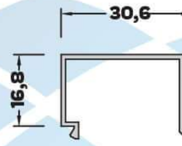
AL-3009 (0,218 kg/mt) TEK CAM ÇITA PROFİLİ
