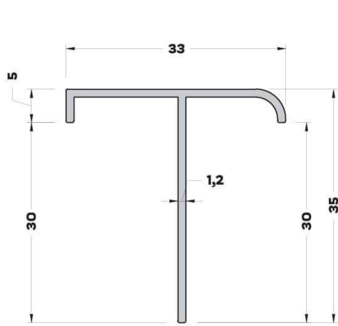
T-1139 (0,239 kg/mt) T BİNİ PROFİLİ
