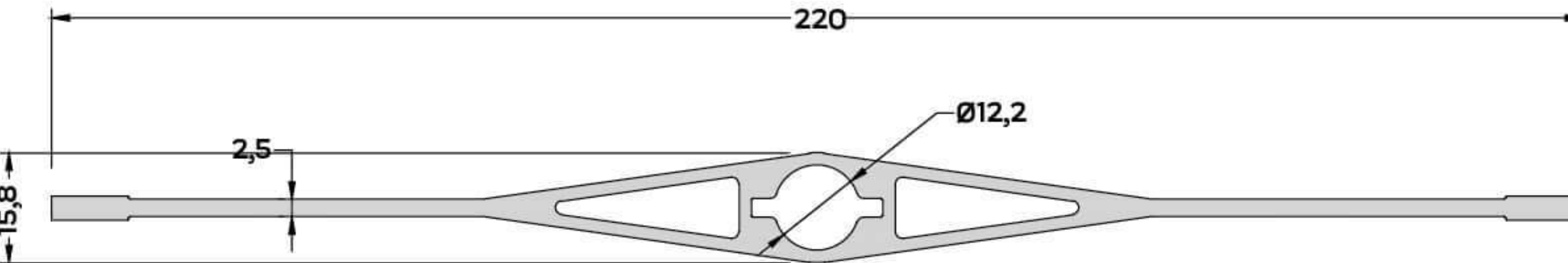
S-7348 (2,515 kg/mt) GÜNEŞ KIRICI PR. 200 mm
