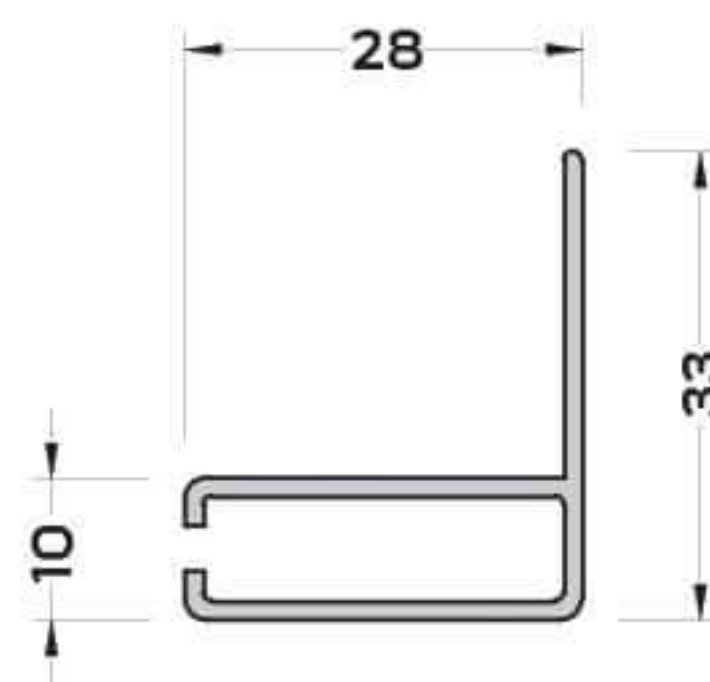
SN-1437 (0,316 kg/mt) SİNEKLİK F PROFİLİ
