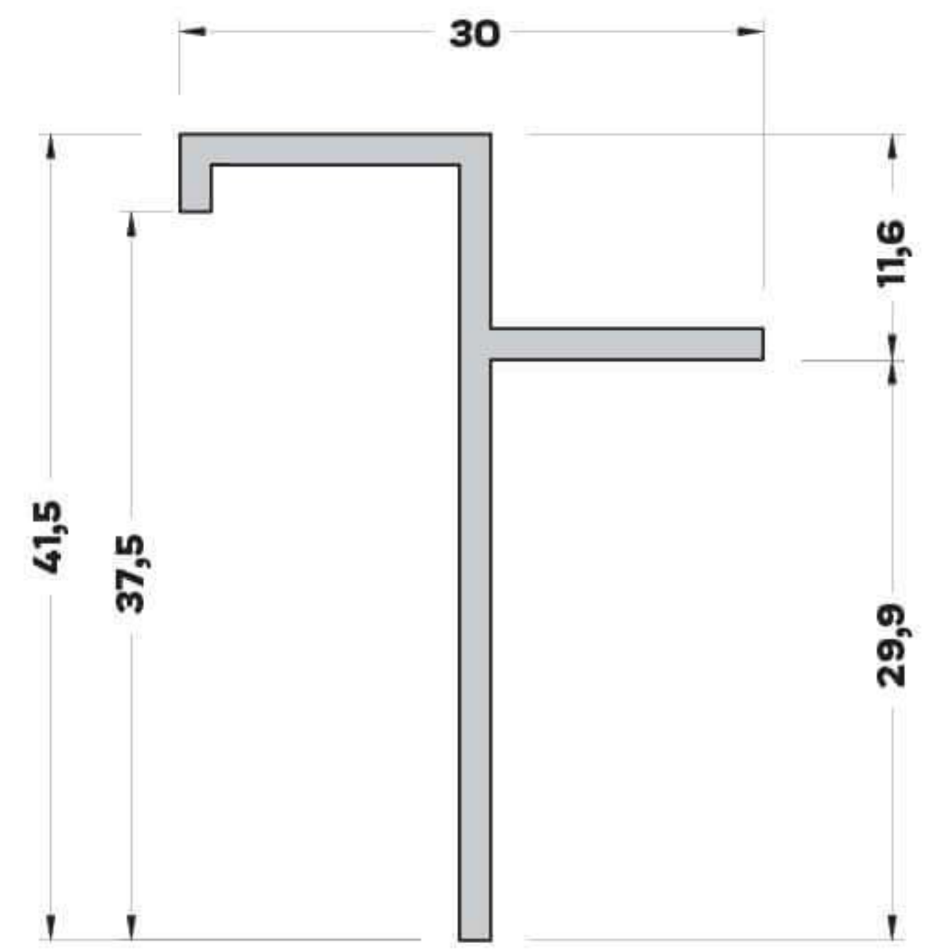
T-11484 (0,320 kg/mt) ASİMETRİK T BİNİ PROFİLİ
