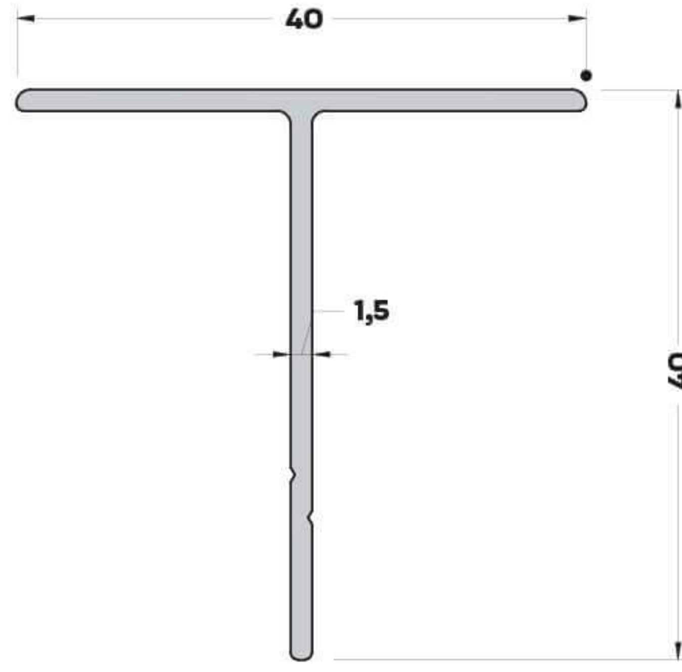
T-4690 (0,320 kg/mt.) T BİNİ PROFİLİ
