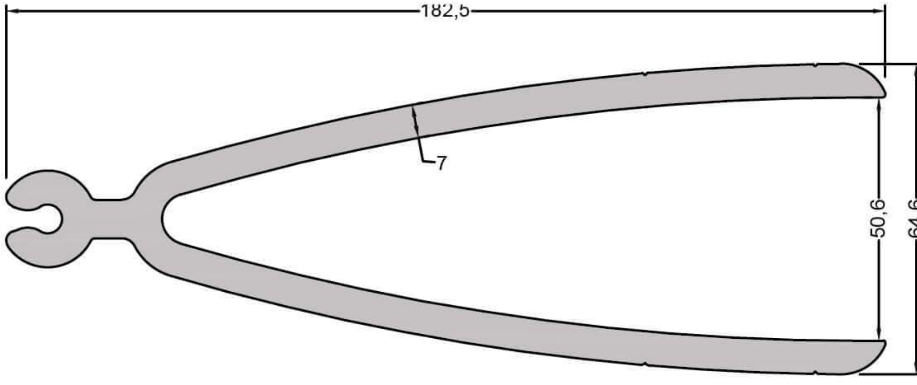
S-4005 ( 6,840 kg/mt ) GÜNEŞ KIRICI TAŞIYICI AYAK PR.
