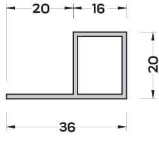
SN-3277 (0,309 kg/mt) SİNEKLİK KASA PROFİLİ
