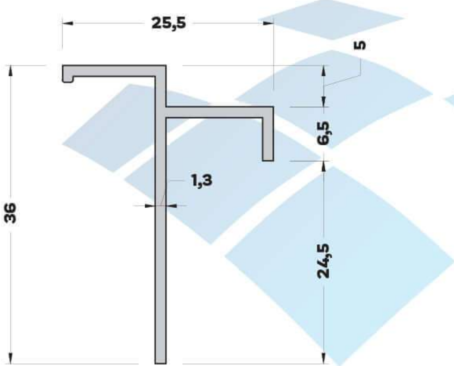
T-1121 (0,232 kg/mt.) ASİMETRİK T BİNİ PROFİLİ
