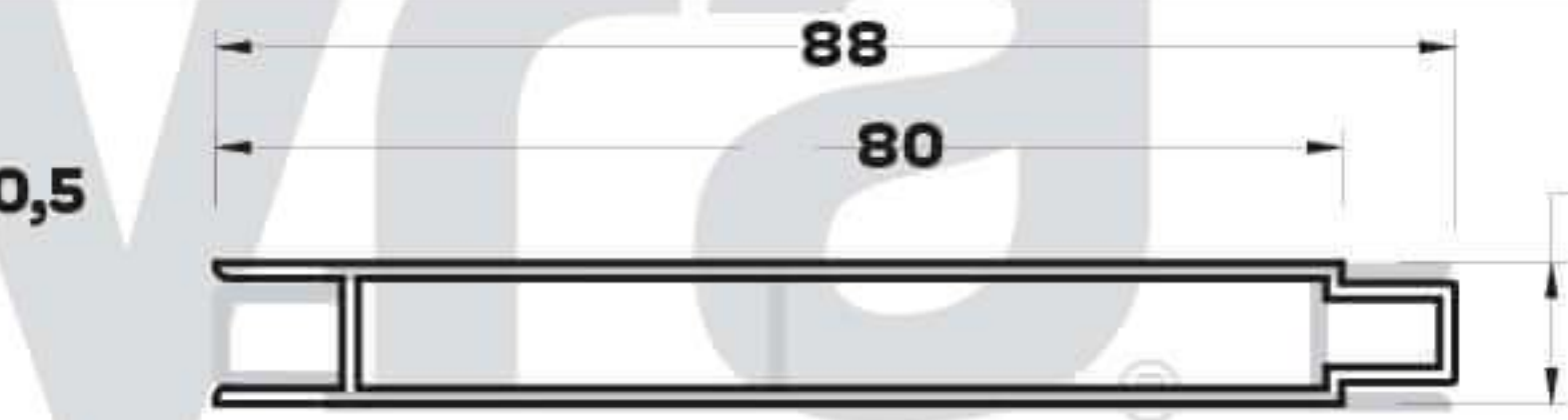
L-4647 (0,647kg/mt) LAMBRI PROFİLİ
