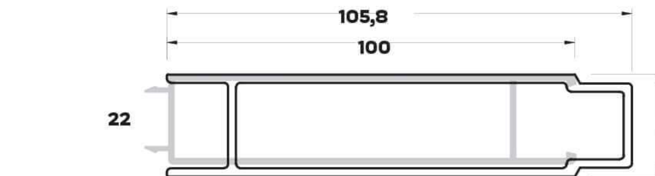
L-1249 (0,689 kg/mt) LAMBRI PROFİLİ
