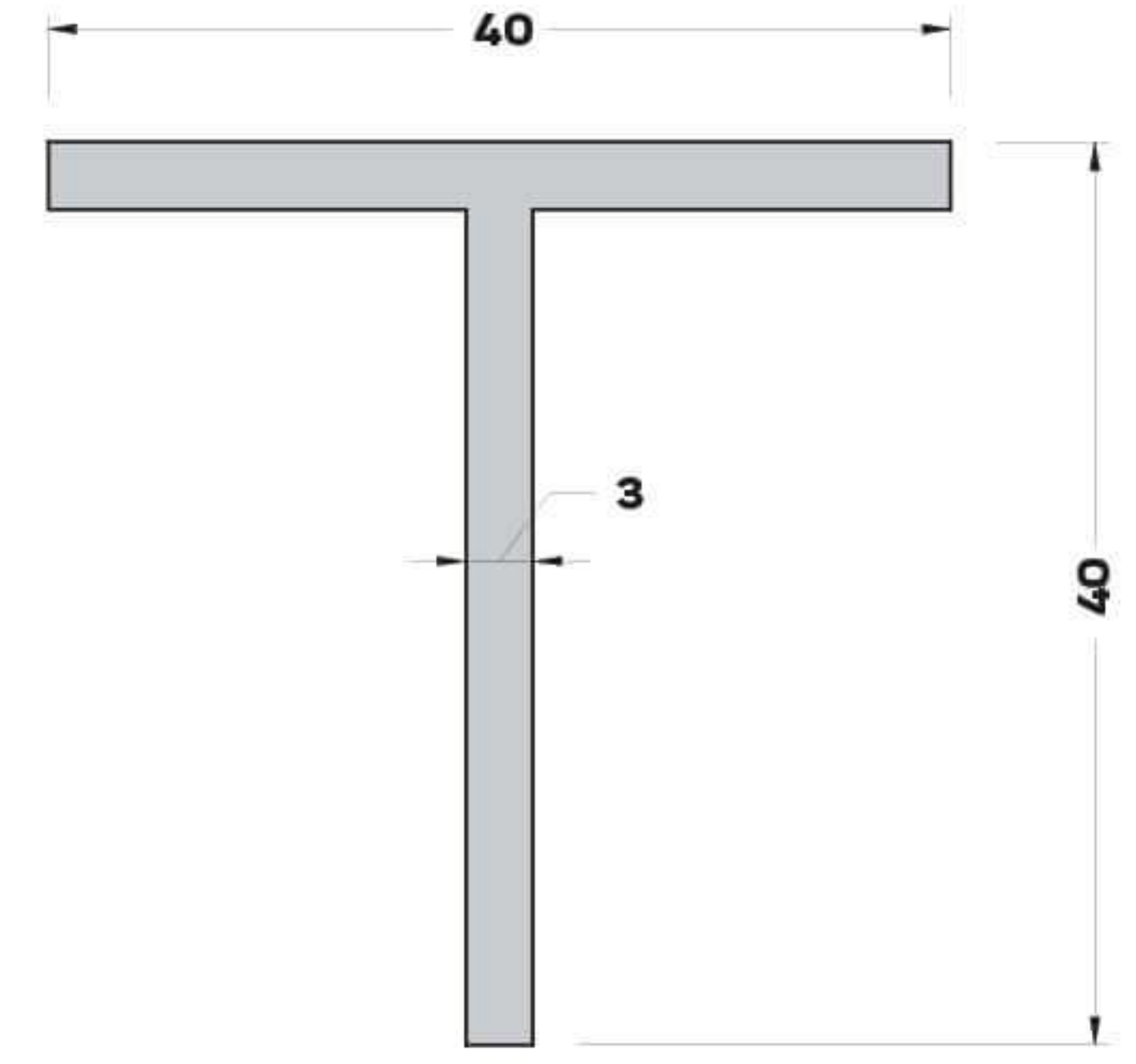
T-8276 (0,626 kg/mt.) T BİNİ PROFİLİ
