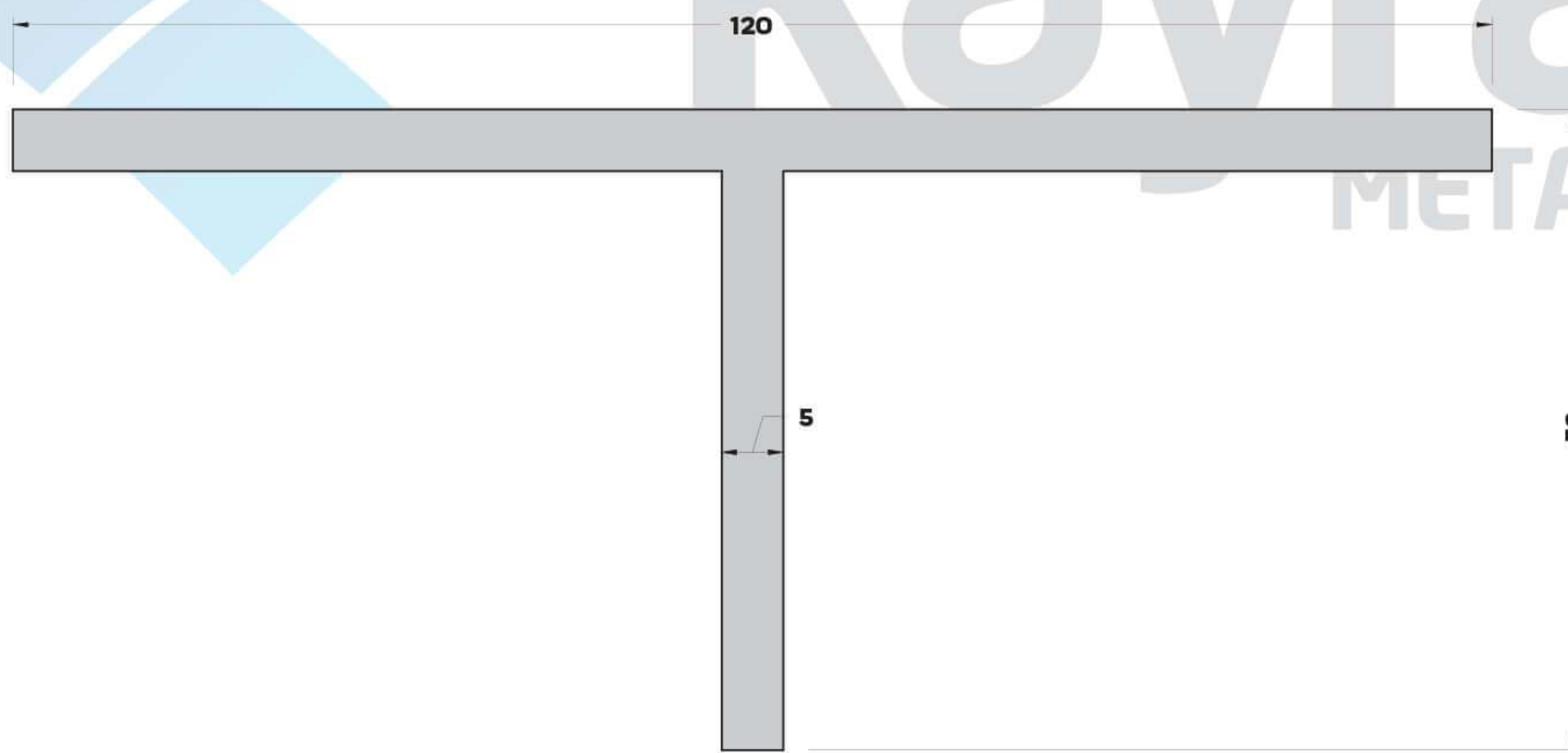
T-7206 (0,853 kg/mt) T BİNİ PROFİLİ
