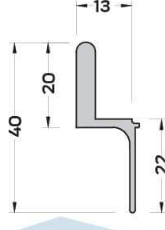
SN-4107 (0,282 kg/mt) SİNEKLİK PROFİLİ
