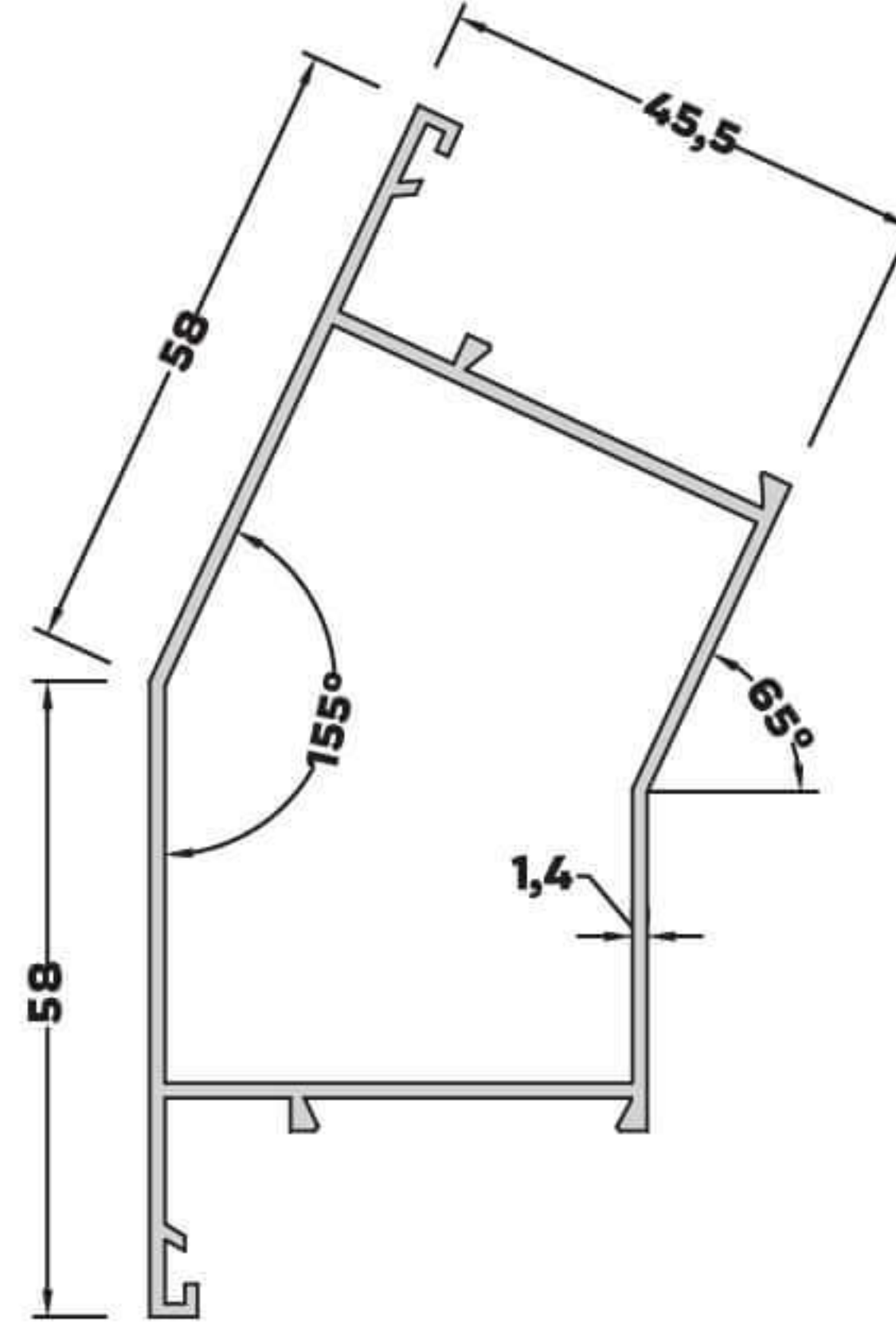
AL-2636 (1,083 kg/mt) 155° KÖŞE DÖNÜŞ PROFİLİ
