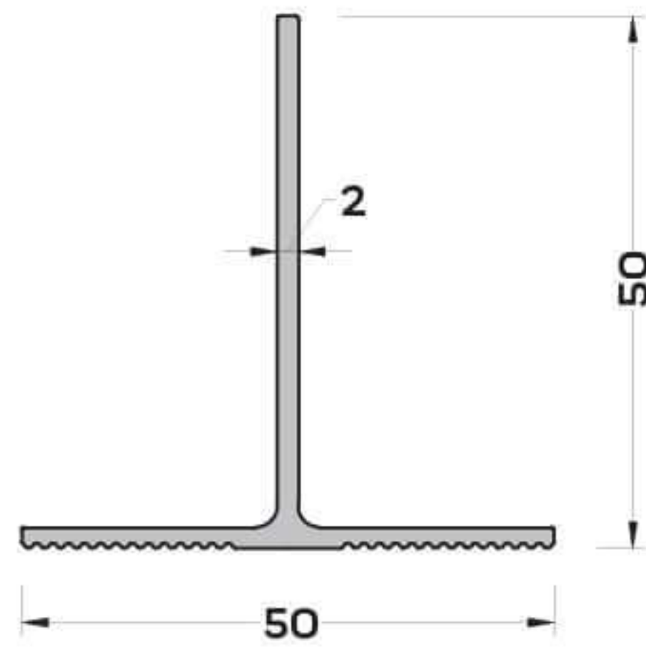
CK-6755 (0,507 kg/mt) T PROFİLİ
