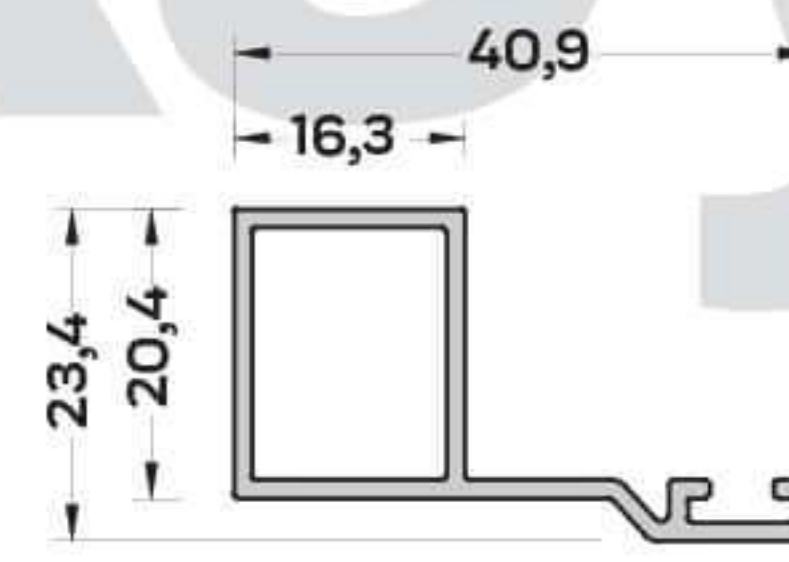
SN-2285 (0,370 kg/mt) SİNEKLİK RAY PROFİLİ
