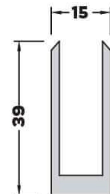
AL-1213 (0,540 kg/mt) DAR U BAĞLANTI PROFİLİ
