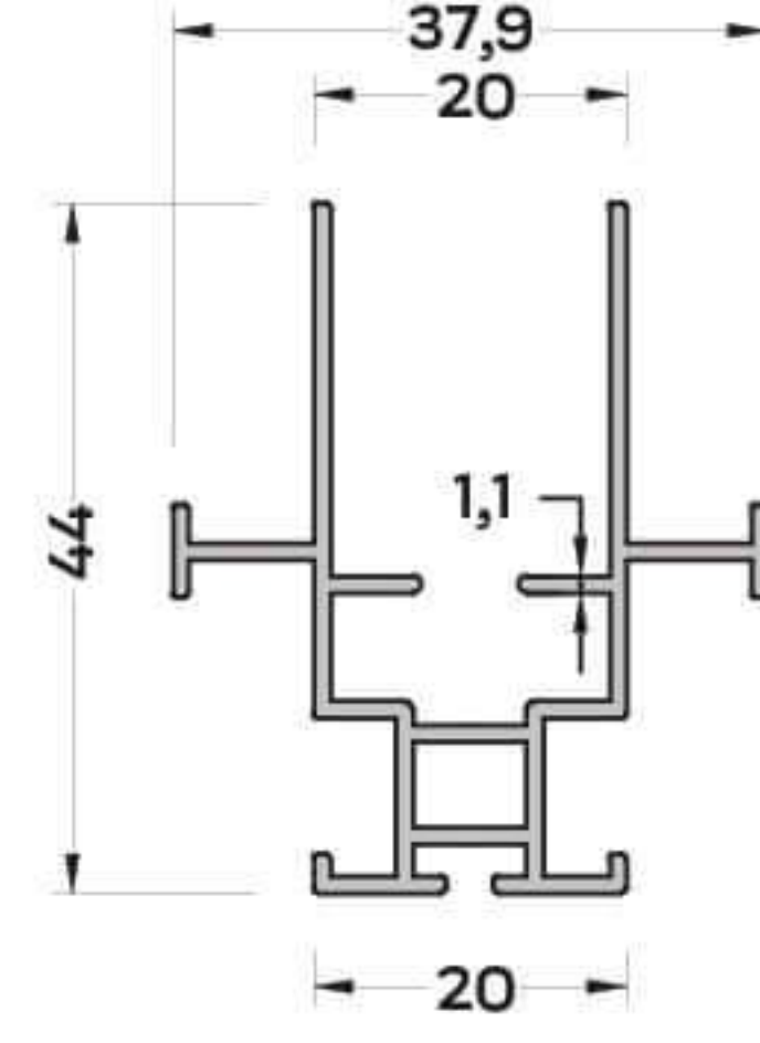
SN-4332 (0,516 kg/mt) SİNEKLİK KANAT PROFİLİ
