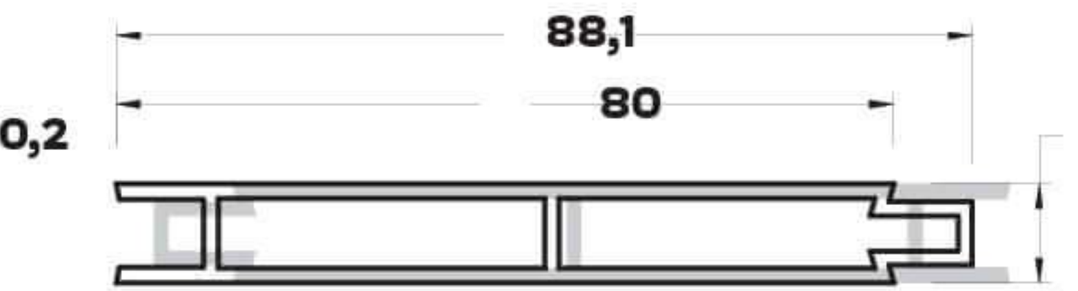
L-115 (0,609 kg/mt) LAMBRI PROFİLİ
