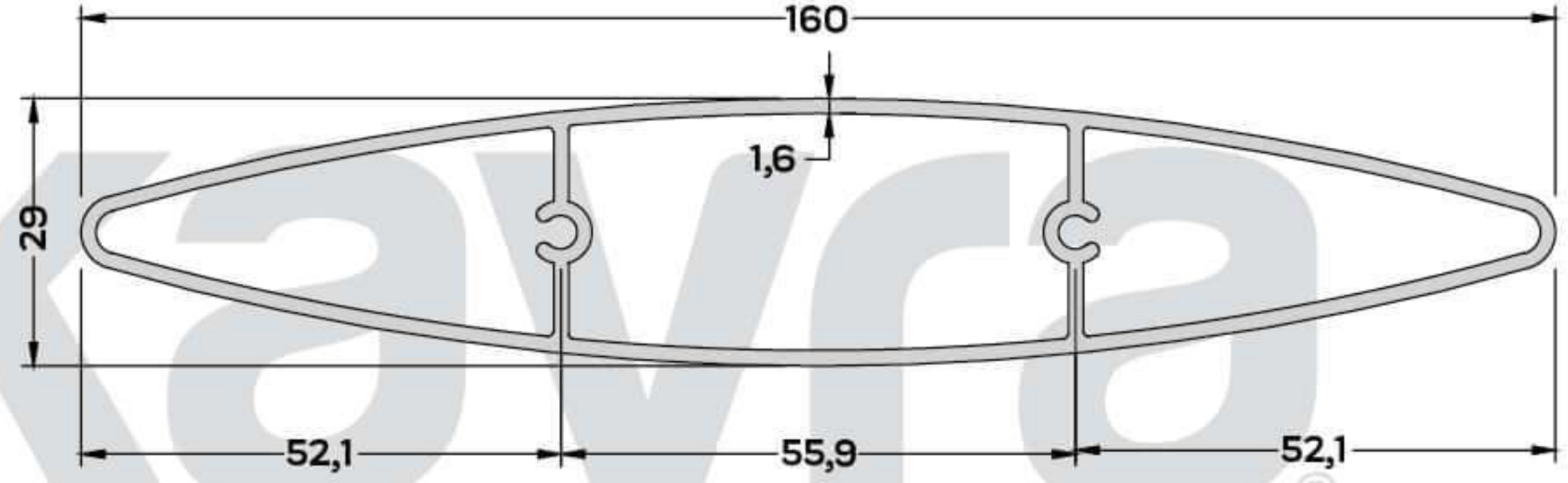
S-6074 (1,675 kg/mt) GÜNEŞ KIRICI PR. 160 mm
