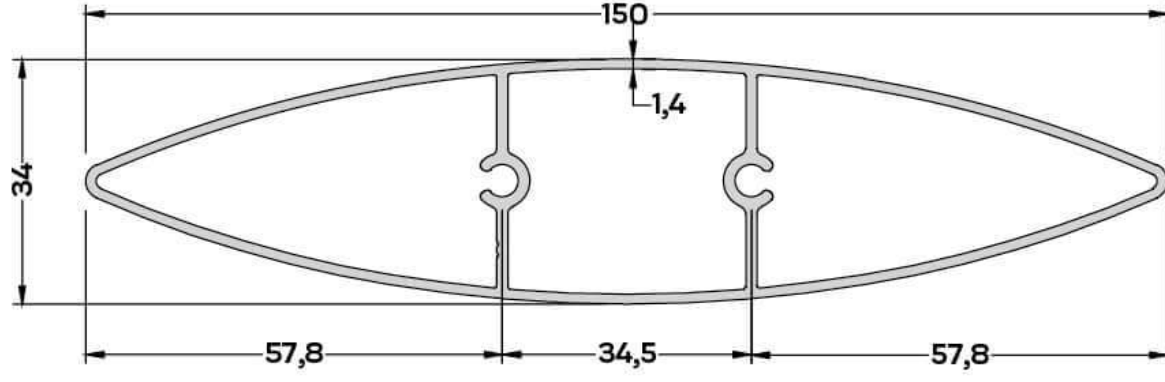
S-8288 (1,486 kg/mt) GÜNEŞ KIRICI PR. 150 mm
