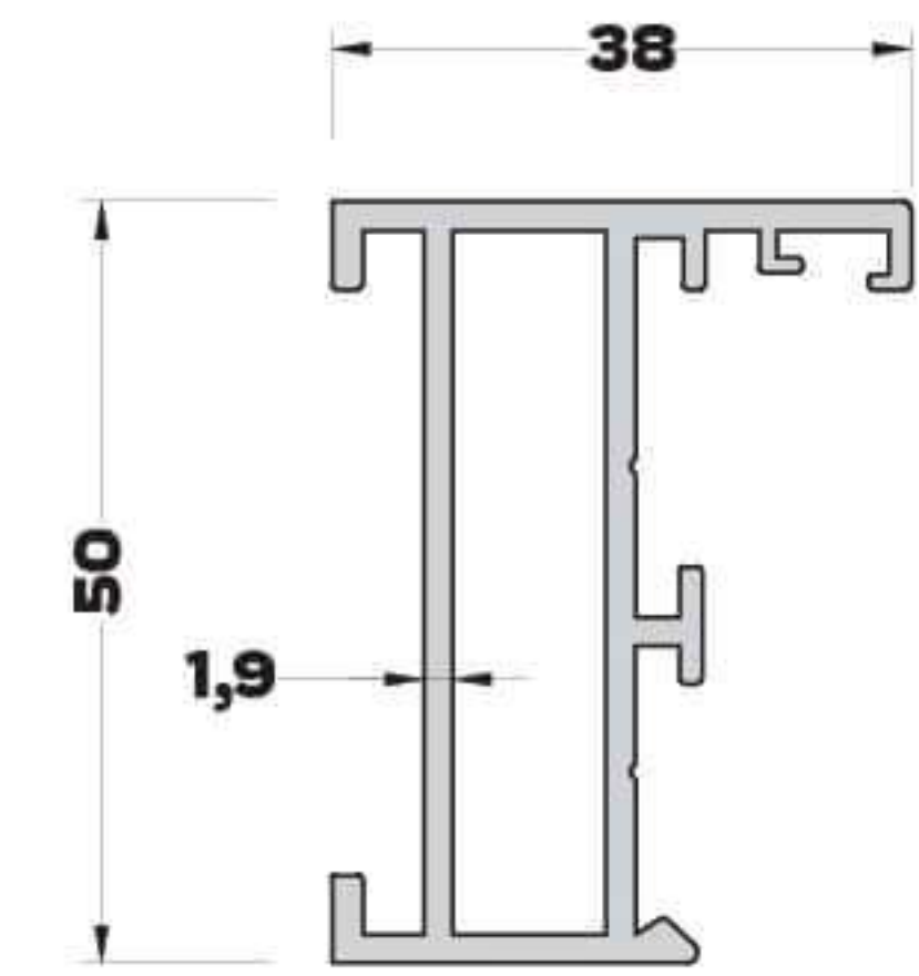
AB-3615 (1,189 kg/mt) TAŞIYICI GÖVDE PROFİLİ
