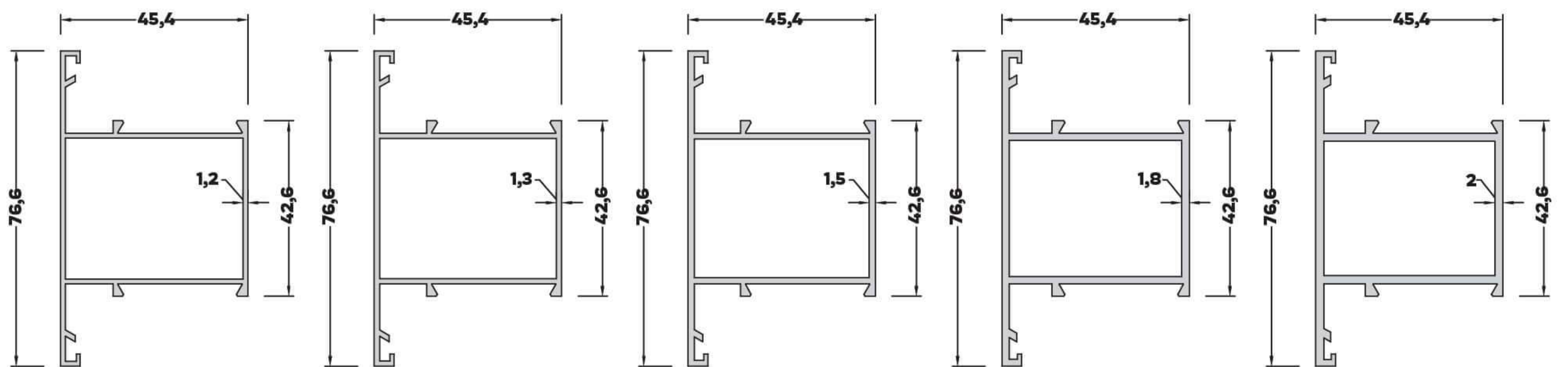
AL-3078 (0,658 kg/mt) DAR ORTA KAYIT PROFİLİ
