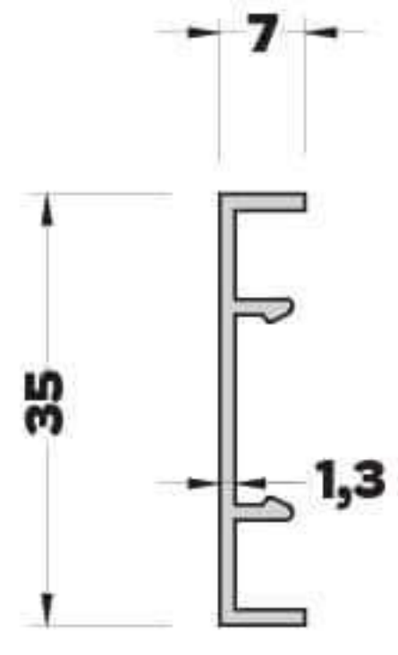
AB-1844 (0,197 kg/mt) KAPAK PROFİLİ
