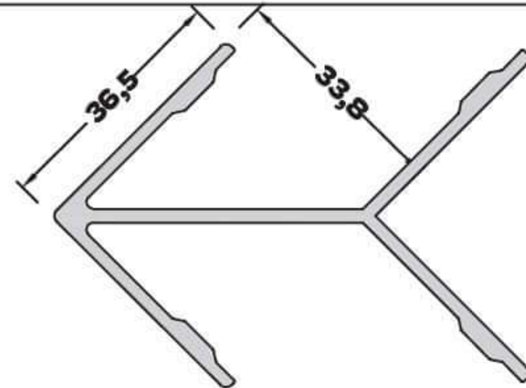
AL-3066 (1,162 kg/mt) GENİŞ KÖŞE ÇAVUŞ PROFİLİ
