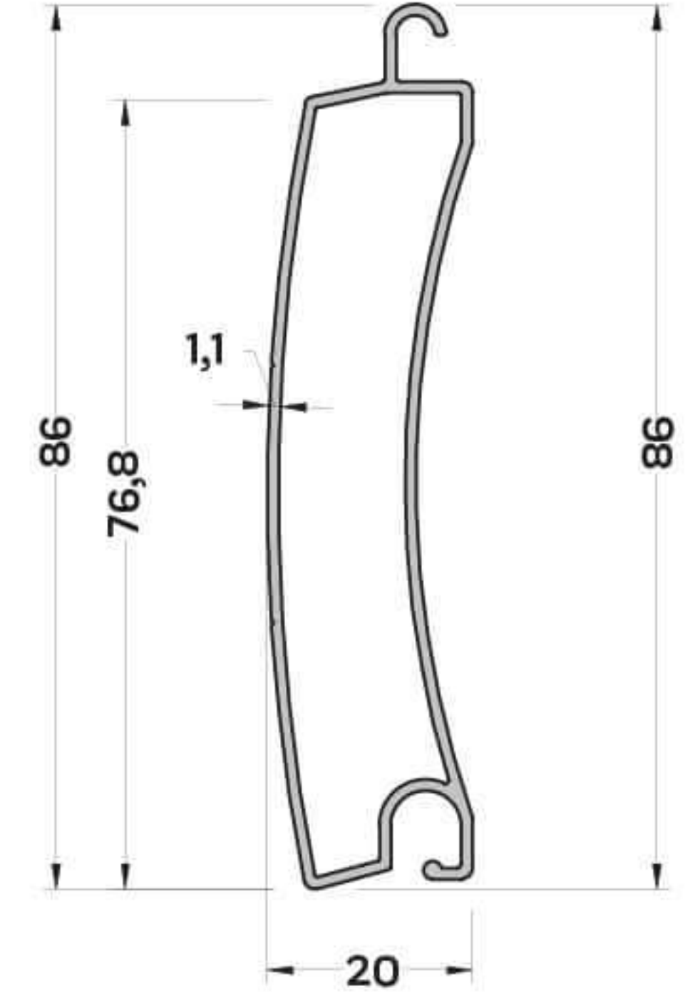
P-3430 (0,615 kg/mt) PANJUR LAMEL PROFİLİ
