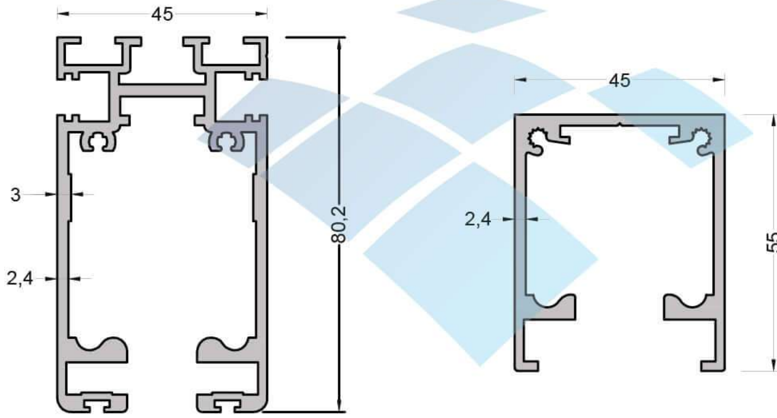
M-8905 ( 2,150 kg/mt ) ÜST RAY PROFİLİ
