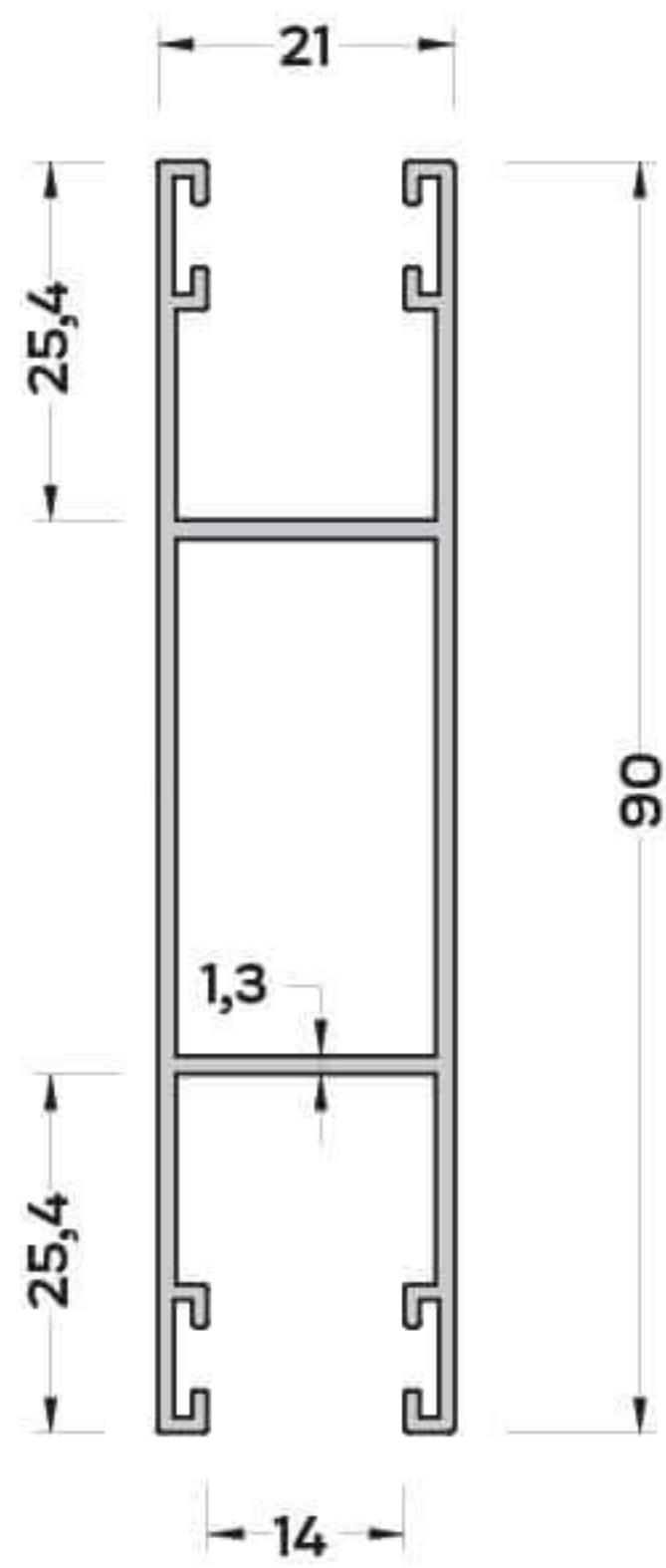
P-3419 (0,846 kg/mt) PANJUR ORTA KASA PROFİLİ
