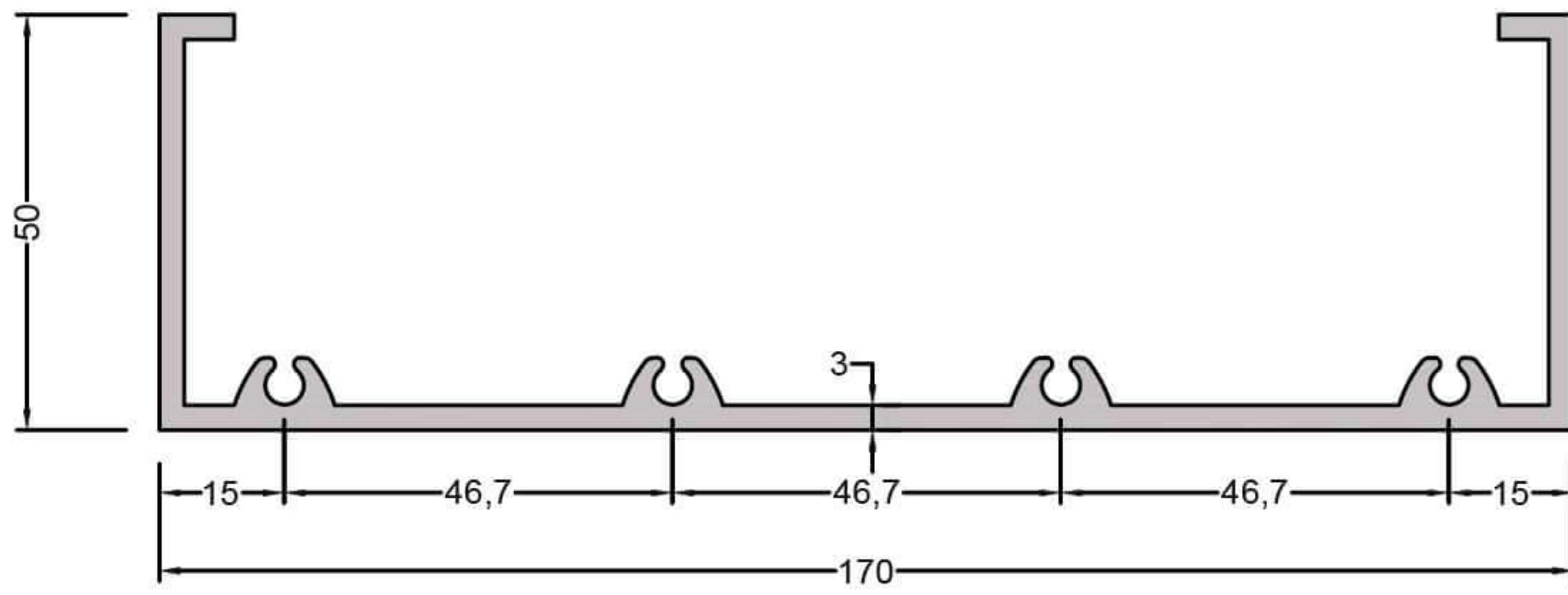
S-3294 ( 2,620 kg/mt ) GÜNEŞ KIRICI TAŞIYICI KUTU PR.
