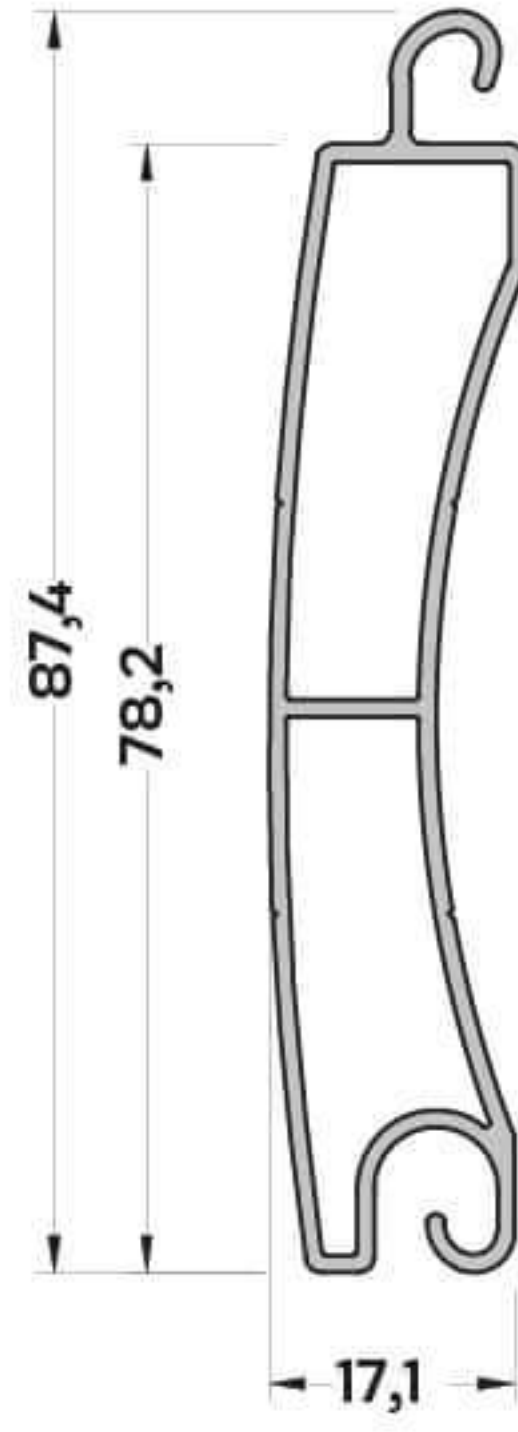
P-3946 (0,420 kg/mt) PANJUR LAMEL PROFİLİ
