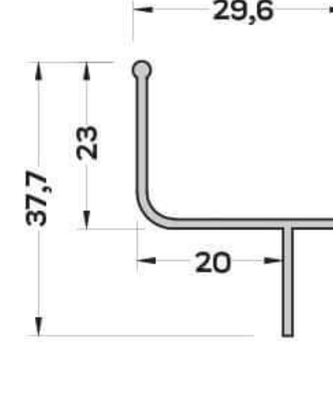
SN-1490 (0,227 kg/mt) SİNEKLİK PROFİLİ
