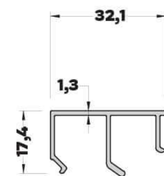
AB-11272 (0,560 kg/mt) ARA BÖLME BAĞLANTI PROFİLİ
