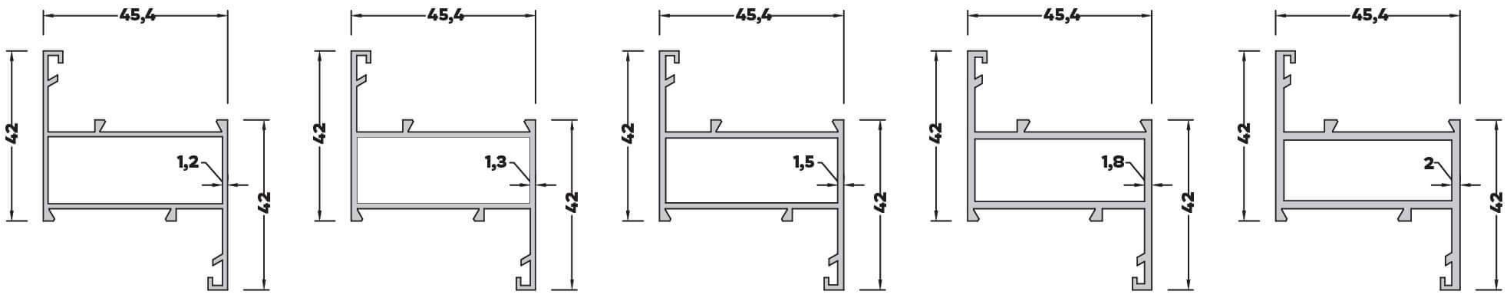
AL-3079 (0,653 kg/mt) DAR KANAT PROFİLİ AL-222 (0,693 kg/mt) DAR KANAT PROFİLİ AL-247 (0,780 kg/mt) DAR KANAT PROFİLİ AL-282 (0,916 kg/mt) DAR KANAT PROFİLİ AL-210 (0,997 kg/mt) DAR KANAT PROFİLİ
