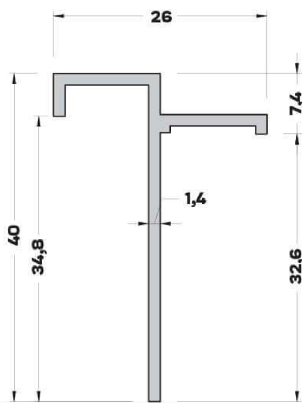
T-1555 (0,270 kg/mt.) ASİMETRİK T BİNİ PROFİLİ
