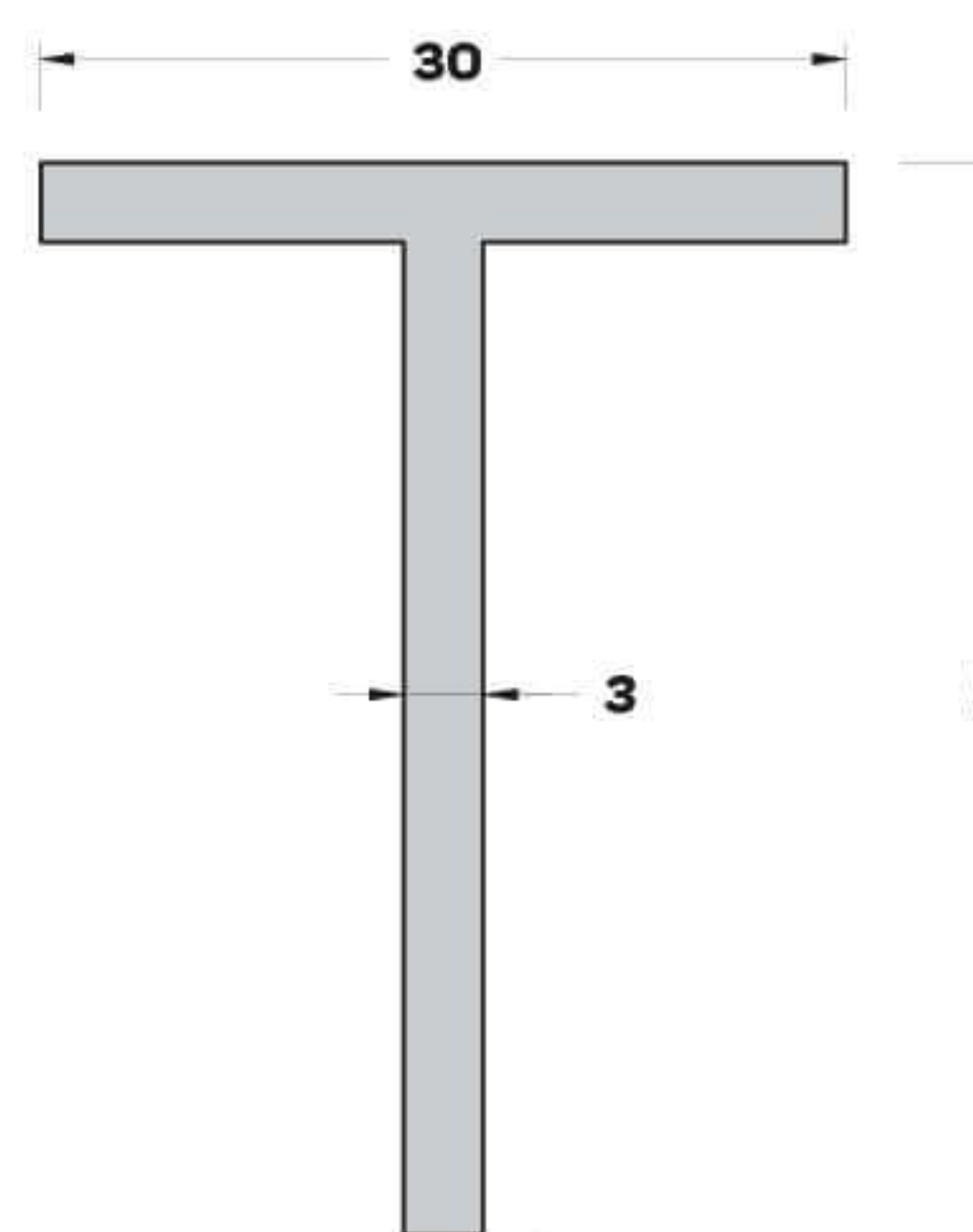
T-1756 (0,273 kg/mt) T BİNİ PROFİLİ
