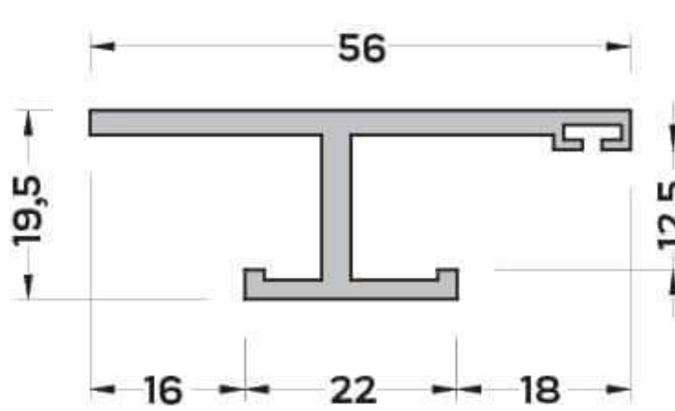
CK-6752 (0,632 kg/mt) YATAY TAŞIYICI KLİPS PR.
