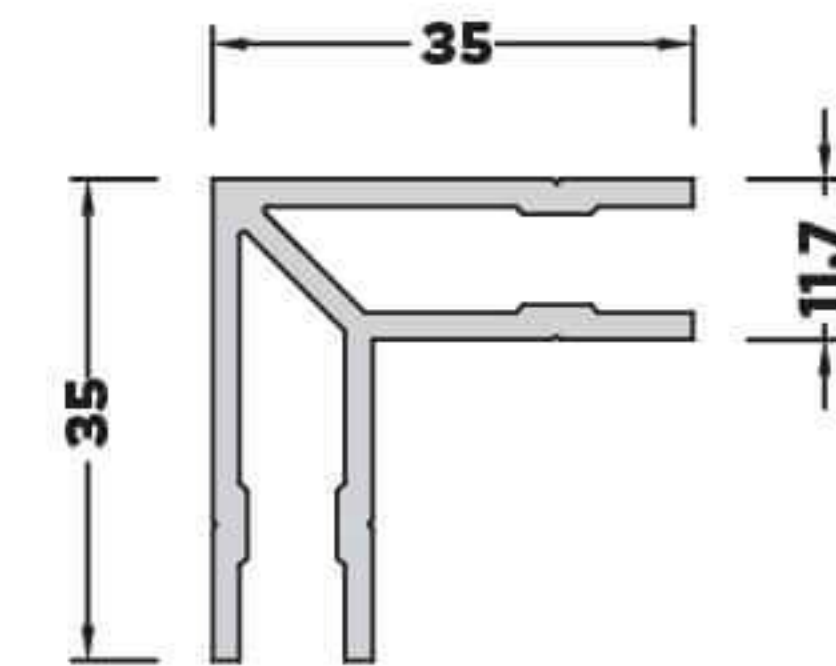
AL-1217 (0,722 kg/mt) DAR KÖŞE ÇAVUŞ PRO.
