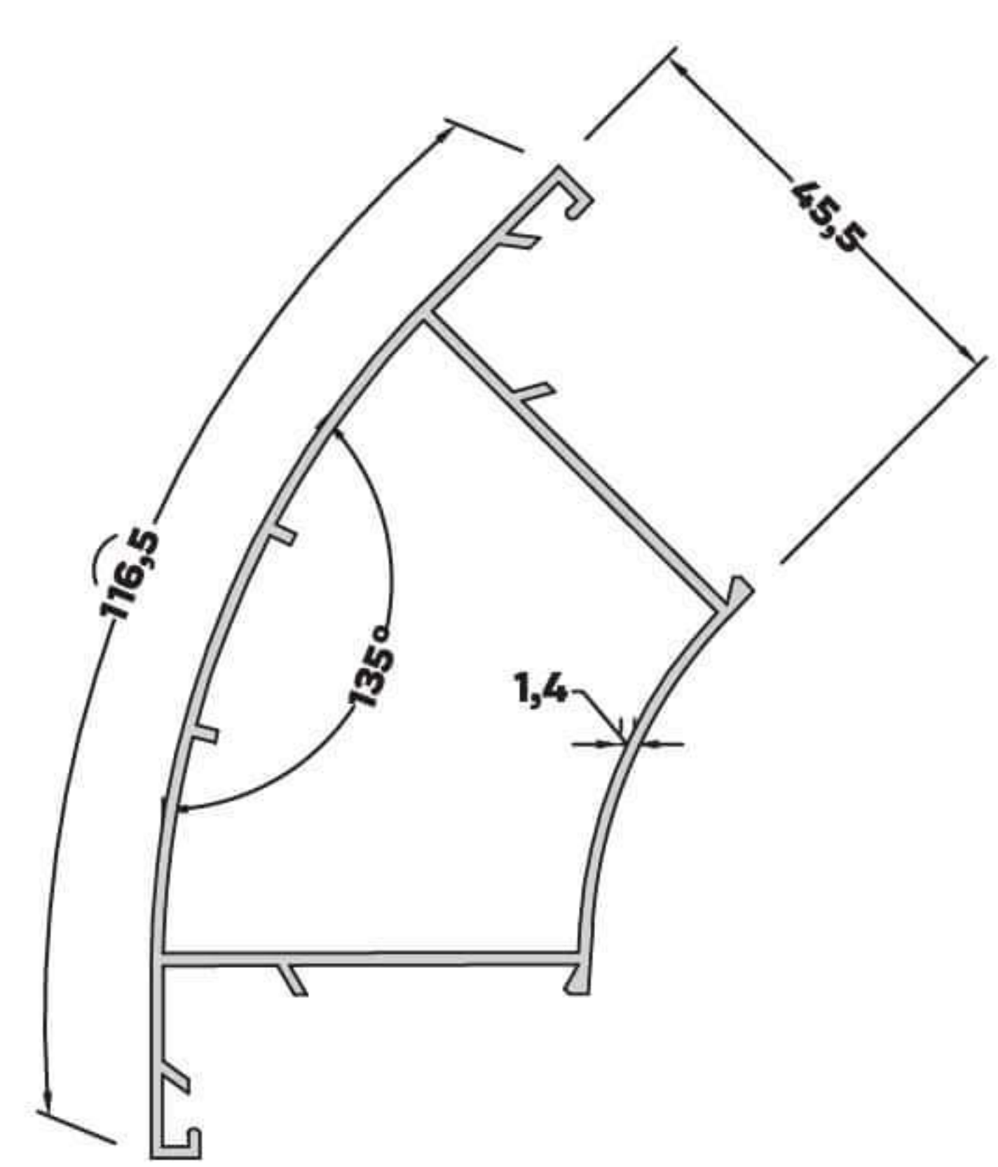
AL-3645 (0,985 kg/mt) 45° DÖNÜŞ PROFİLİ
