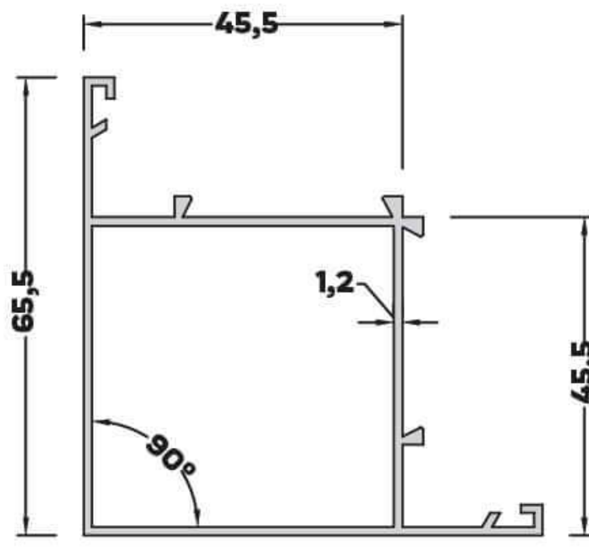
AL-3908 (1,582 kg/mt) 90° KÖŞE DÖNÜŞ PROFİLİ
