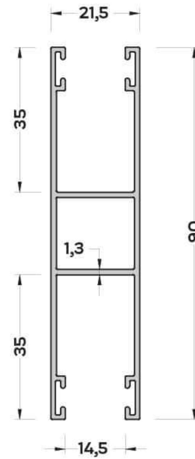
P-3420 (0,845 kg/mt) PANJUR ORTA KASA PROFİLİ
