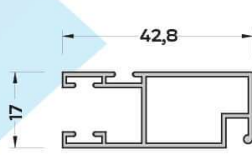
SN-1823 (0,380 kg/mt) SİNEKLİK RAY PROFİLİ
