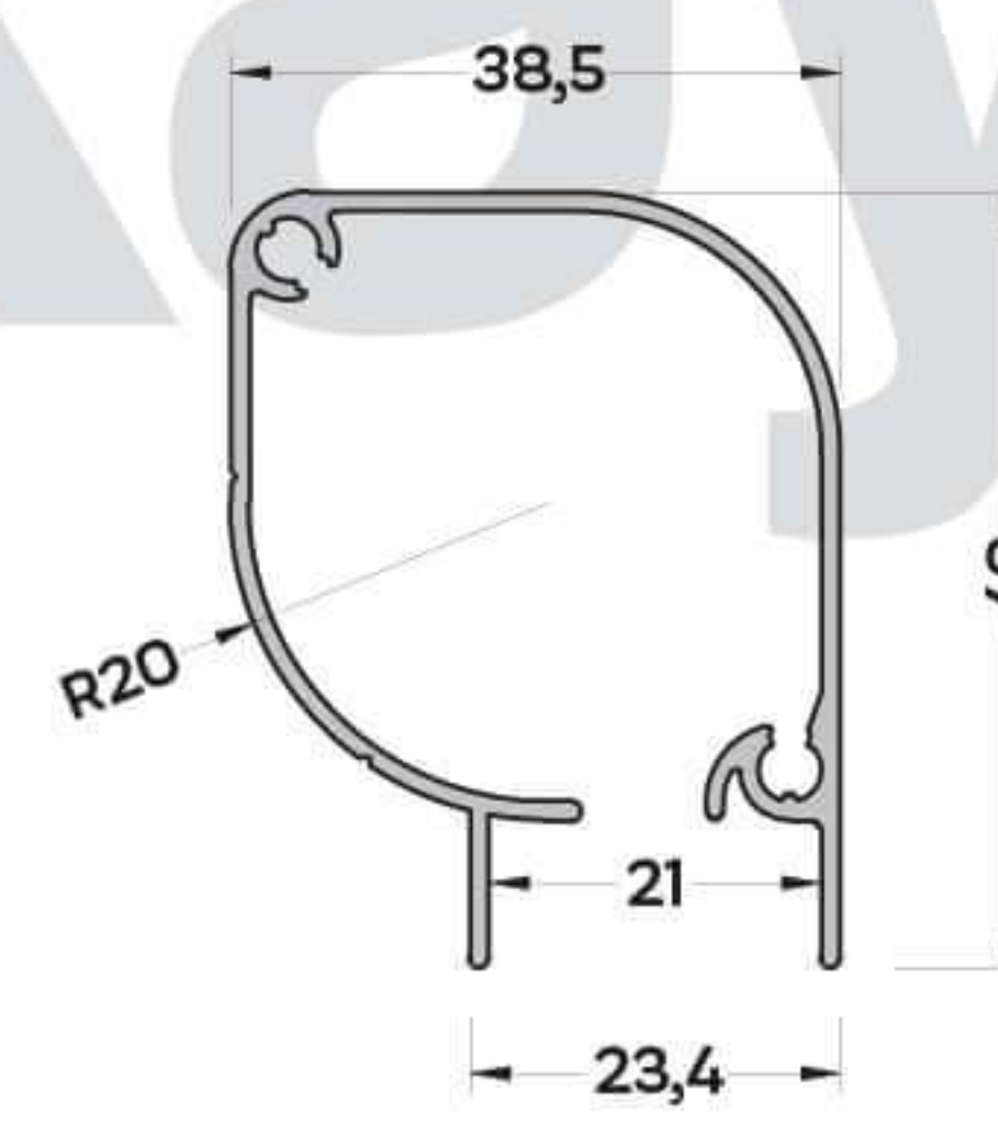
P-7625 (0,645 kg/mt) PANJUR LAMEL PROFİLİ
