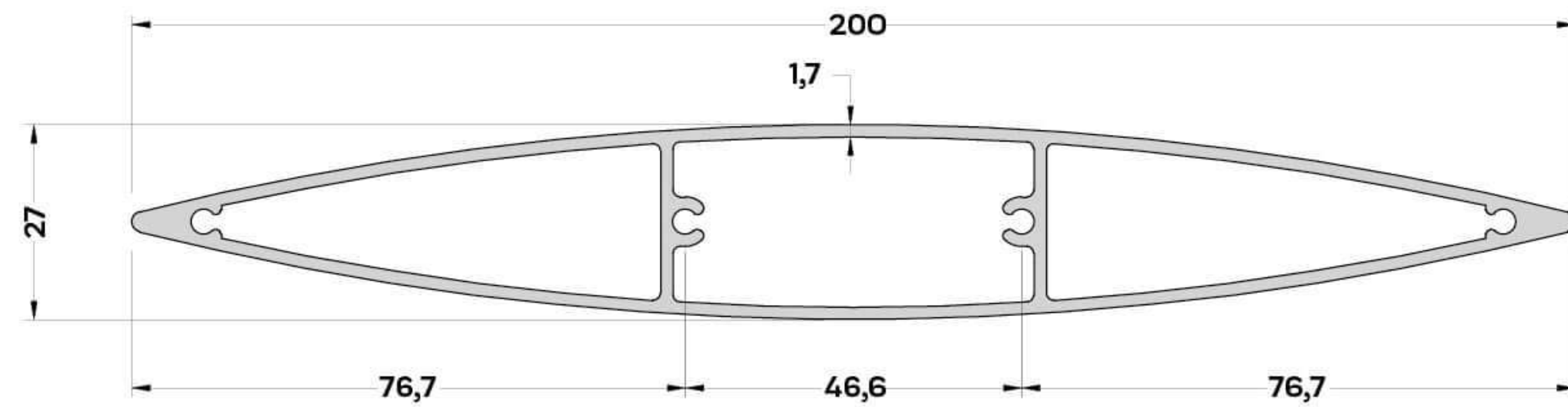
S-9439 (2,393 kg/mt) GÜNEŞ KIRICI PR. 200 mm
