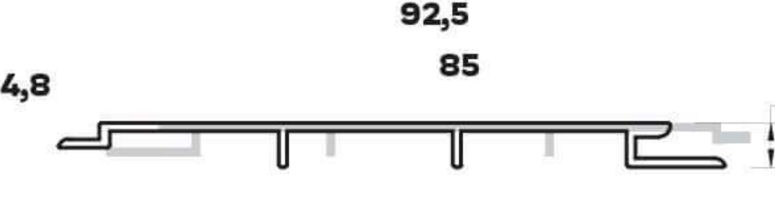
L-222 (0,378kg/mt) LAMBRI PROFİLİ
