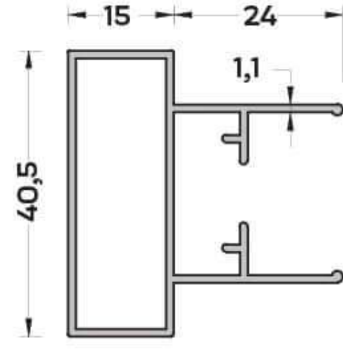
SN-4331 (0,520 kg/mt) SİNEKLİK DİKME PROFİLİ
