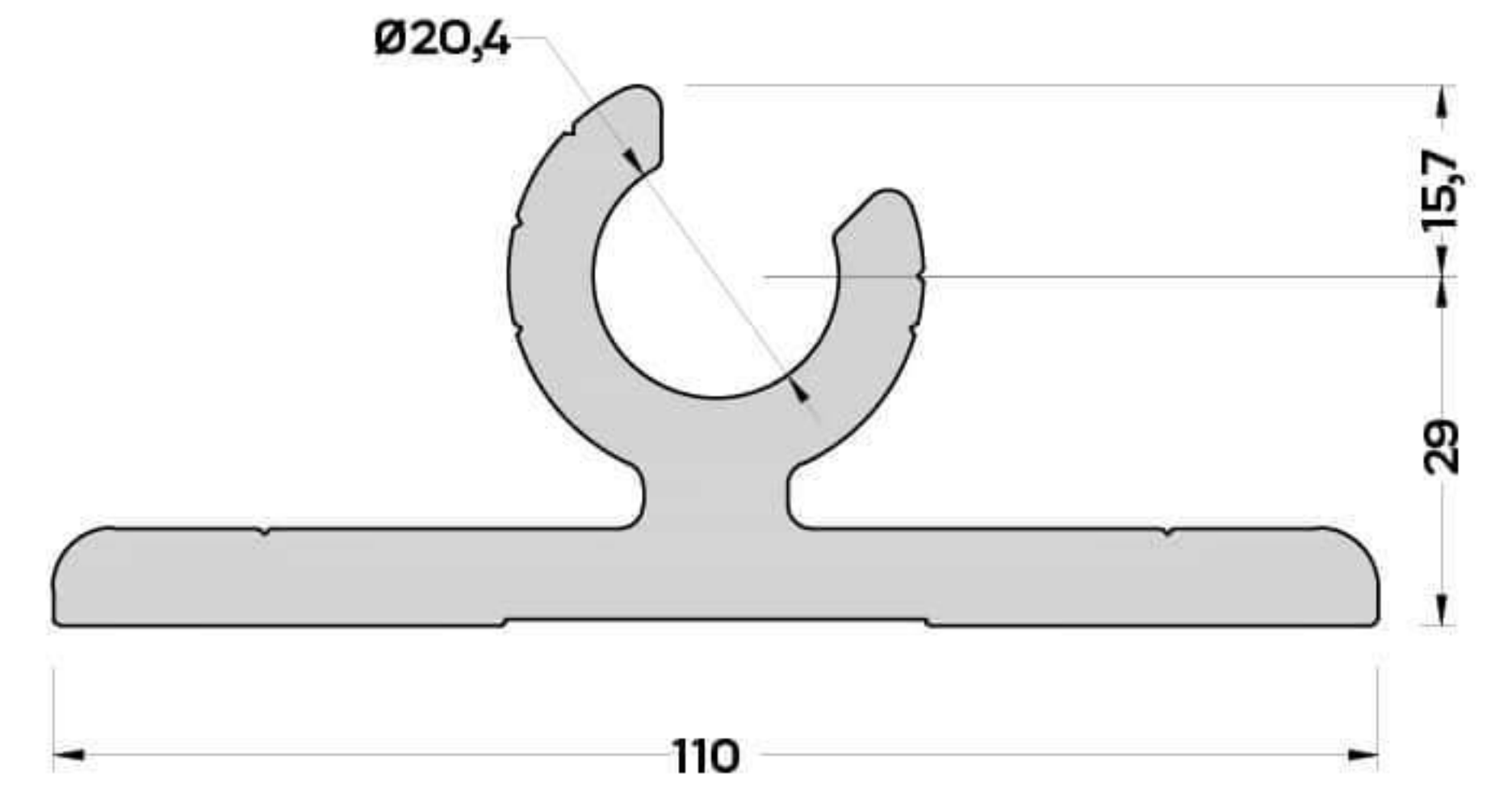
S-7523 (1,687 kg/mt) GÜNEŞ KIRICI AYAK PR.
