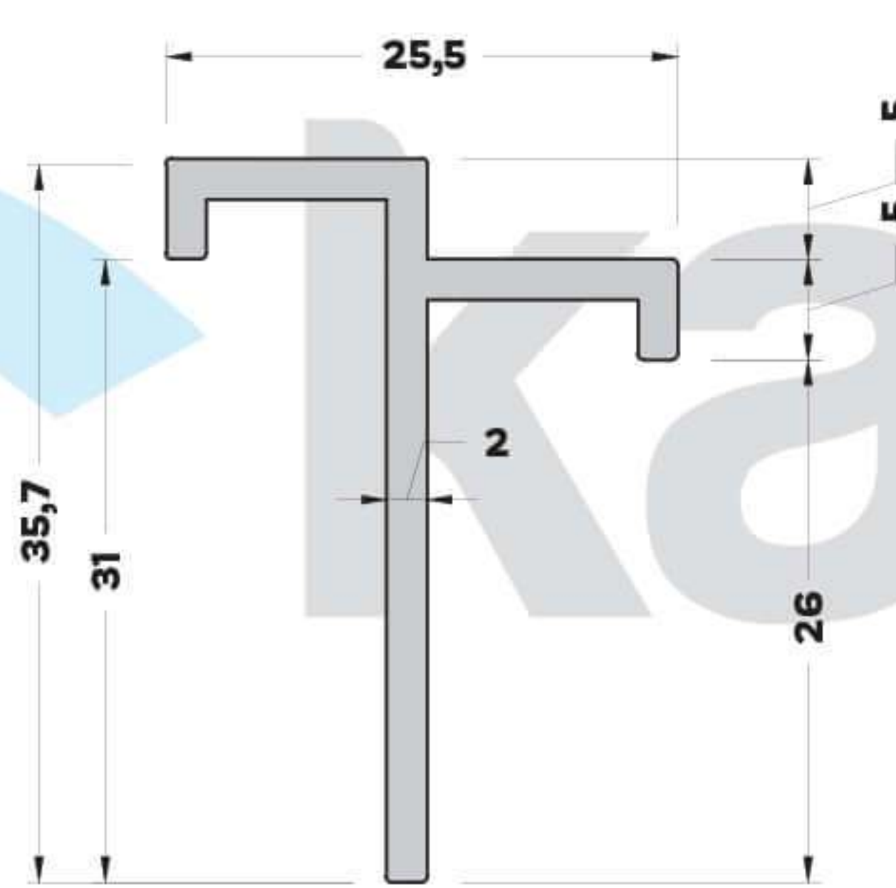
T-1123 (0,355 kg/mt.) ASİMETRİK T BİNİ PROFİLİ
