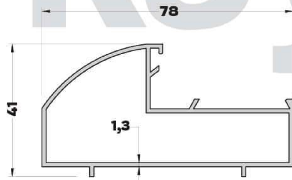
AB-6635 (0,203 kg/mt) KAPAK PROFİLİ
