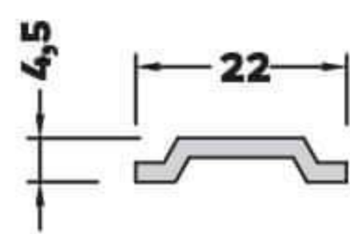
AL-3007 (0,217 kg/mt) ÇİFT CAM ÇITA PROFİLİ
