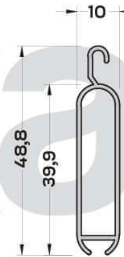
P-3420 (0,845 kg/mt) PANJUR ORTA KASA PROFİLİ
