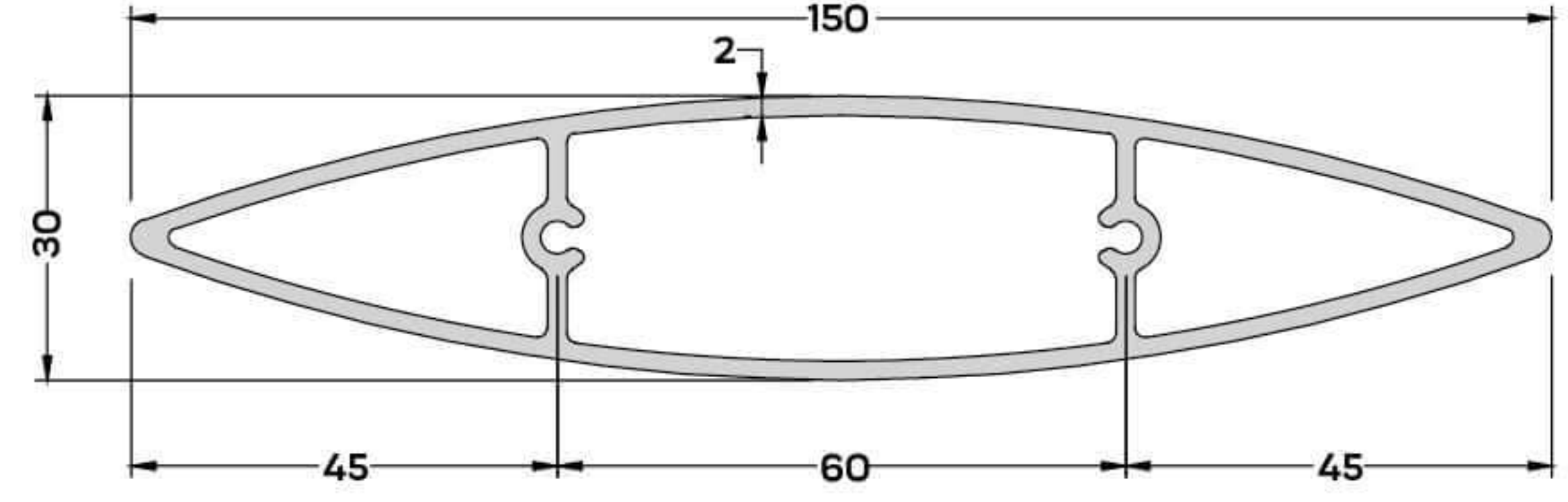
S-4835 (1,968 kg/mt) GÜNEŞ KIRICI PR. 150 mm
