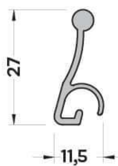
P-3442 (0,209 kg/mt) PANJUR ASKI PROFİLİ
