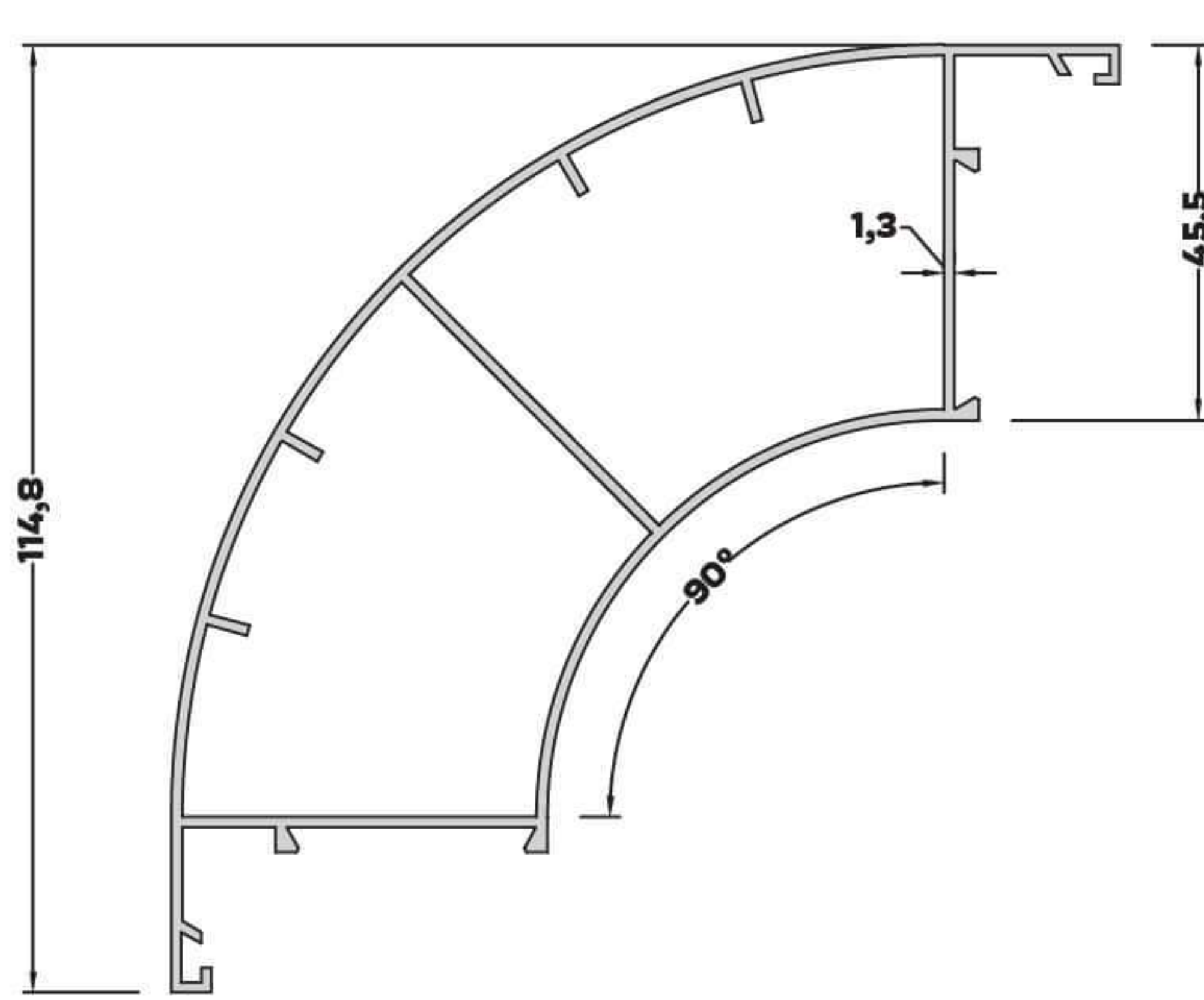
AL-3908 (1,582 kg/mt) 90° KÖŞE DÖNÜŞ PROFİLİ
