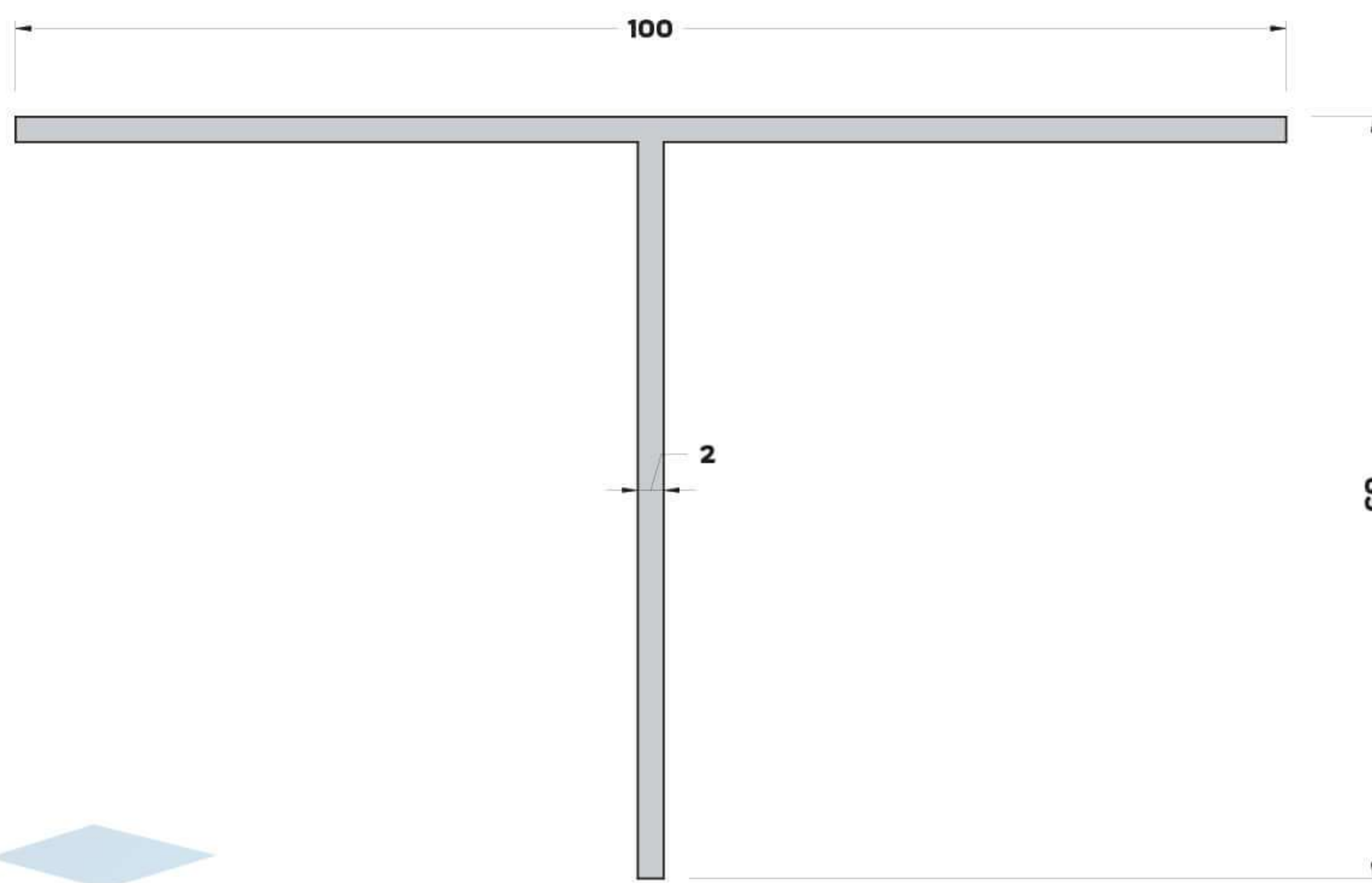
T-7206 (0,853 kg/mt) T BİNİ PROFİLİ
