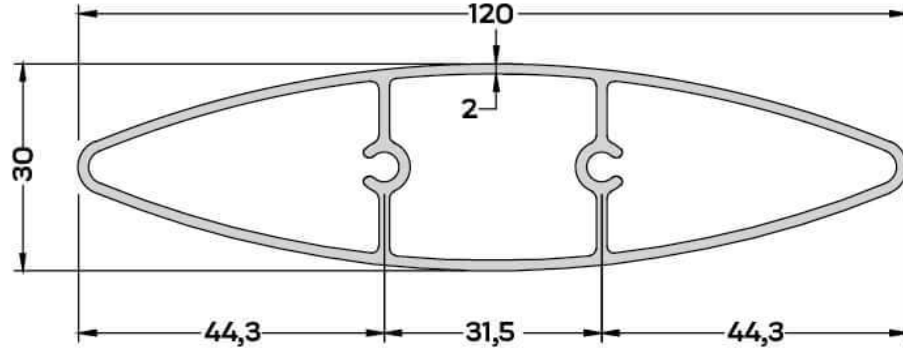
S-6336 (1,300 kg/mt) GÜNEŞ KIRICI PR. 120 mm
