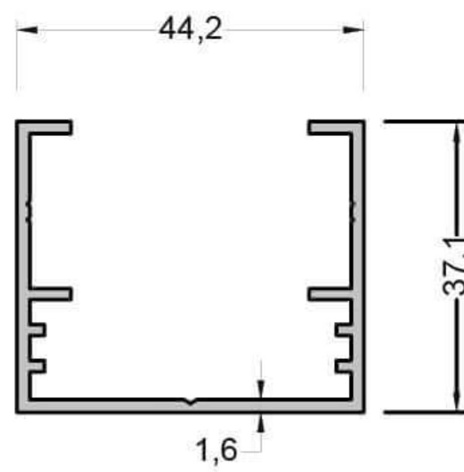
M-11096 ( 1,365 kg/mt ) ÜST RAY PROFİLİ
