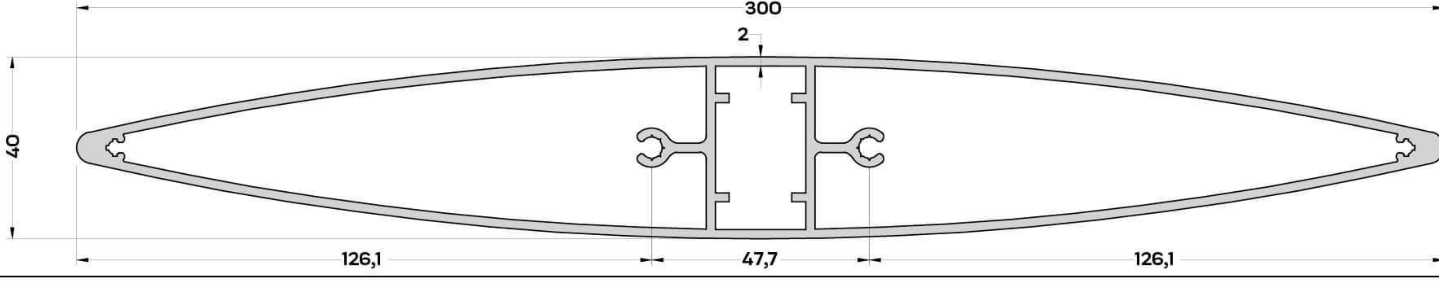
S-6780 (4,170 kg/mt) GÜNEŞ KIRICI PR. 300 mm
