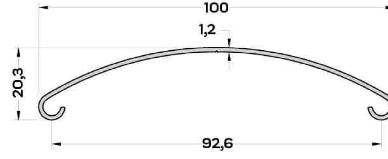
S-10067 (0,410 kg/mt) GÜNEŞ KIRICI PR.
