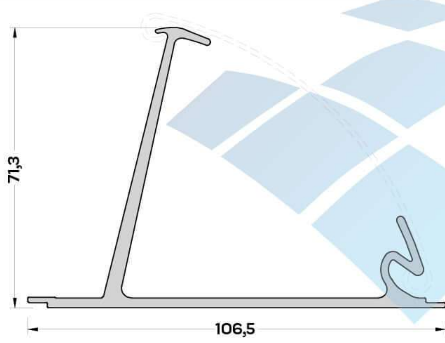
S-10068 (0,954 kg/mt) GÜNEŞ KIRICI PR.
